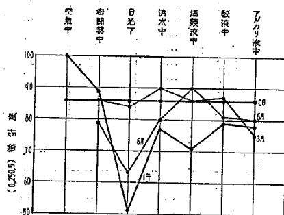
第 13 図 ストレート・アスファルト (150~200) 1.0°C 稠度変化 但し, (0mm, 250g, 5sec) の微針度
