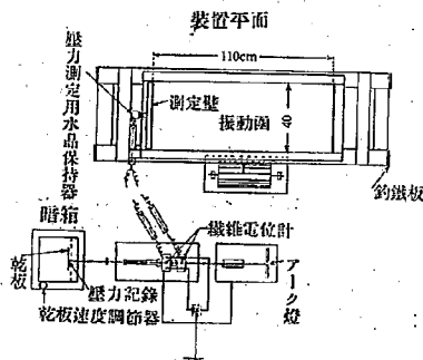
第 8 圖 振動試験装置
