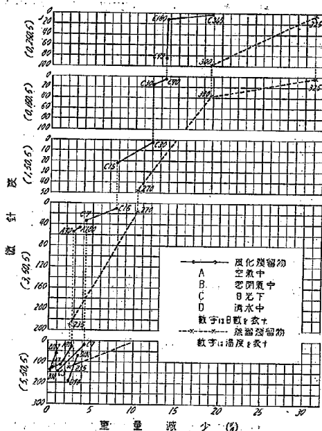
第 40 圖 タール (5) 蒸溜殘留物及風化殘留物 1.0°C 微針度と重量變化との比較
