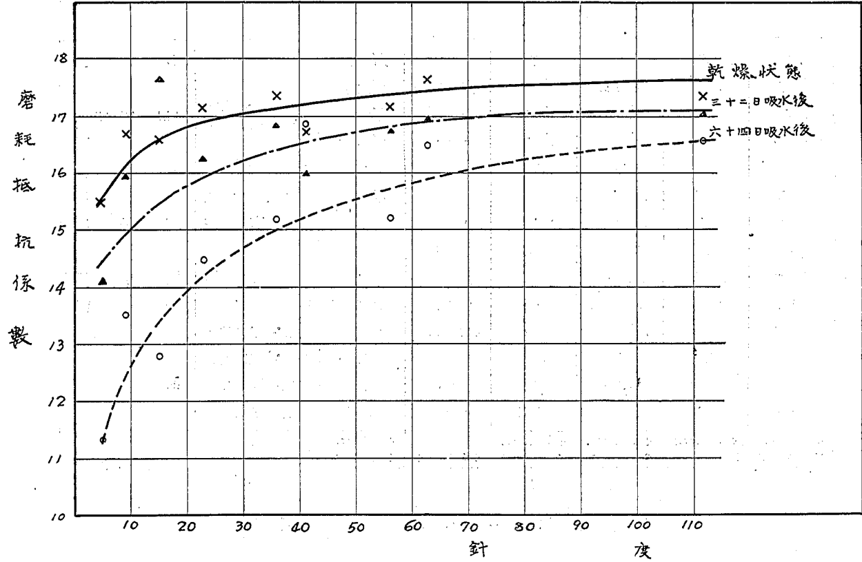
針度と磨耗抵抗係数の関係
