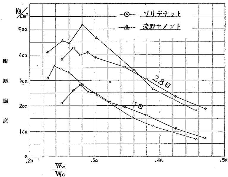
第八圖 水量と耐圧強度の關係
