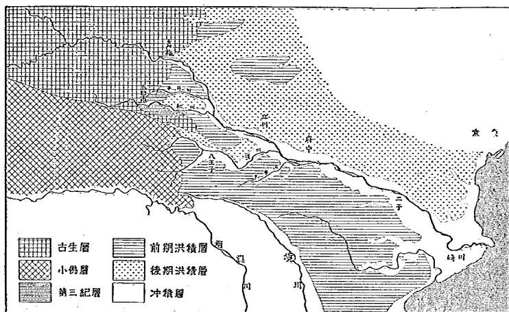
第十三圖 多摩川流域地質略圖
