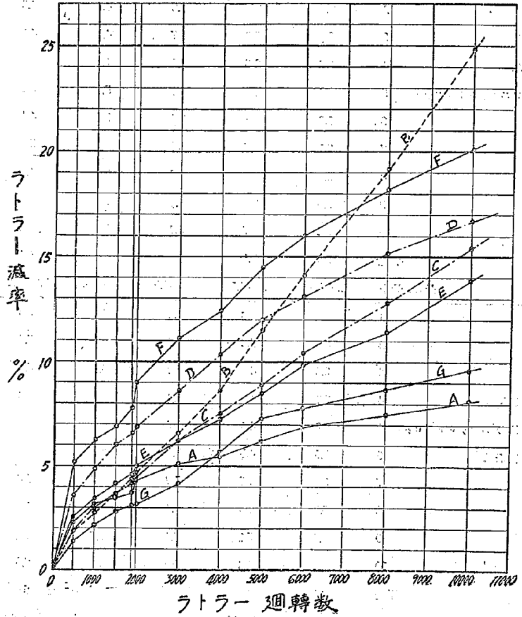
第一圖 ラトラー減率
