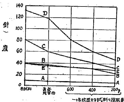
第四表 蒸發減試験 ( 163^{\circ}\text{C} , 50g, 5h) 及び一年放置後に於ける針度の比較
