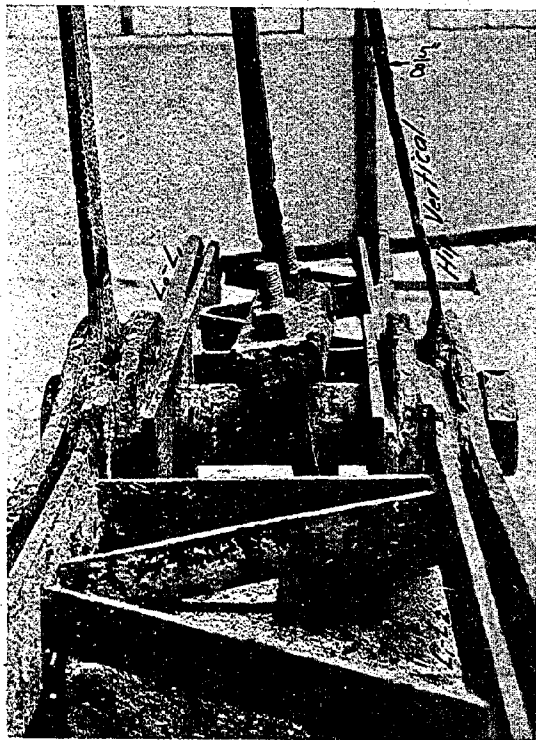
写真第一 舊橋側桁間第二下格點腐 蝕狀況(其一)
