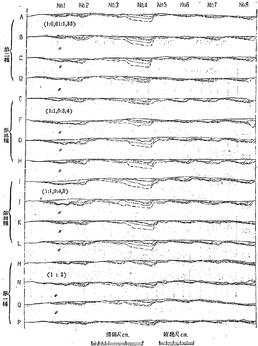
第 10 圖 甲種試験路面磨耗横断面圖
