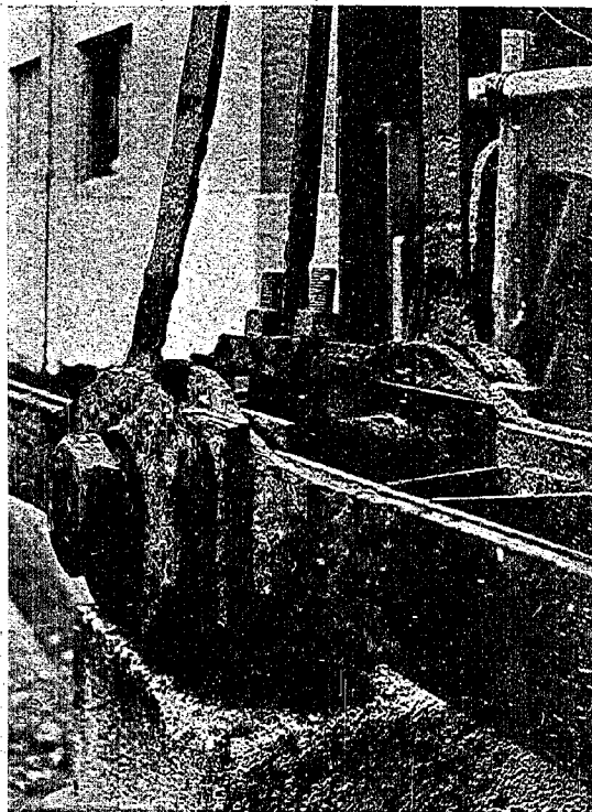
写真第二 舊橋側桁間第二下格點腐 蝕狀況(其二)
