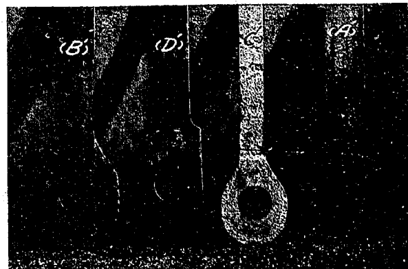
寫真第五 部材 A, B, C, D, 內側腐蝕狀態
