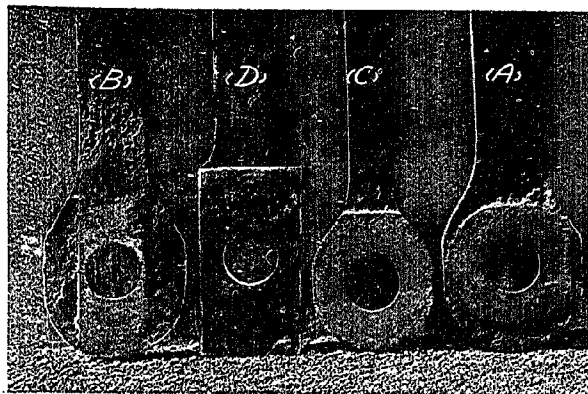
寫真第三 部材 A, B, C, D, 內側腐蝕狀態
