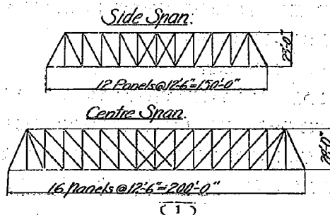
第一圖 舊橋結構略圖
