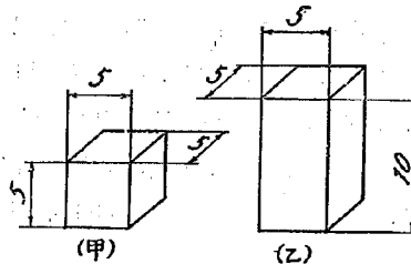
第一圖 抗壓試験片
