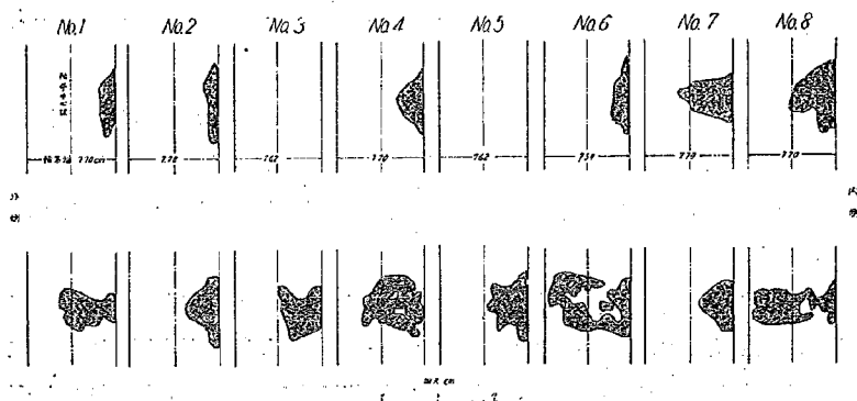
第9圖 鐵輪帶と混凝土路面との接觸面
