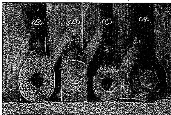
寫真第四 部材 A, B, C, D, 外側腐蝕狀態
