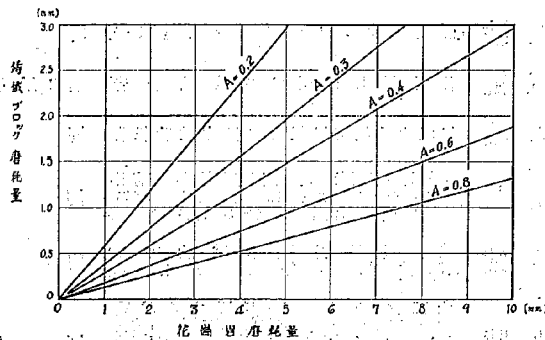
第三圖 鑄鐵ブロックに於ける突起部の面積と磨耗量との比較
