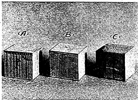
写真第一 抗 壓 試 験 (甲)
