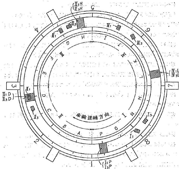
第 12 圖 甲種試驗路面磨耗狀況 (其一)
