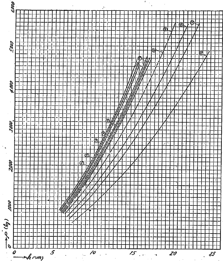
第16圖 混凝土舗装許容荷重と所要厚
