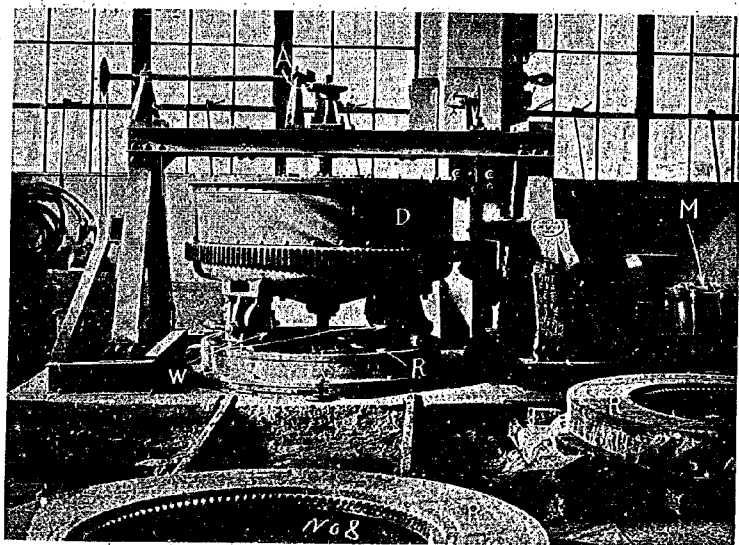
第 7 圖 乙種道路試驗機
