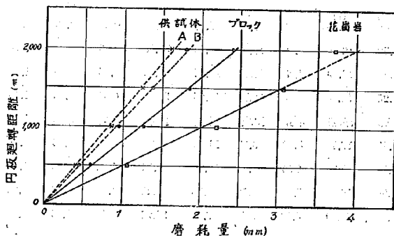
第二圖 磨耗量比較
