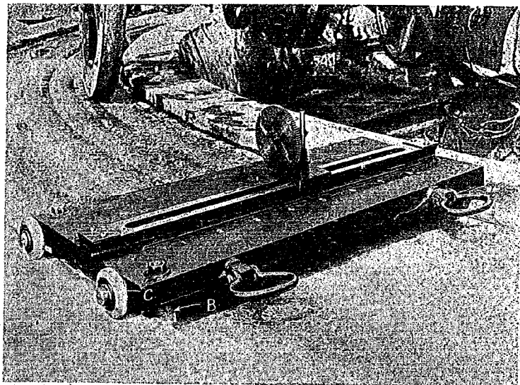
第 6 圖 凹 凸 計(甲種試驗用)
