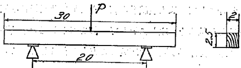
第三圖 彎曲試験片
