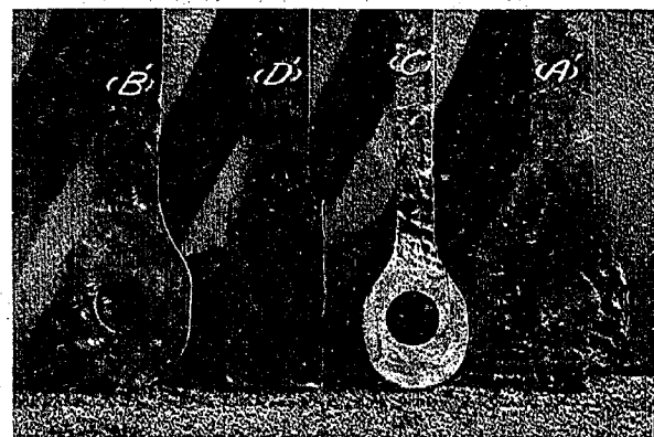
寫真第六 部材 A, B, C, D, 外側腐蝕狀態
