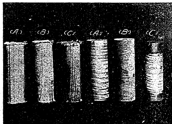
写真第四 壓 縮 試 験
