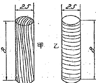
第四圖 磨 耗 試 験 片
