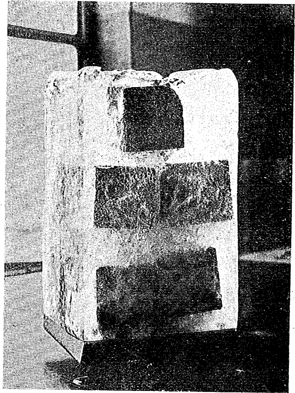
写真第三 凍結試験中の供試體
