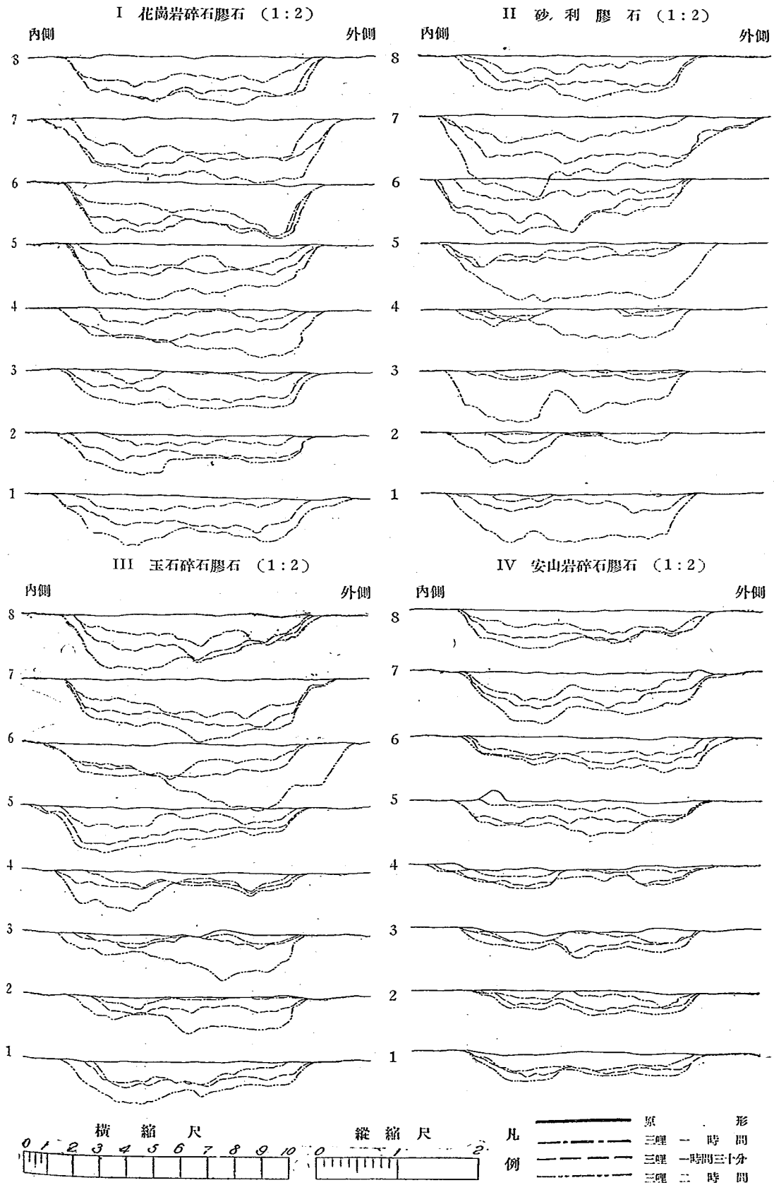
第 八 圖 乙種試験磨耗横断面圖
