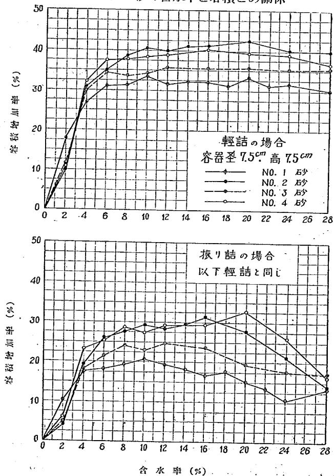
第四圖 砂の含水率と容積との關係
