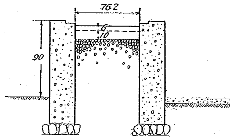
其二 横断面圖
