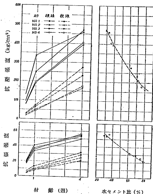
第五圖 1:2.5 モルタルの強度比較
