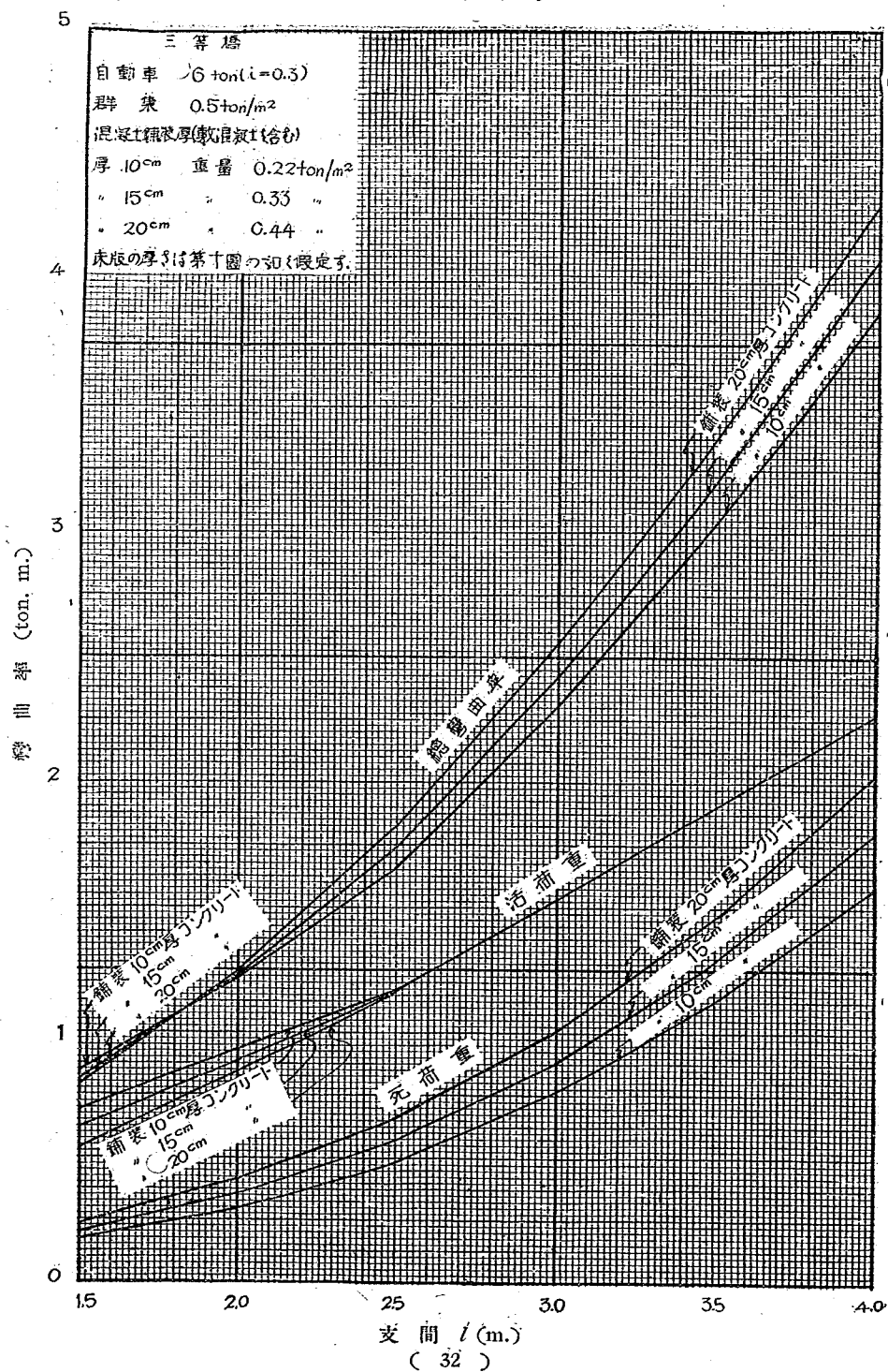
附圖第八 丁桁橋床版支間中央における單桁としての最大彎曲率 (1 m. 巾) (III-10, 15, 20)
