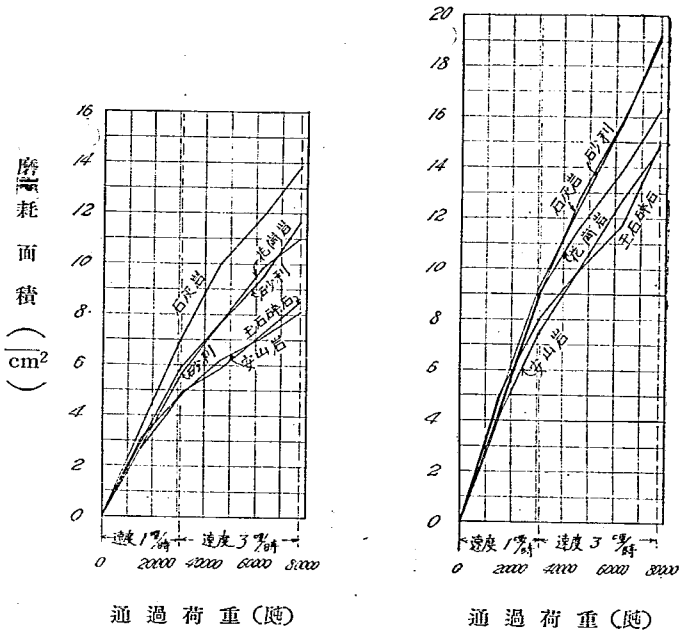
第 六 圖 甲種試験磨耗曲線圖
