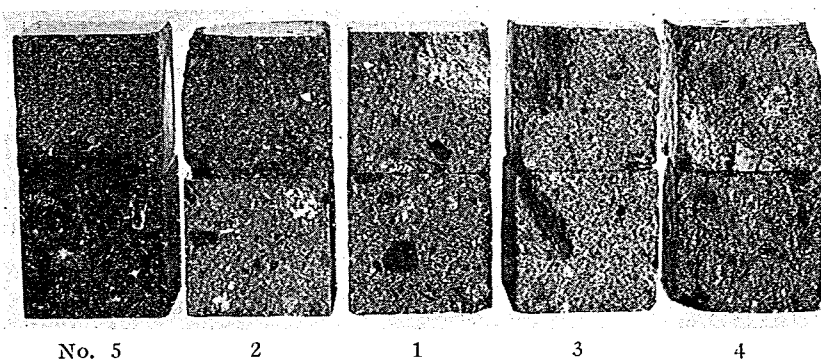
写真第二 凍結試験後の供試體
