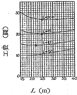
第二十一 a 圖 三等橋における主桁間隔と 工費との関係
