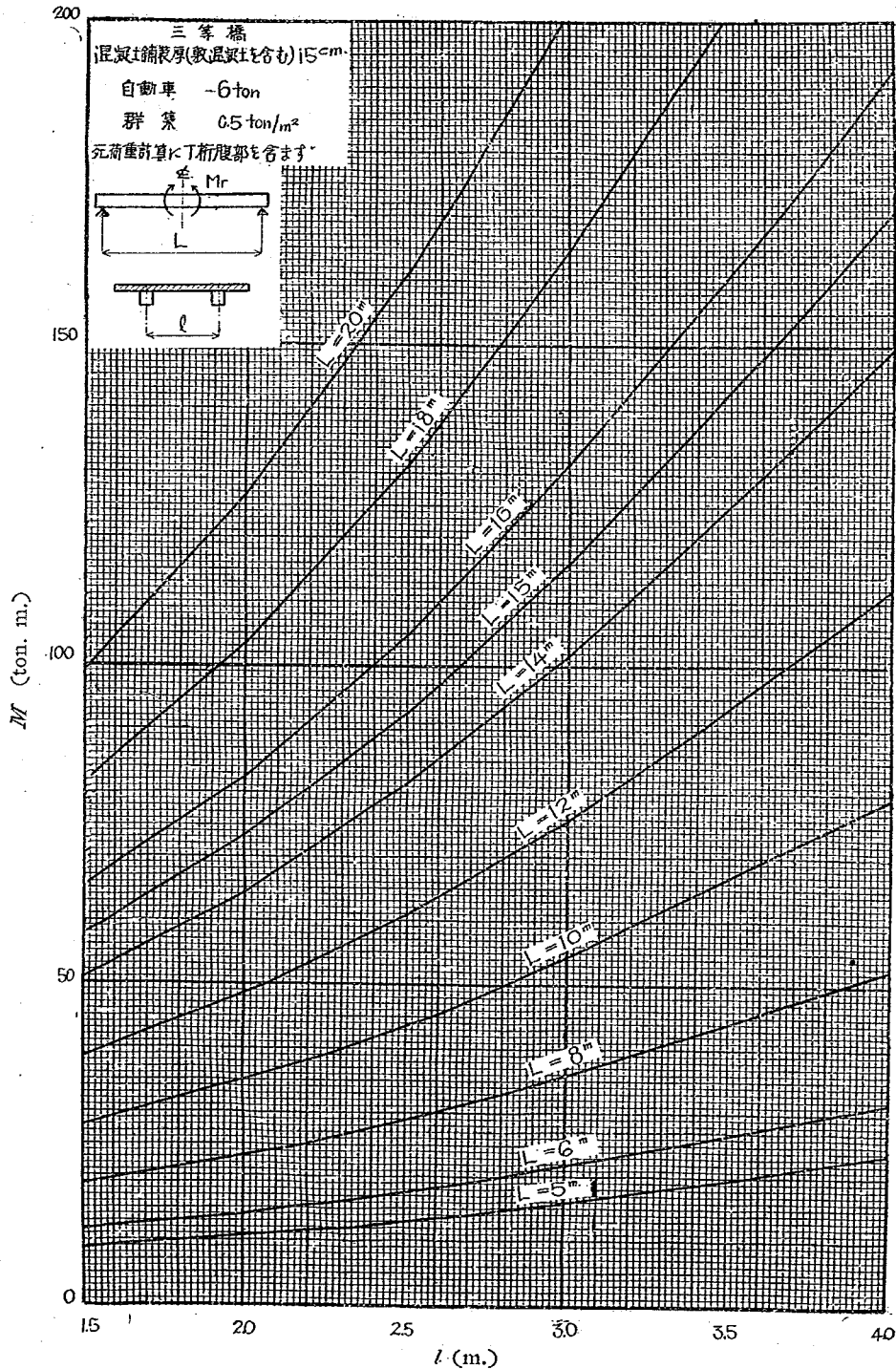
附圖第十五 丁桁彎曲率(桁1本當り) (III-15)
