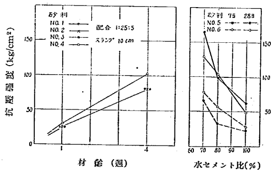
第六圖 混凝土の抗壓強度
