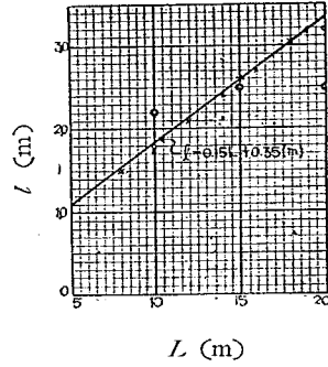
第二十一 b 圖 三等橋における主桁支間と 其の経済的間隔との関係
