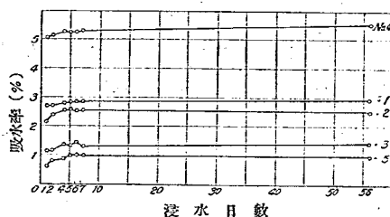
第二圖 吸水率の比較
