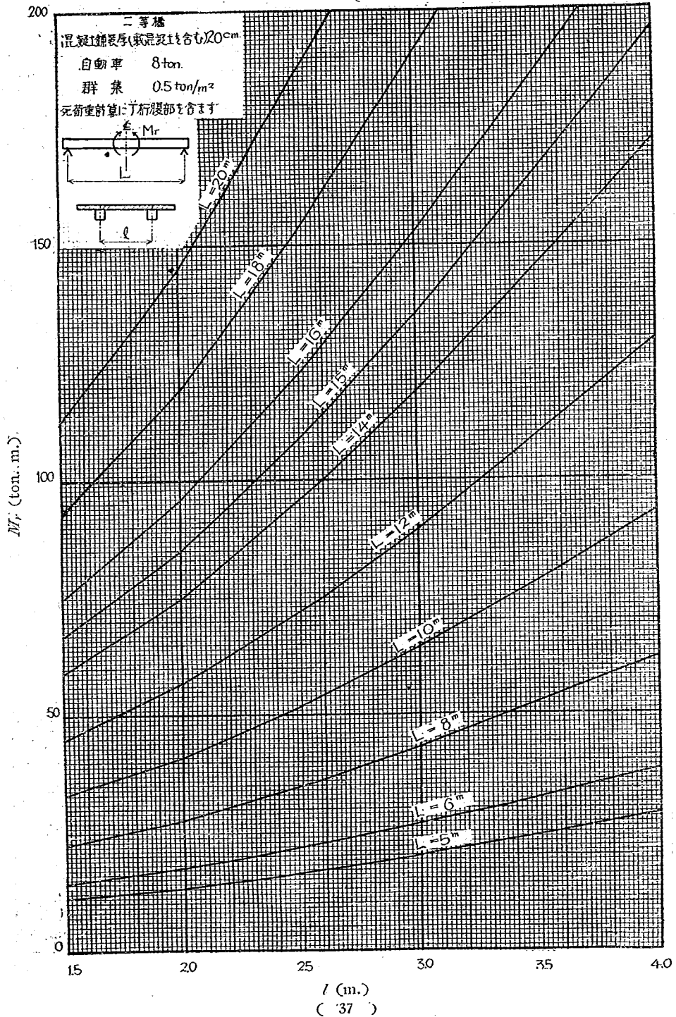
附圖第十三 丁桁彎曲率(桁1本當り) (11-20)
