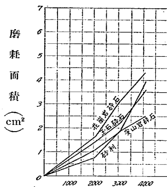
通過荷重(噸)
