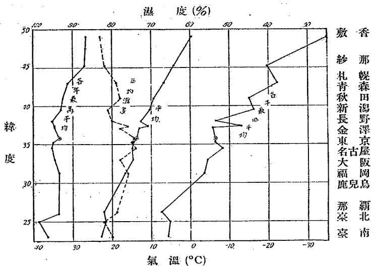
第三十二圖 緯度と気温
