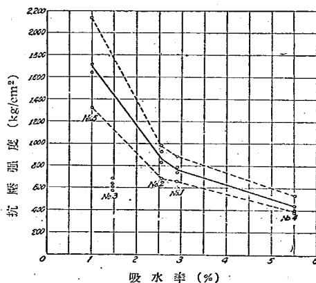
抗壓強度及吸水率の比較
