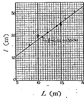
第二十二 b 圖 三等橋における主桁支間と 其の経済的間隔との関係
