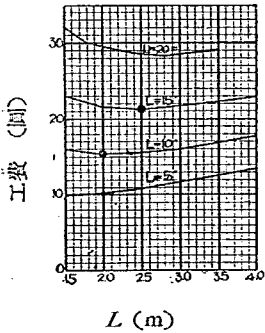
第二十二 a 圖 三等橋における主桁間隔と 工費との關係
