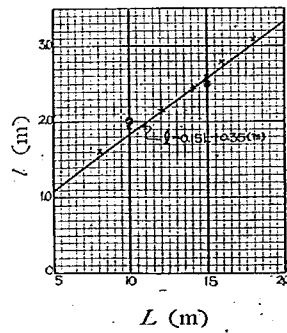
第二十二 b 圖 三等橋における主桁支間と 其の經濟的間隔との關係
