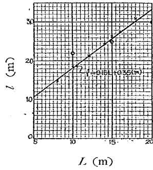
第二十二 b 圖 三等橋における主桁支間と 其の經濟的間隔との關係
