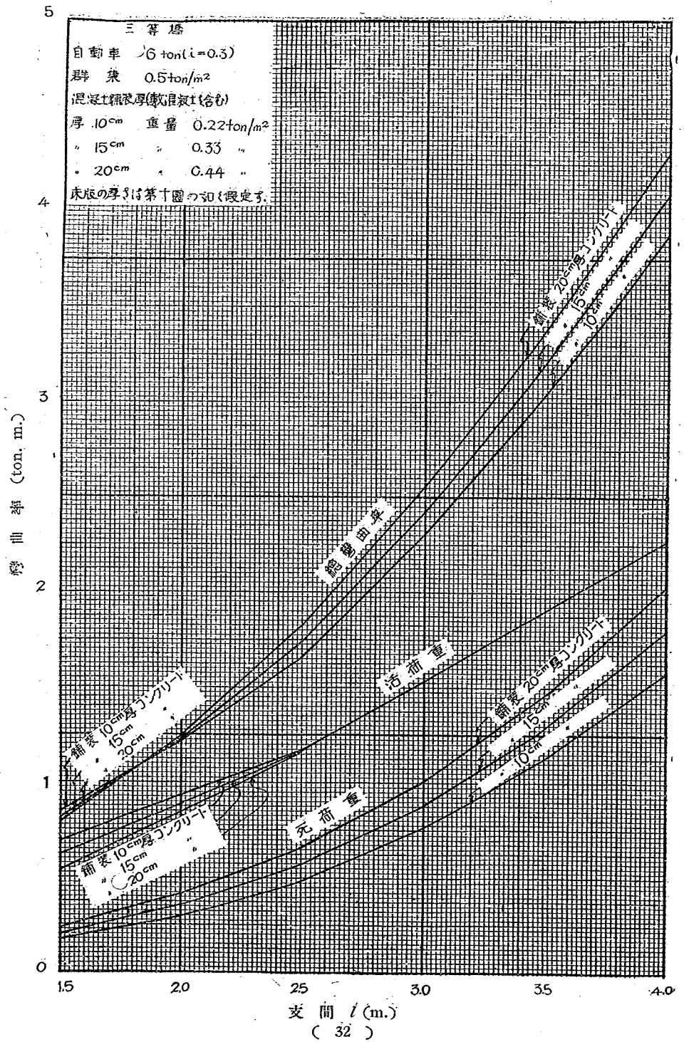
附圖第八 丁桁橋床版支間中央における單桁としての最大彎曲率 (1 m. 巾) (III-10, 15, 20)
