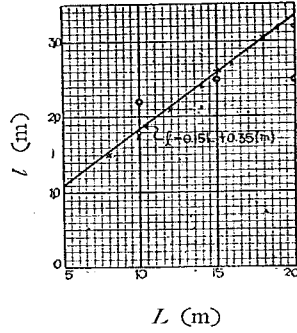
第二十一 b 圖 三等橋における主桁支間と 其の經濟的間隔との關係
