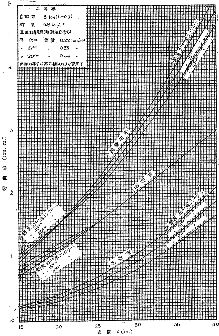
附圖第七 丁桁橋床版支間中央における單桁としての最大彎曲率 (1 m. 巾) (II-10, 15, 20).
