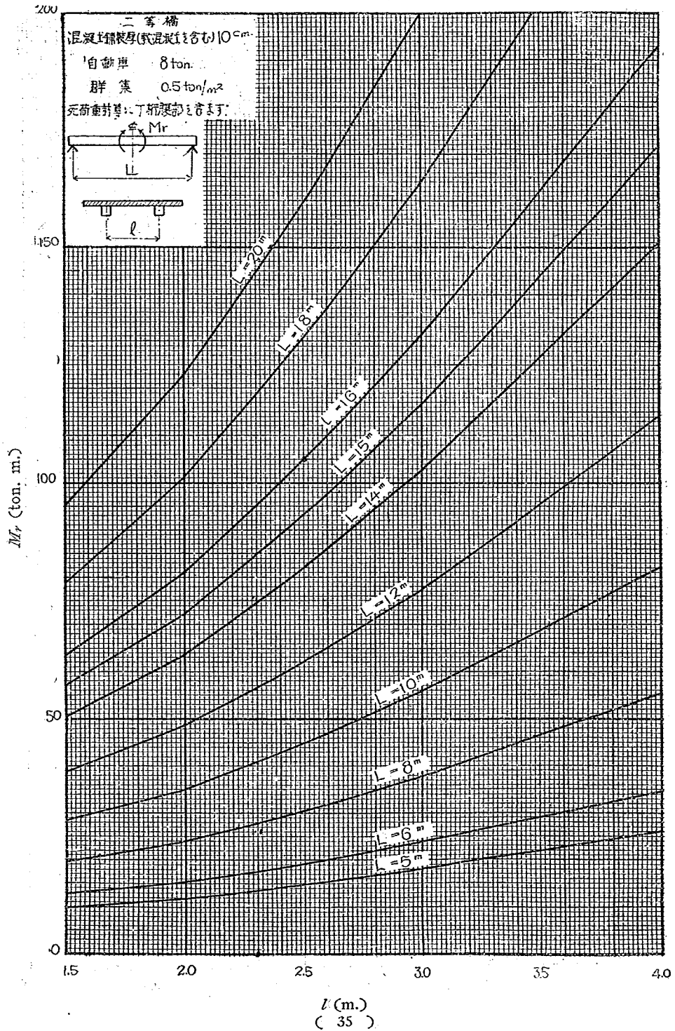
附圖 第十二 丁 桁 彎 曲 率 (桁1本當り) (II-10)
