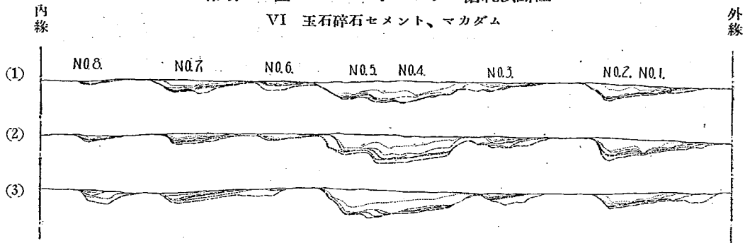
附第二圖 セメント、マカダム磨耗横断面圖
