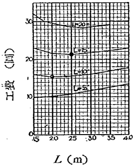
第二十二 a 圖 三等橋における主桁間隔と 工費との関係
