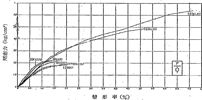
第 十 圖 天然赤土の壓力變形率に及ぼす含水率の影響 a (地層の垂直方向に加壓した場合)
