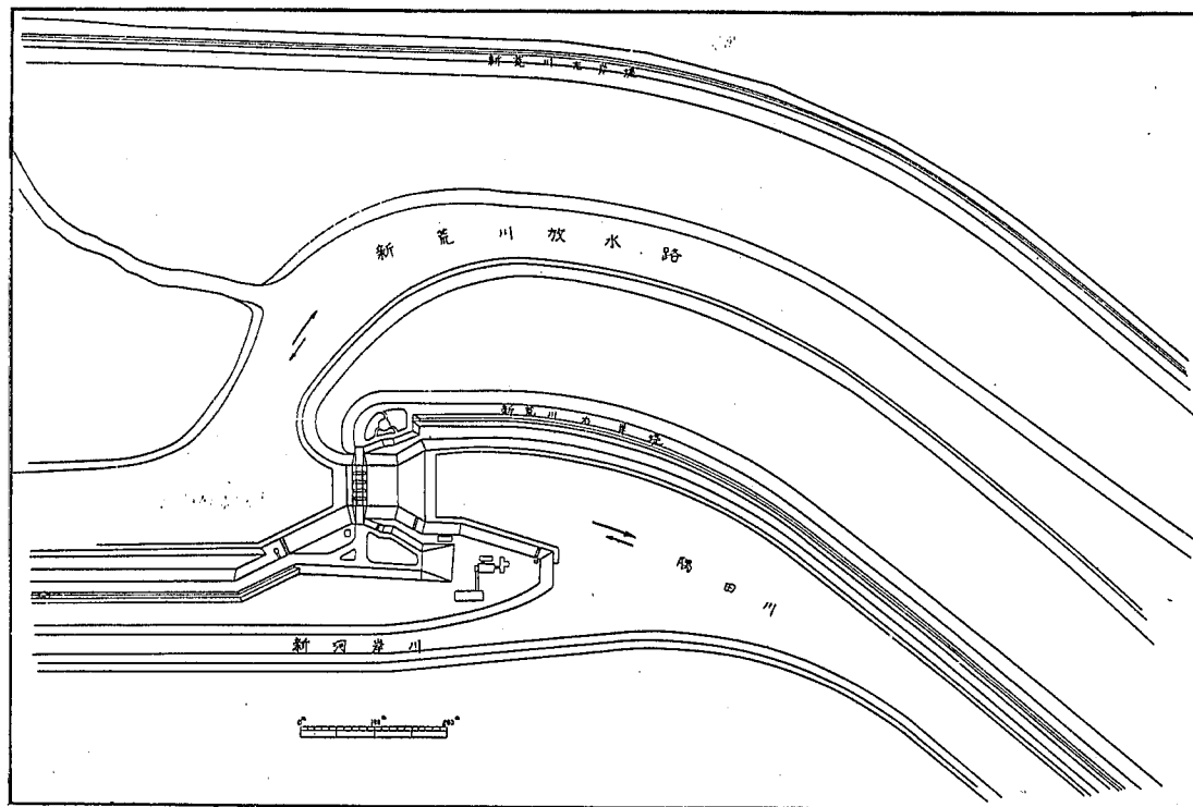
岩淵水門附近平面圖
