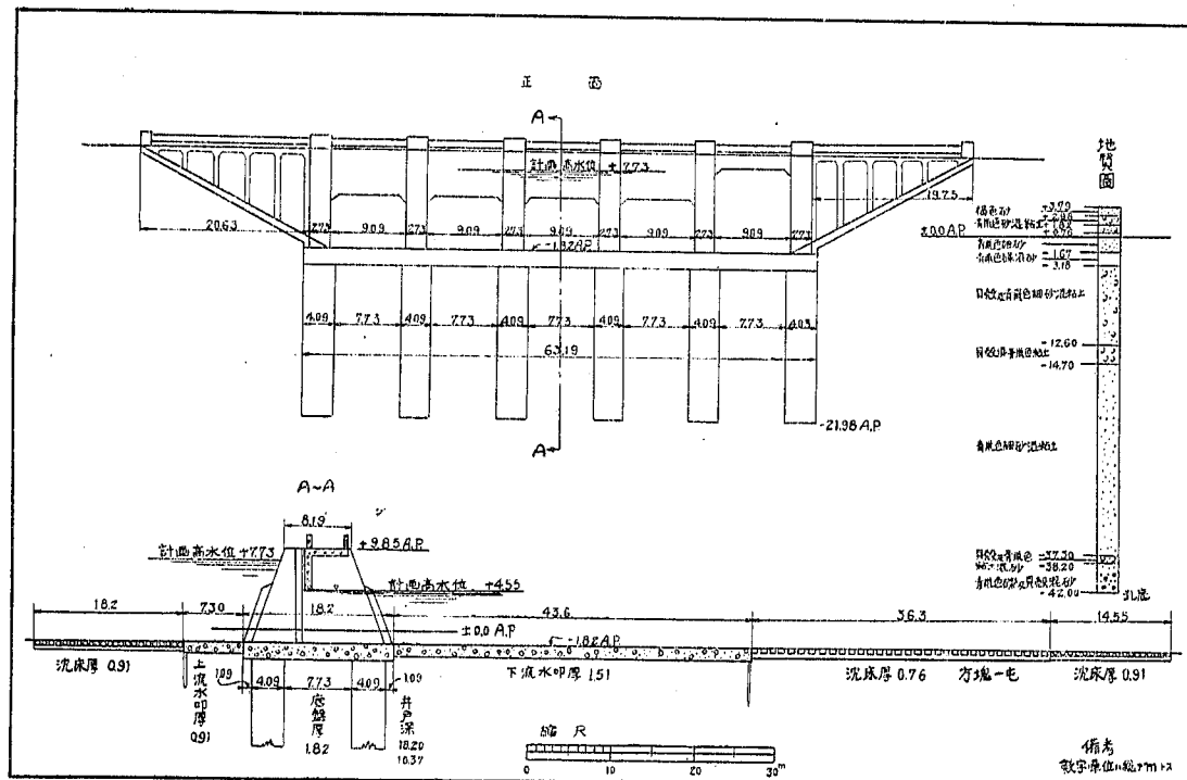
岩淵水門
