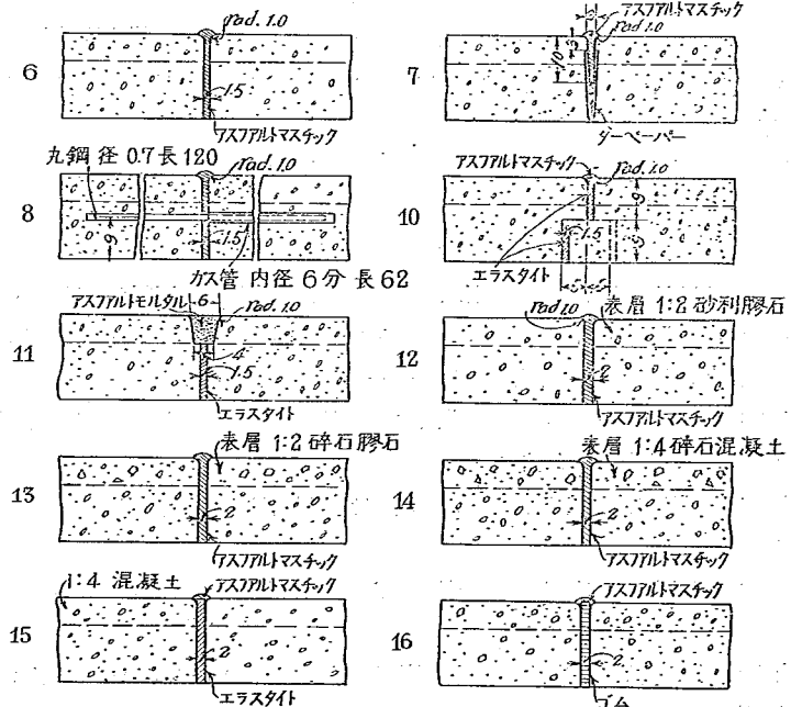
第一圖 継目構造圖
