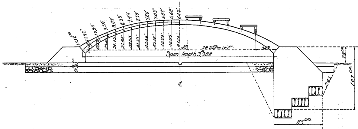
附圖第一 模型單鉸拱橋
