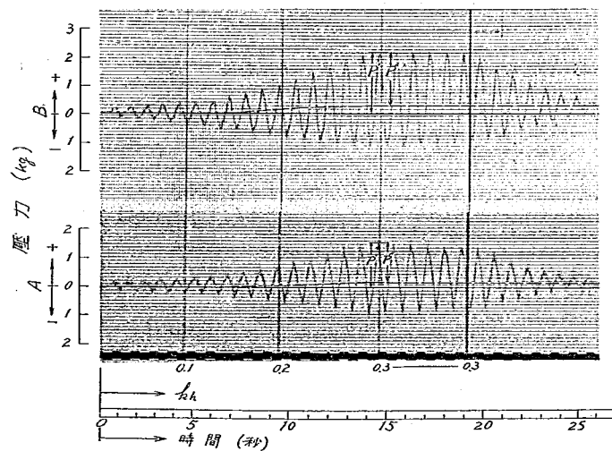
寫眞第六 振動初期土圧水平分力の變化 (2) (第四章 [8] 参照)
