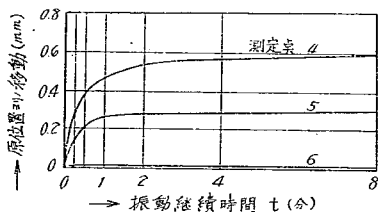
壁ノ位置ノ移動
