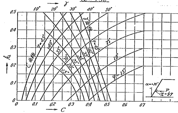
附圖第二 土壓圖表
