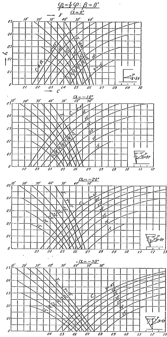
附圖第四 土壓圖表
