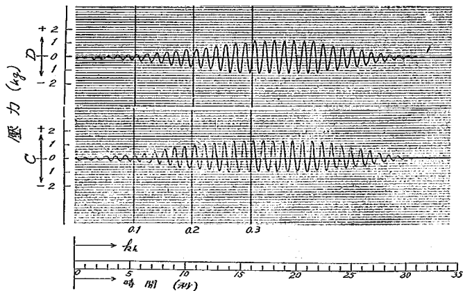
写真第九 安定状態に於ける土圧垂直分力の變化(第五章[12]参照)
