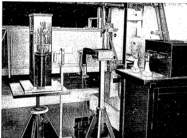
寫真第一 振動函及測定裝置一般(第一章參照)
