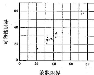
第二圖 液狀限界と可塑性 限界との關係
