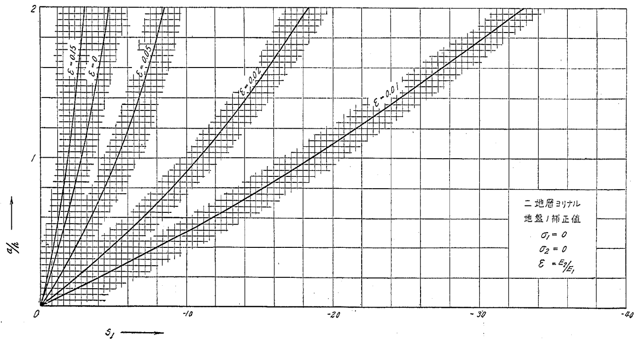
附 圖 第 一 (b)
