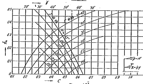
附圖第八 土壓圖表
