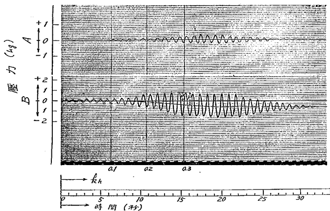
写真第八 掘き固めをなしたる場合の土圧水平分力の變化(第四章[10]参照)
