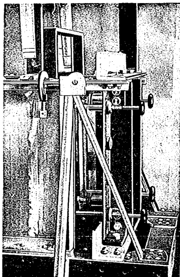
寫真第二 壓力計及支柱(第一章參照)
