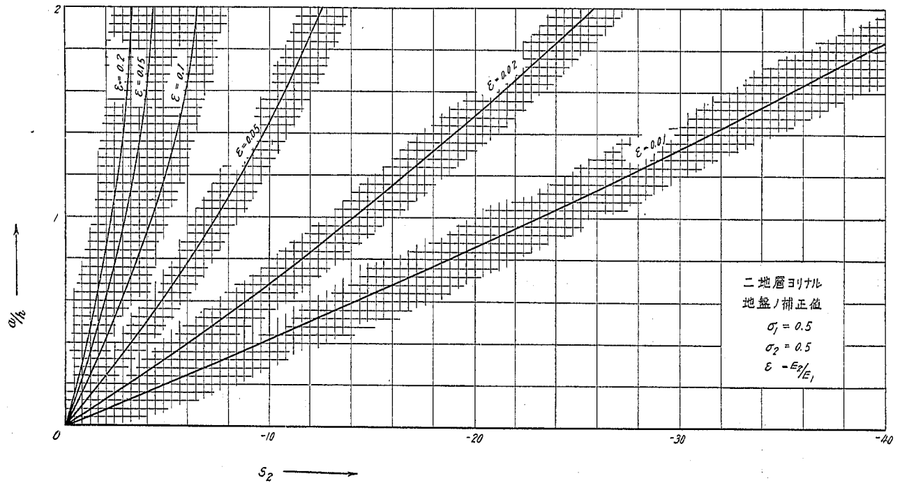
附圖 第二 (b)
