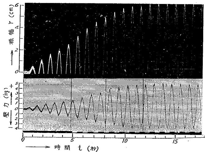
寫眞 第五 筒の振幅と土圧水平分力の變化 (第五章 [11] 参照)
