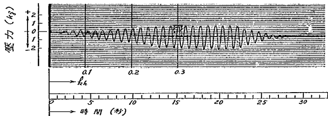
写真第七 振動初期土圧垂直分力の變化(第四章[8]参照)
