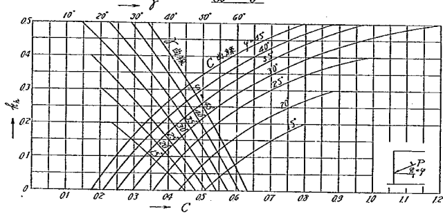
附圖第三 土壓圖表
