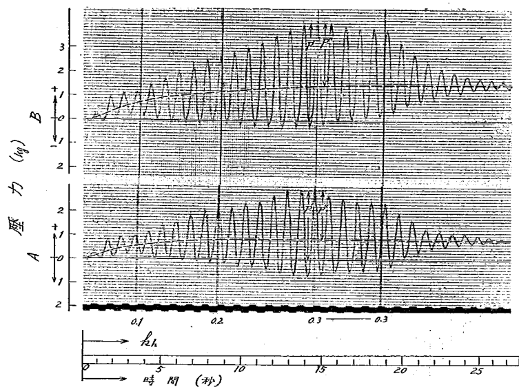
寫眞第六 振動初期土圧水平分力の變化 (1) (第四章 [8] 参照)
