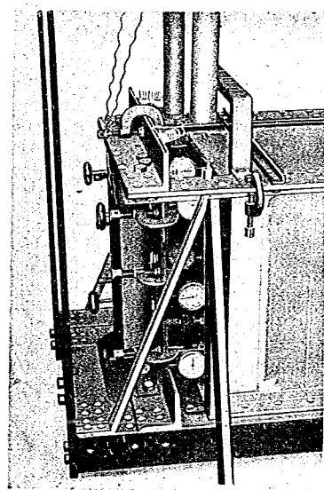
寫真第三 壁面振動測定裝置(第一章參照)
