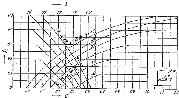
附圖第七 土壓圖表
