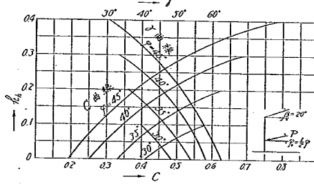
附圖第十二 土壓圖表
