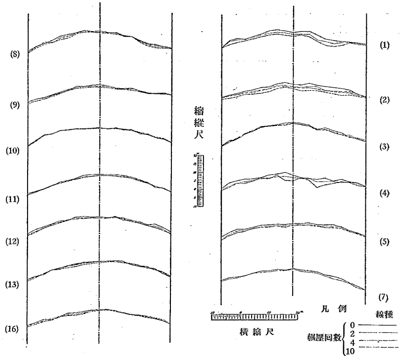
第七圖 輾壓に因る路床の沈下
