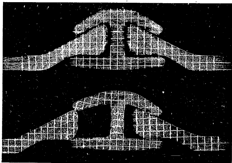
寫真第五 Krupp 銅矢板縱手強度試驗片
