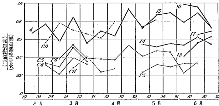
第二十圖 右岸の水平移動距離に對する河床隆起高の變化
