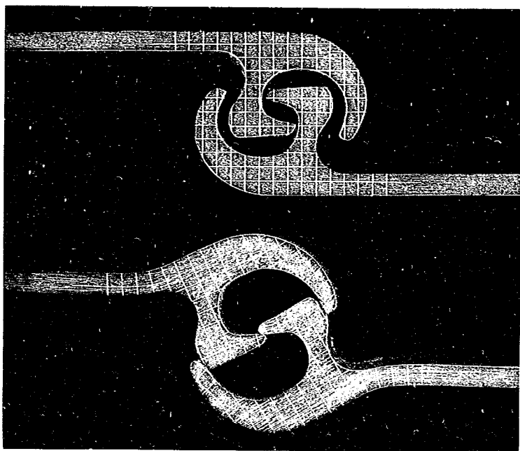
寫真第三 Lackawanna 銅矢板繼手強度試驗片
