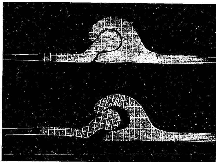
寫真第六 Klöckner 銅矢板縱手強度試驗片
