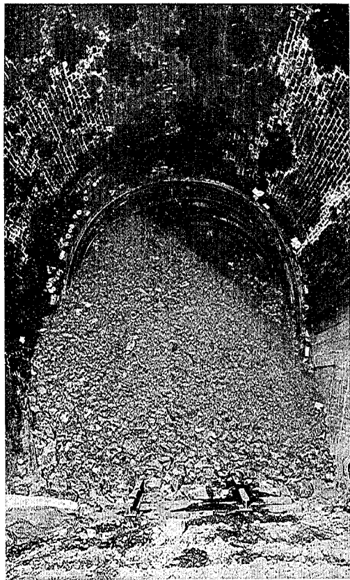
寫眞第二十三 隧道内の壊崩。西口より約80mの上り線坑内に崩落した築塊岩及煉瓦。(2月10日撮)
