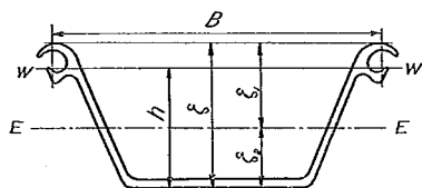
第九圖 Lackawanna DP 型鋼矢断面形
