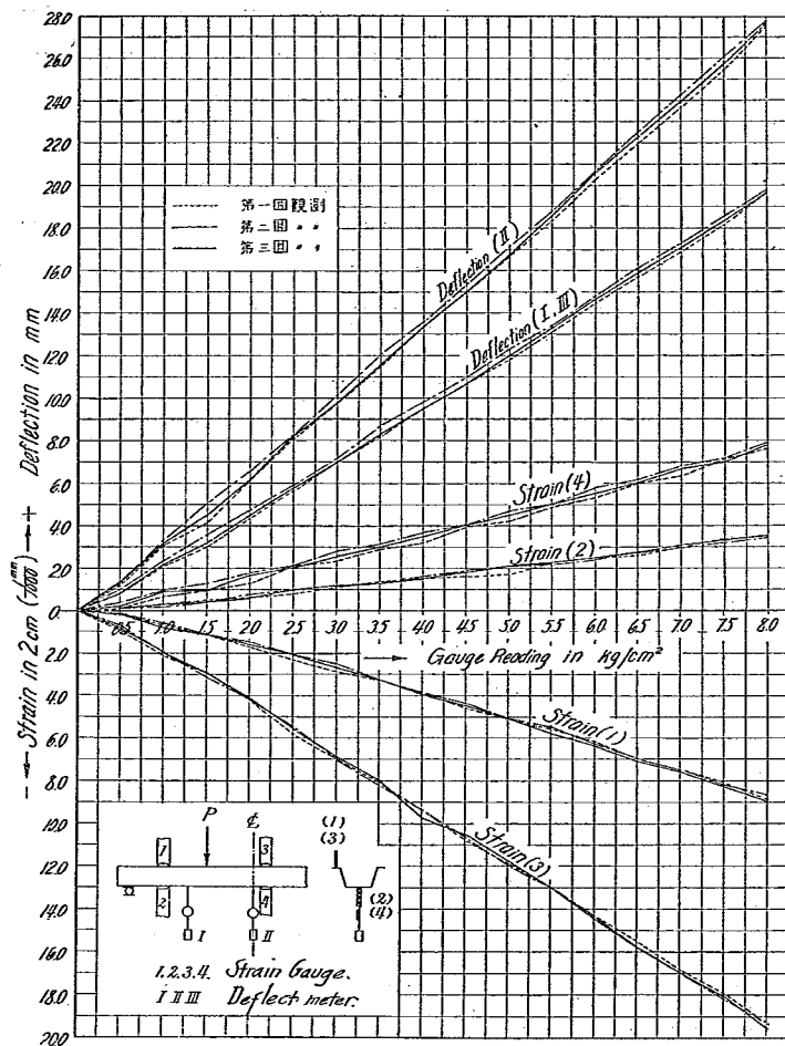
第五圖 製鐵所銷矢板抗曲試験成績 (第二號 A 型)
