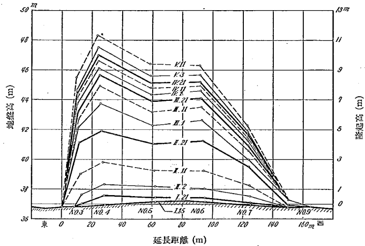
第十七圖 府縣道奈良大阪線路面の隆起
