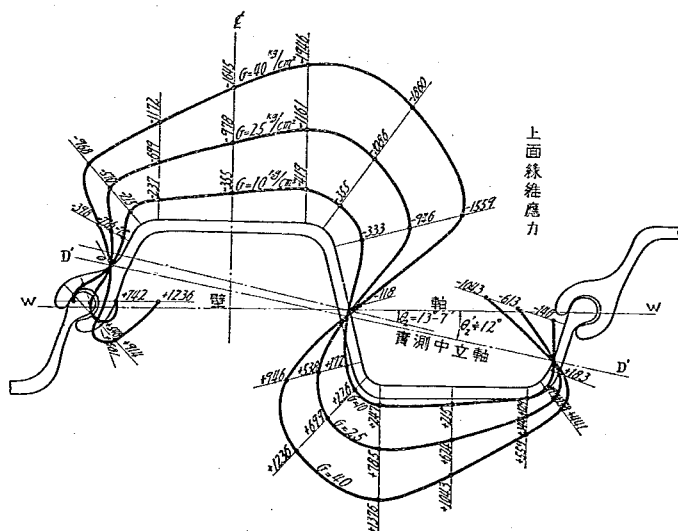
第四十九圖 Terres Rouges 銅矢板壁抗曲試驗應力分布圖 (其二)
