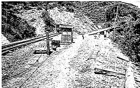
寫眞第四 西口附近の山崩。7月5日拂曉崩壊して線路及徒歩連絡道を埋没遮斷した。(7月6日撮)
