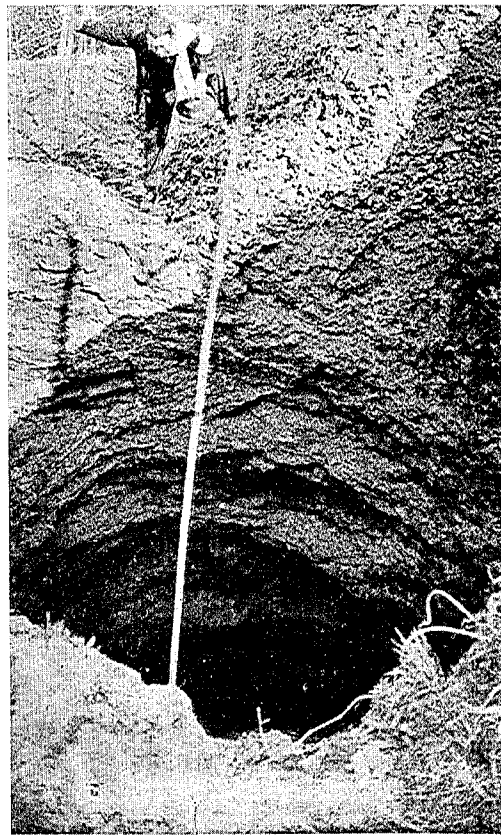
寫眞第二十四 隧道上に當る地表に生じた陥没穴。2月13日雪中筋に生じたもの、上徑3m、下徑8m深さ10m
