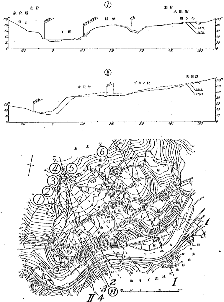
第十五圖 地ニ地域横斷面の變化
