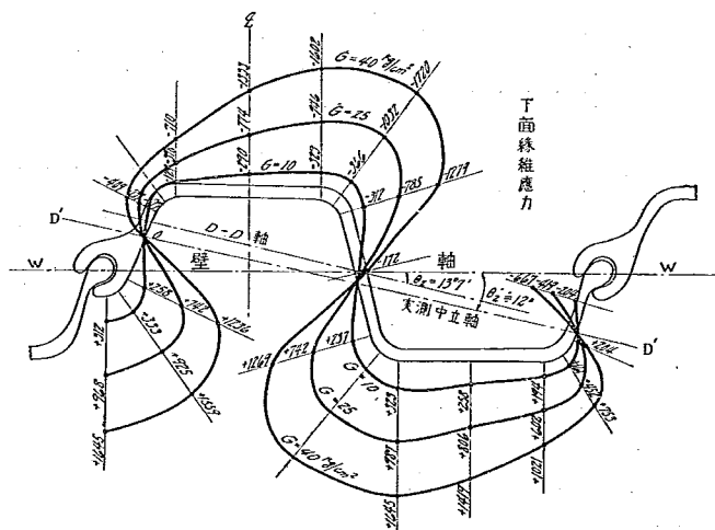
第四十九圖 Terres Rouges 銅矢板壁抗曲試驗應力分布圖 (其二)
