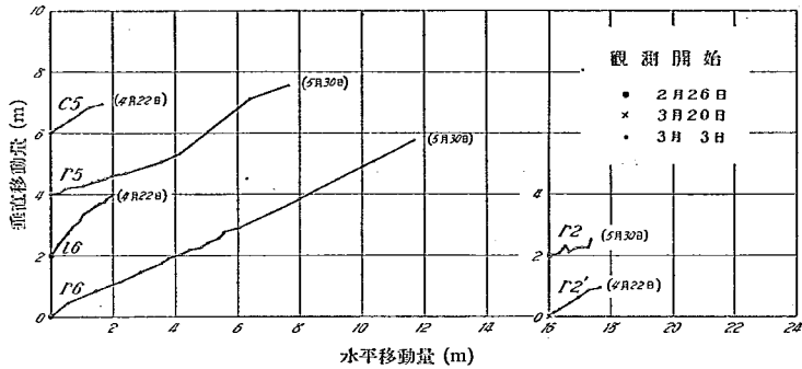
第十九圖 隆起地域に於ける測點の移動仰角
