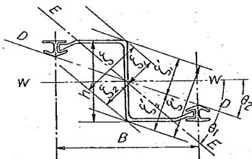
第十三圖 Krupp 型鋼矢板斷面形
