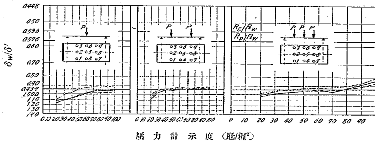
第三十四圖 Larssen 複斷面矢板壁抗曲試験 \delta_w/\delta' 圖表 (其二)
