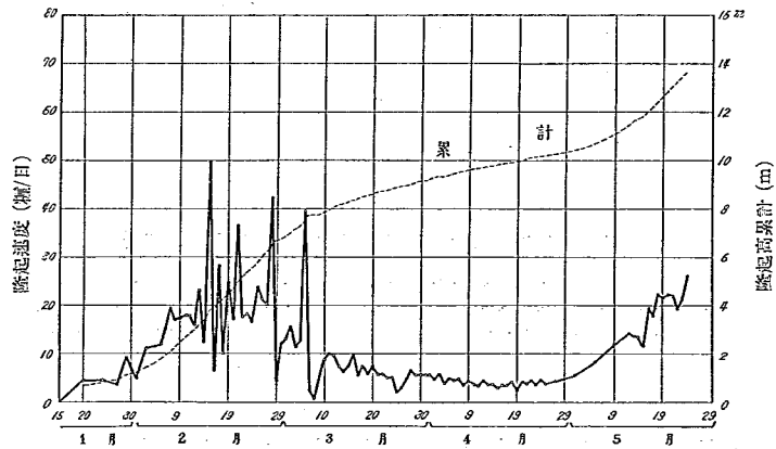
第十八圖 府縣道奈良大阪線路面の隆起速度及累計
