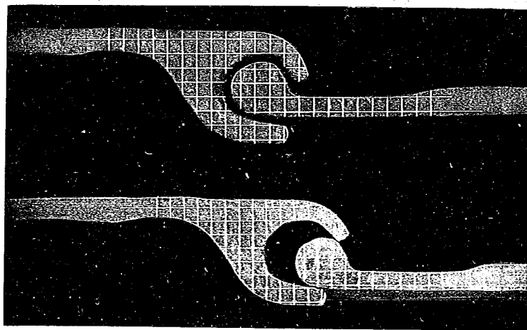
寫真第四 Terres Rouges 銅矢板繼手強度試驗片
