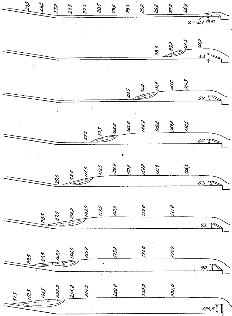
第 八 図 a 阻柱なき場合の水面形状測図
