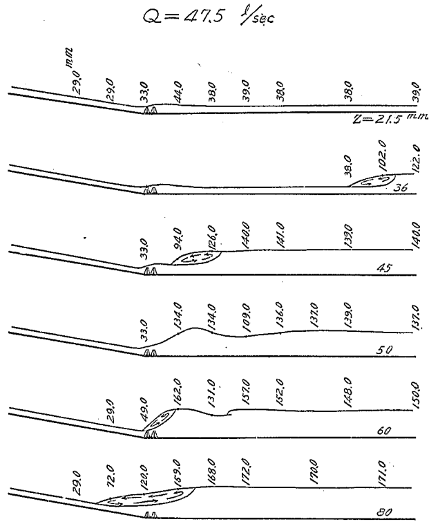
第十四圖 柱模型 IV
