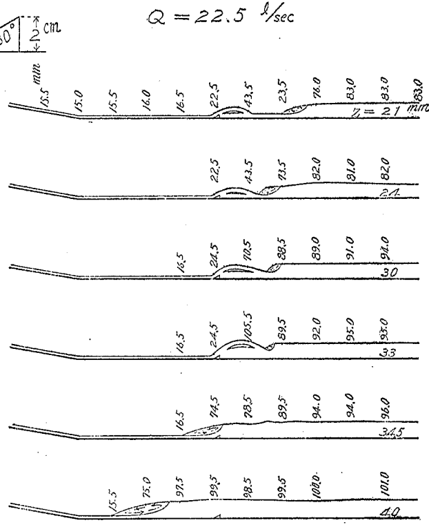
副堰堤試驗
