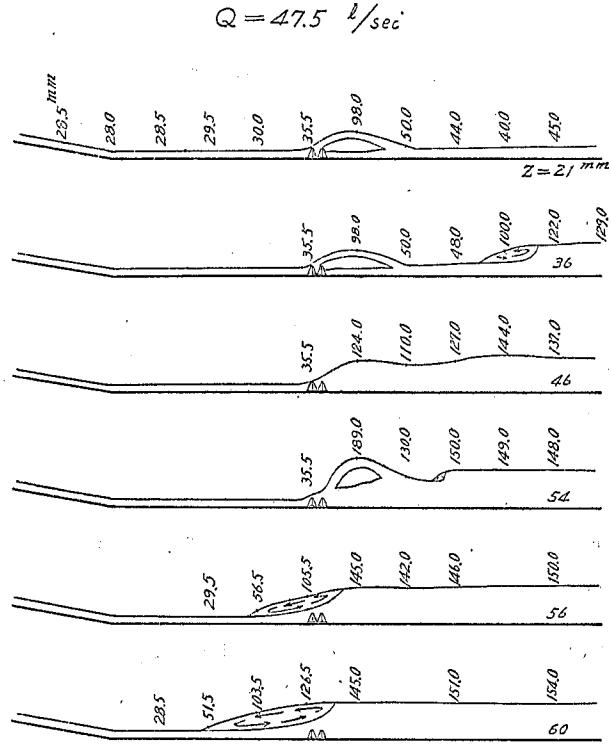
第十四圖 a 阻柱模型 IV
