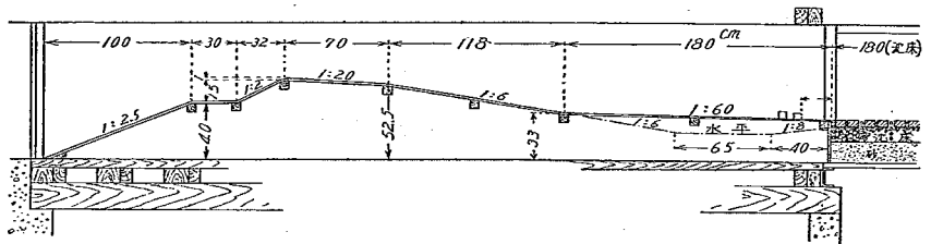
第十九圖 橫溢流提洗掘試驗設備縱斷面圖
