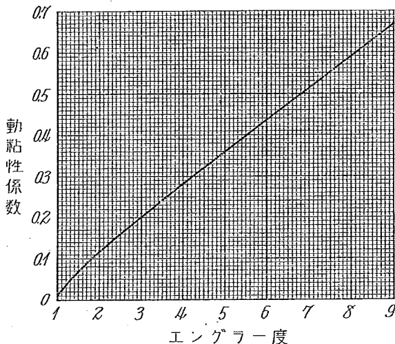
比粘度一粘度曲線 (W.H. Herschel に由る)
