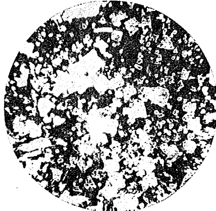
第二十八圖 鑛 滓
