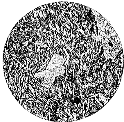
第十六圖 橄欖玄武質安山岩
