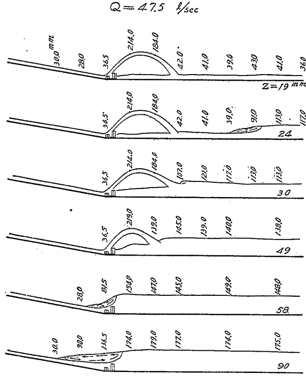
第十圖 b 阻柱模型 II
