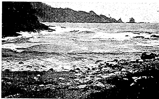
寫眞第十二 九戸郡田野畑村離賀。寫眞の白い石は津浪にて打上げられたもの。最大のもので一個約 0.15 m 3 。この海岸汀線より約 100 m の距離に自然勾配にて高さ約 8 m 上つた所に高さ 4 m の線柱間知があつて津浪の勢力を大いに弱めた。 (5 月 29 日撮)
