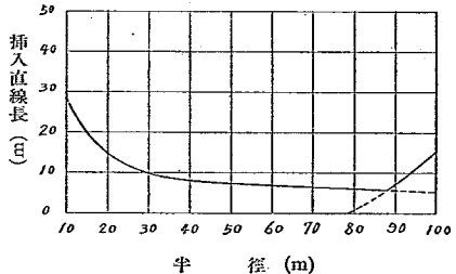
第 16 圖 摩擦係數 0.10 の場合
