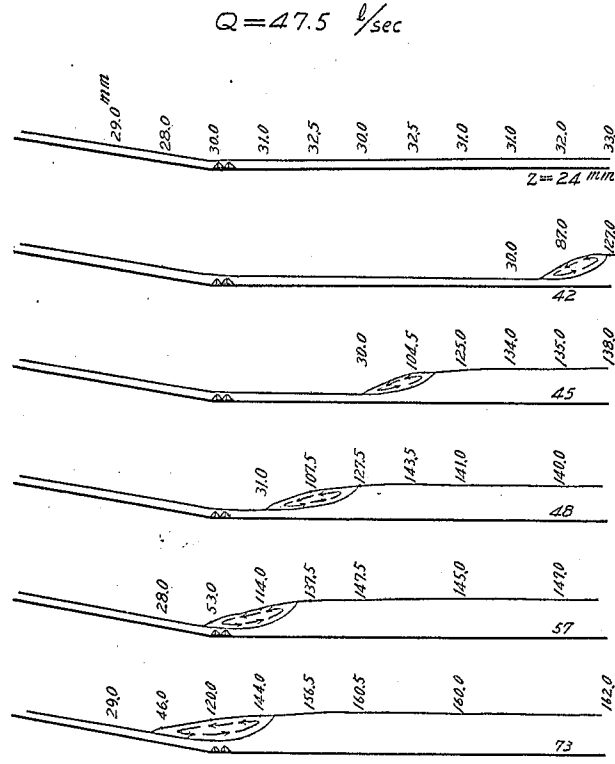
第十一圖 阻 柱 模 型 III
