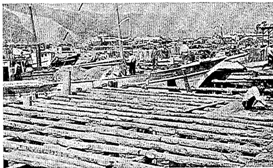
写真第三十九 釜石町漁船用棧橋。写真は復旧工事中的のものであるが同様の構造のものが津浪の場合には写真三十八の如く上部が殆ど全部流失した。(5月27日撮)
