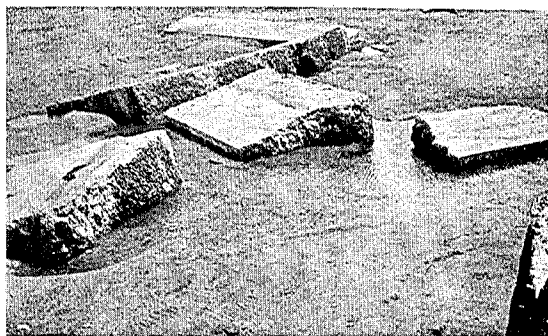
寫眞第四 八木。船溜り用護岸。寫眞の右端前方には舊位置に残つた壁が見える。中央にある混凝土ブロックは引き浪により倒され破壊散亂して流れ出た裏込土砂の中に埋つたもの。
