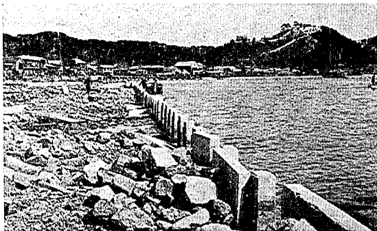
写真第二十一 下関伊都宮古町宮古港。鉄筋混凝土柱の間にスラブを樹て込んだ構造の物揚場岸壁。裏込が流された爲にスラブの一部が散乱したもの。寄せ波及引き波の兩作用に依つてスラブは或は内に或は外に移動してゐる。(3月6日報)
