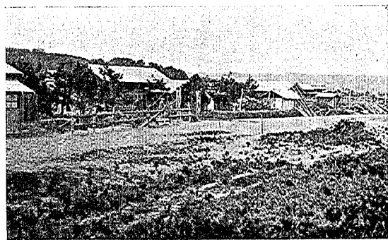
写真第八 九戸郡野田村赤代海岸。写真中央稍左の家は写真に見える様な低い堤防(断面高さ0.6m、巾0.4~1.0m)を平常の暴風の浪を防ぐ目的で築いてあつたので隣の之なき家は家財等が流され僅に柱が残つたのみであつたがこの家は何等の破壊作用を受けなかつた。
