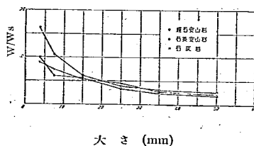
第二圖 碎石の磨損率( W' )と標準試験に依る磨損率( W )との關係
