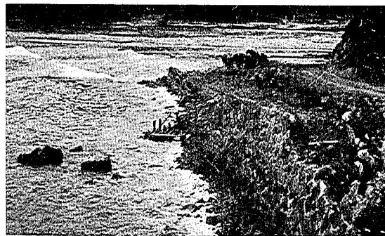
写真第四十三 小白濱片岸間知護岸。写真四十二の護岸の一端の破壊した一部。
