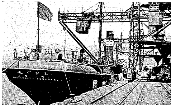
写真第三十七 釜石町鎮山棧橋。灣内に突出してゐるにかゝらず殆ど被害を受けなかつた。僅に根本に於て多少破損したのみである。
