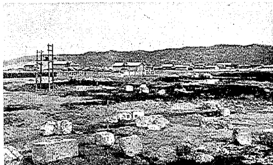
写真第六 九戸郡久慈町湊海岸。岩手縣久慈港工務所の工事用混凝土方塊(重量一個約6t)600個が製作の後海岸の汀線より約120m線に4列に平均水面より6.8mの高さの砂丘の裏に長く(列の間隔約1.0m、横の間隔約0.3m)配置してあつたものが散亂摩滅した状態。(5月30日撮)
