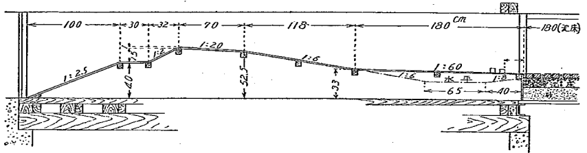
第十九圖 横溢流堤洗堀試験設備縦断面圖
