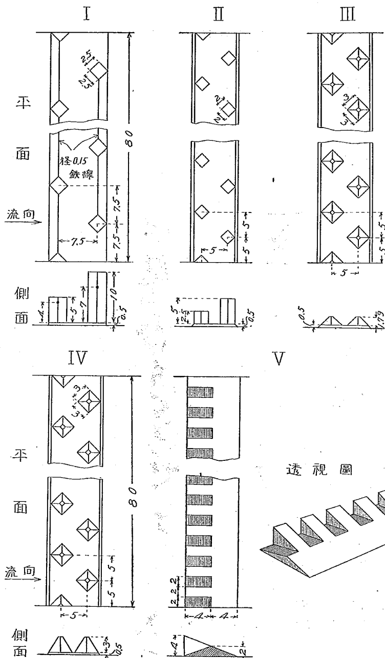
第七圖 阻柱模型
