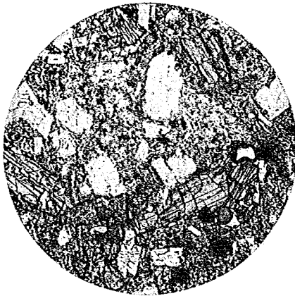
第十三圖 橄欖輝石安山岩
