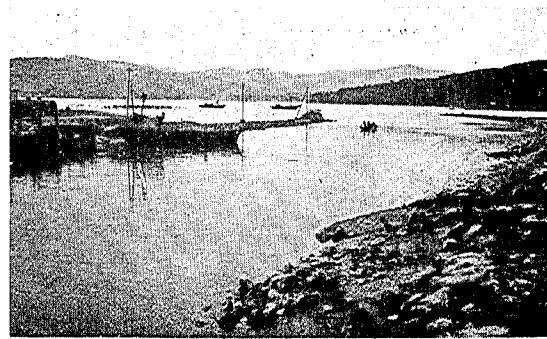
写真第七十 本吉郡志津川町尋流堤。写真の前方右の絶張 り尋流堤の根本は津浪による破壊。
