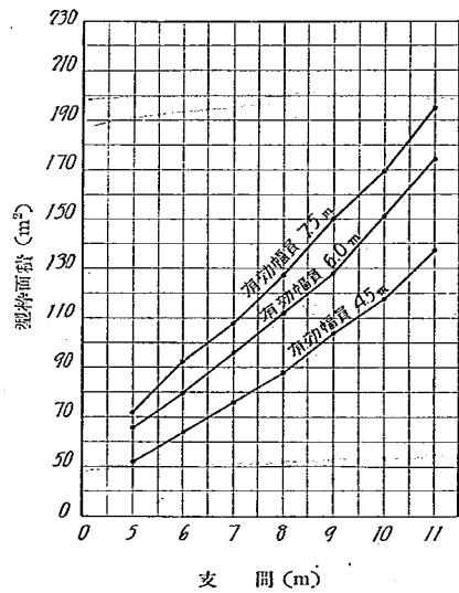
第五圖 所要型枠面積
