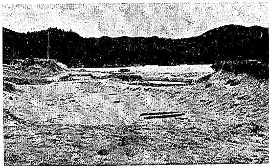
寫眞第七十六 牡鹿郡大原村大谷川。海岸道路築堤の一部流失。築堤は粘土分渺なき砂よりなつてゐた爲に津浪により容易に破壊された。
