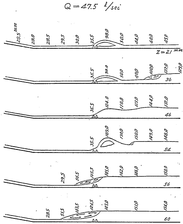
第 十 二 圖 a 阻 柱 模 型 IV
