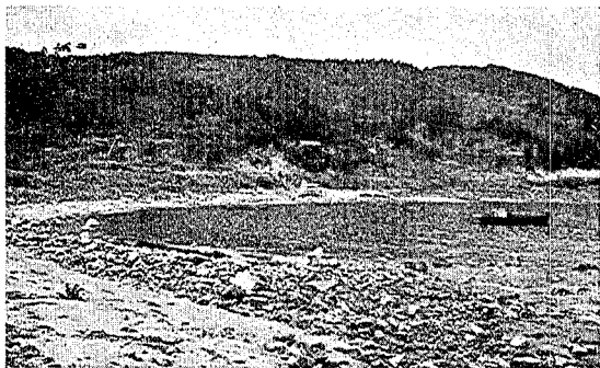
写真第五十六 気仙郡廣田村根岬。綾里白濱に次で今回の津浪が高かつた根岬及集落。高さ最大 26.7 m。写真の白い石は多く津浪にて打上げられたもの。大きさ最大 1.5 \times 0.8 \times 0.8 m。(5月24日撮)
