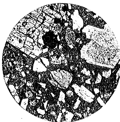
第十圖 複輝石安山岩
