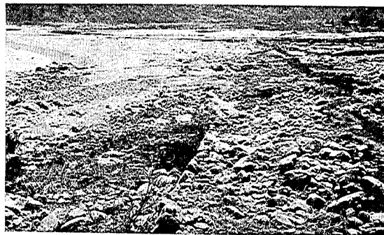
写真第四十五 氣仙郡吉濱村。明治 29 年の津浪の被害甚大なりしに依り築造した防浪堤(斷面底巾 9.8 m, 天端巾 2.7 m 高さ最大 5.5 m 海に面する側は 3 分勾配にて間知碁の土堤)は今回の津浪で全部流失。写真は長さの方向に撮つたもので右方に一部基礎部分の残を見る。
