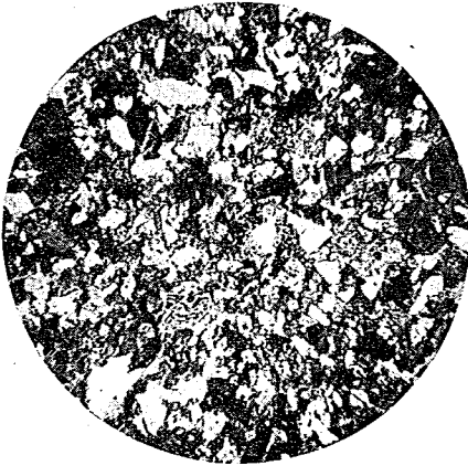
第二十三圖 砂岩
