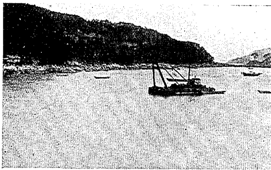
写真第四十六 気仙郡越喜来村崎濱。写真の起重機船（揚力30 t）は津浪當時も略この位置に汀線より約150 mの所に碇泊してゐたが浪の爲一旦岸まで押流されたがエンジンに依り沖の碇を巻き第二の波に乗つて元の位置に歸つた。浪の高最大7.3 m。（5月26日撮）
