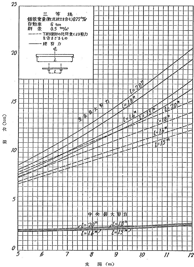
第二圖 丁桁最大剪力
