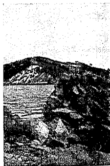
寫眞第二十六 宮古町。埋立護 岸線積間知の崩壊。(3 月 6 日報)
