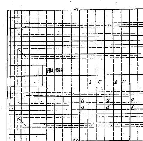
鐵筋表
