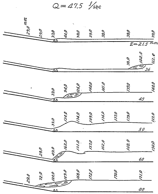
第十二圖 阻 柱 模 型 IV
