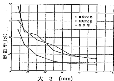
第一圖 碎石の大きさと磨損率との關係
