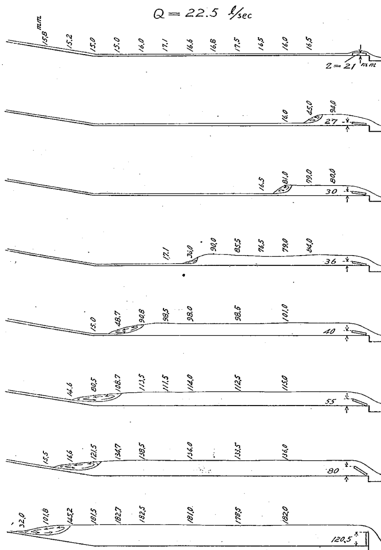
第八圖 6 阻柱なき場合の水面形
