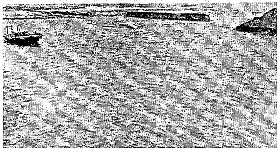
写真第五 八木。船溜り外壁及防波堤。写真の後方中央に横に延くある防波堤(寸法高2.0m以上、市天端に於て1.65m下部に於て2.15m)はその儘残りその内側の船溜り外壁(寸法写真第三のものと畧同様、但し水深が大なるだけ高さ大)は破壊された。写真の右端に残った一部を見る。
