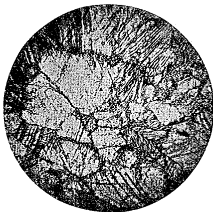
第十九圖 結晶質石灰岩
