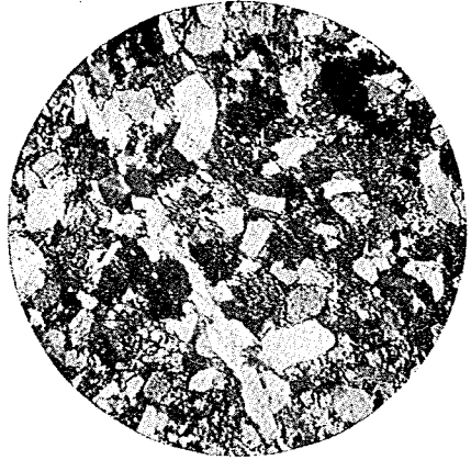
第二十二圖 硬砂岩
