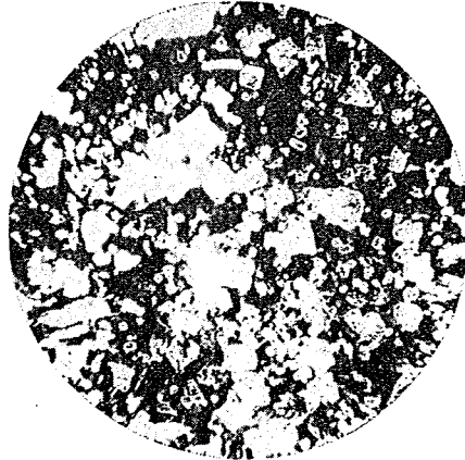
第二十八圖 鑛 滓
