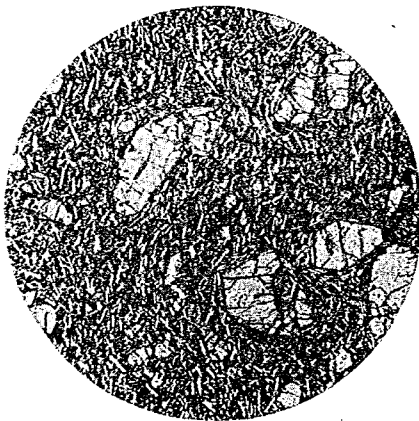
第十五圖 古銅輝石安山岩 (讃岐岩)
