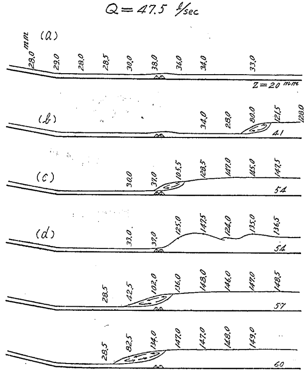
第 十 一 圖 a 阻 柱 模 型 III
