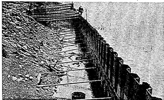
写真第五十三 気仙郡大船渡町海岸。岩手県大船渡港工事、八幡製鐵所鐵矢板長 9 m (水深 4 m) は津浪の際寫眞の如き状態にあり工事中の爲一部分掘損及取付溝形鋼がなかつたものは後方に彎曲した。寫眞後方の支へ木村は之を修正する爲のもの。 (5 月 25 日報)
