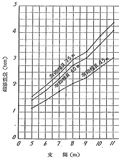
第四圖 所要鉄筋重量
