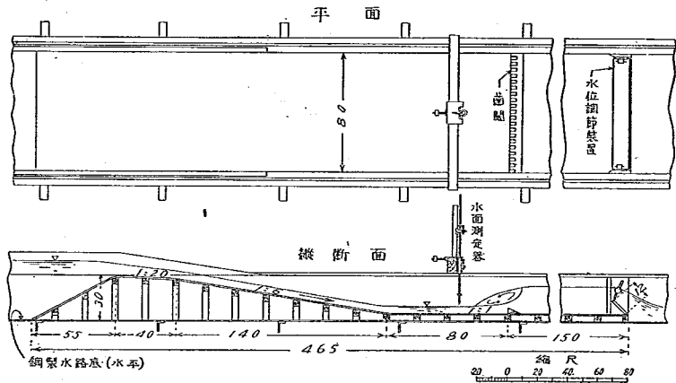
第 六 図 阻 柱 試 験 装 置 (単 位 種)
