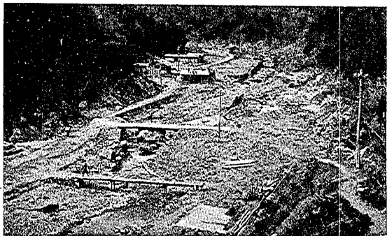
写真第十七 小本村茂師。寫眞のバラック及橋梁は其後築造されたもので津浪はその渾の奥深く約 650 m 浸入その間の家屋等悉く流失、津浪の高海岸に於て最大 15.1m(5 月 28 日報)
