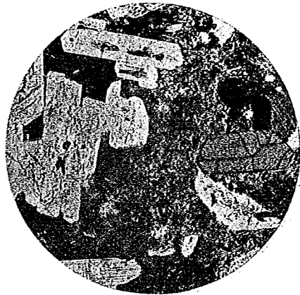
第十四圖 橄欖輝石安山岩
