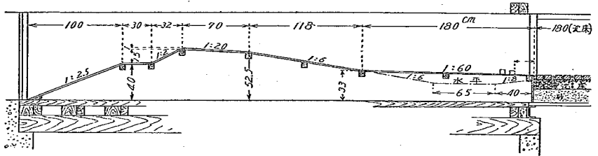
第十九圖 横溢流堤洗掘試験設備縦断面圖
