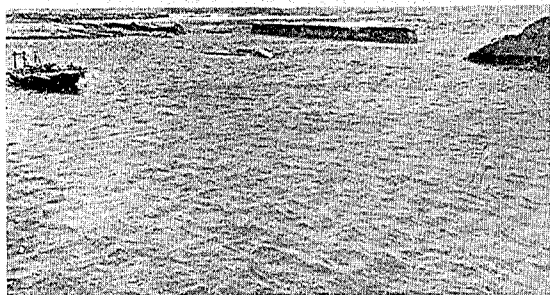
写真第五 八木。船溜り外壁及防波堤。写真の後方中央に横に延くある防波堤(寸法高2.0m以上、市天端に於て1.65m下部に於て2.15m)はその儘残りその内側の船溜り外壁(寸法写真第三のものと略同様、但し水深が大なるだけ高さ大)は破壊された。写真の右端に残った一部を見る。
