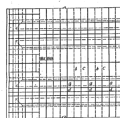
鐵筋表
