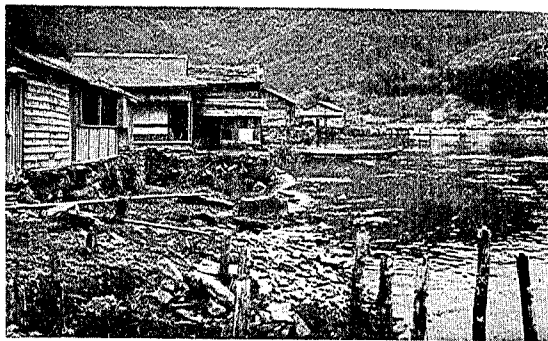
寫眞第七十四 雄勝。この附近に産するスレートに依る空積護岸は大部分破壊を免れた。この部落では寄せ波よりも引き波の勢力が大であつた。
