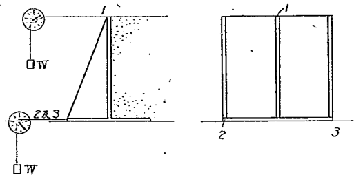
第8圖 1.2 米 試験函の \varepsilon の測點
