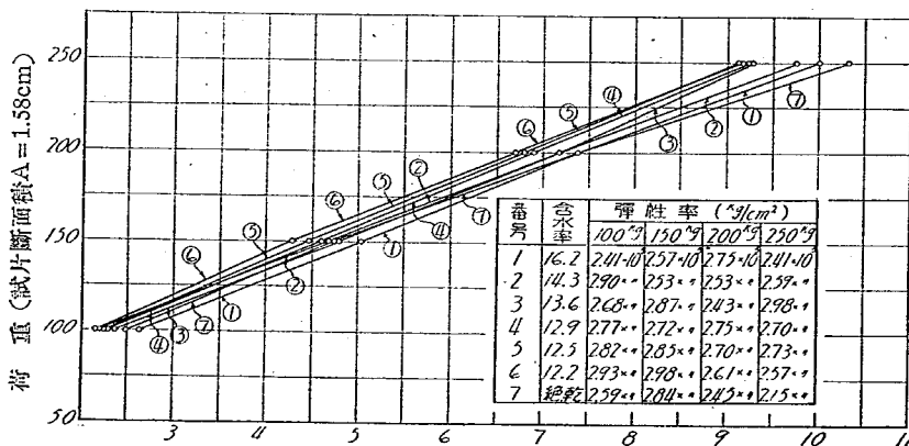
第9圖 含水率の變化と弾性率の關係
