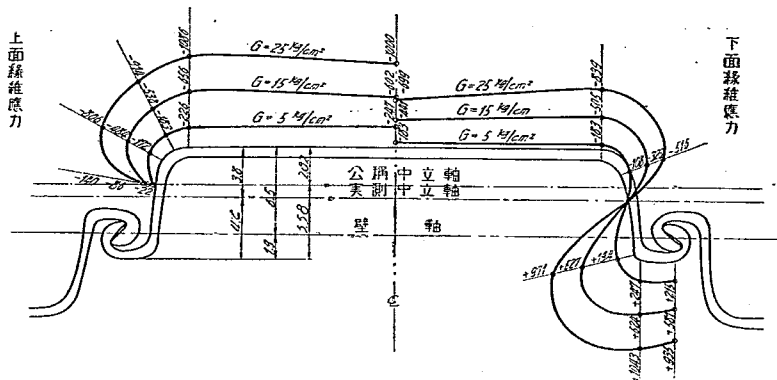
第 6 圖 Larssen 鋼矢板壁抗曲試験縁維應力分布圖 (兩端銲接)
