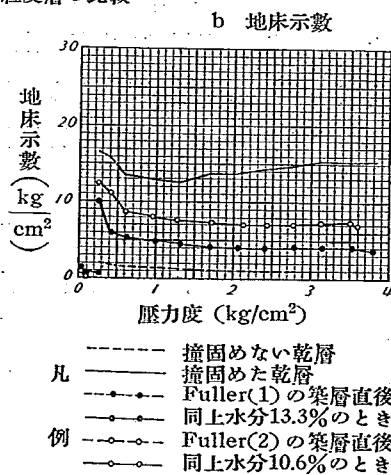
第 20 圖 Fuller 粒度層の比較
