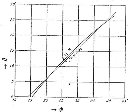
第 21 圖 \phi = 33^\circ の砂に對する計算値
