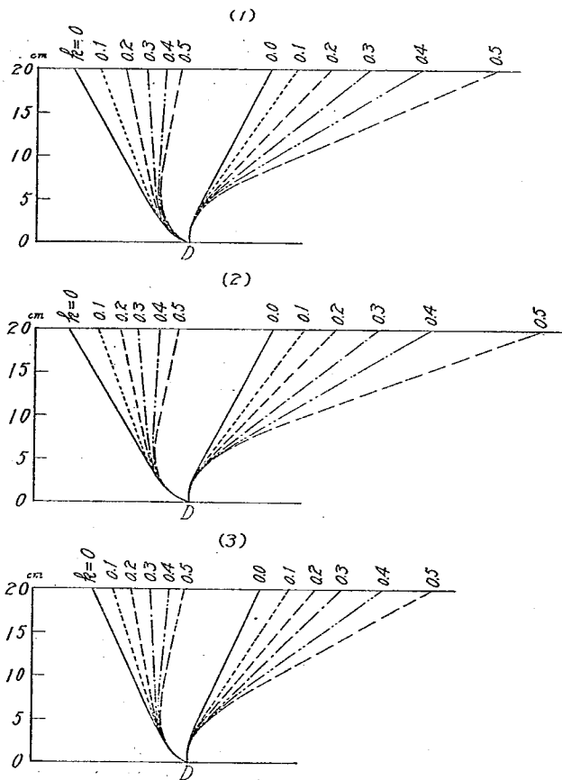
第29圖 種々の傾斜に對する崩壊面計算値 茲に k = \tan \theta
