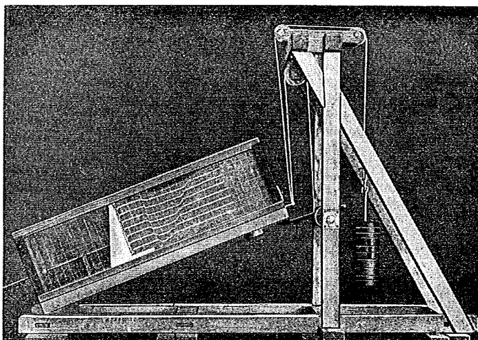
寫真第 2 20 糶試驗函（傾斜狀態）
