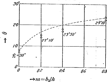
第 16 圖 鎮定材の位置の影響 (40 厘函)
