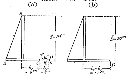
第 19 圖 鎮定材の有無による影響試験の模型 (寫眞第 6 及第 7 参照)
