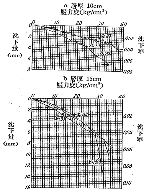
第5圖 単一粒度の砂利層沈下曲線の粒度による比較
