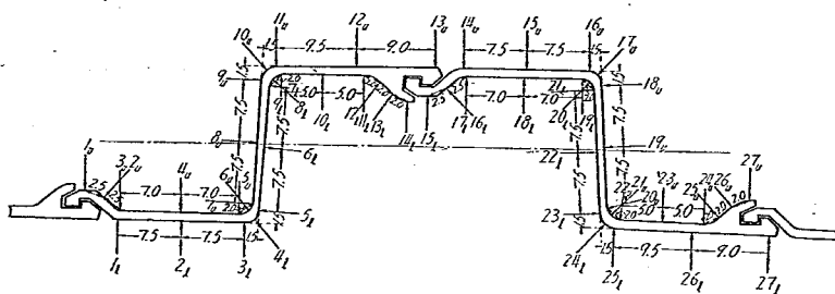
第 7 圖 Hoesch 鋼矢板壁抗曲試驗應力測定點
