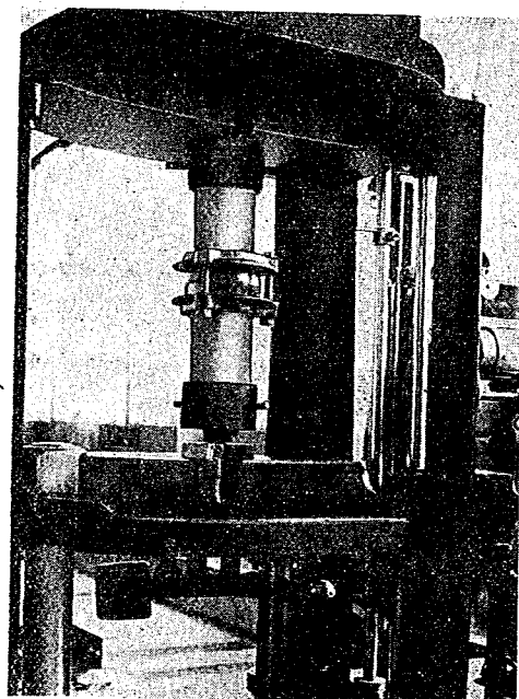
第 20 圖 接手牽引試験
