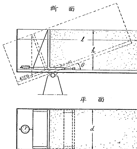
第 7 圖 鎮定材の模型試験装置
