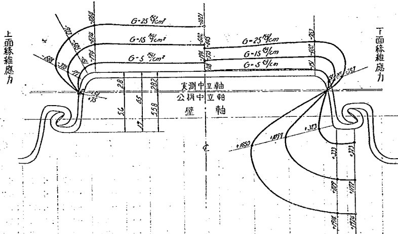
第 4 圖 Larssen 銅矢板壁抗曲試験縁維應力分布圖 (兩端自由)
