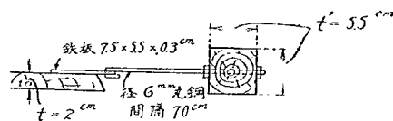
第 11 圖 1.2 米函模型底部詳細断面
