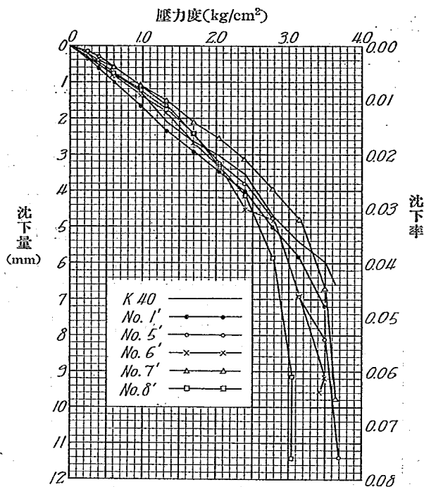
第 13 圖 混合粒度の砂利層の 沈下曲線
