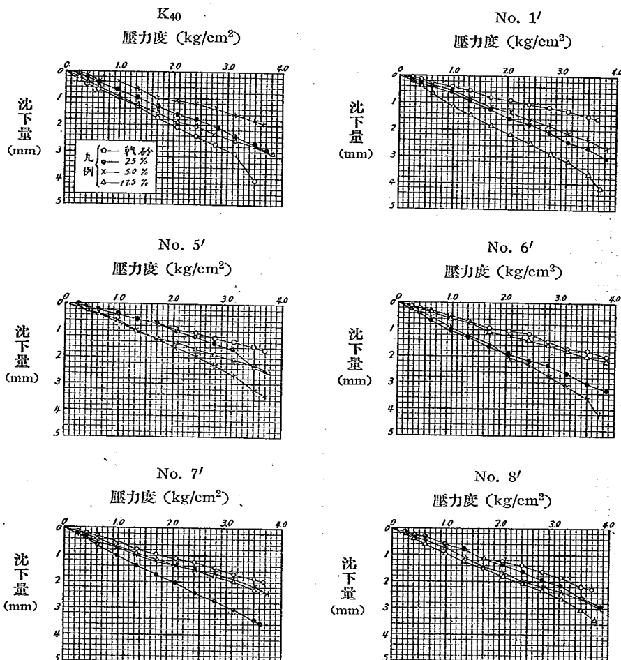
第 17 圖 混砂の含水量と沈下曲線
