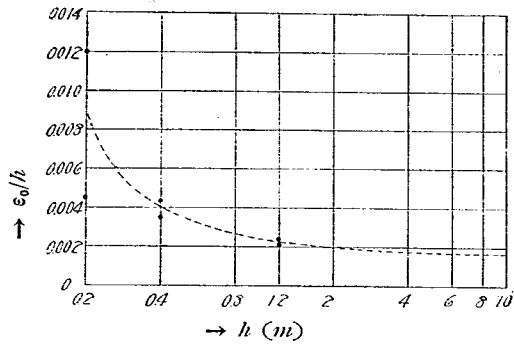
第 20 圖 模型の大きさに依る \varepsilon_0 の變化 ( m=0.2 の場合)
