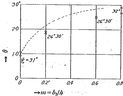
第 17 圖 鎮定材の位置の影響 (1.2 米函)
