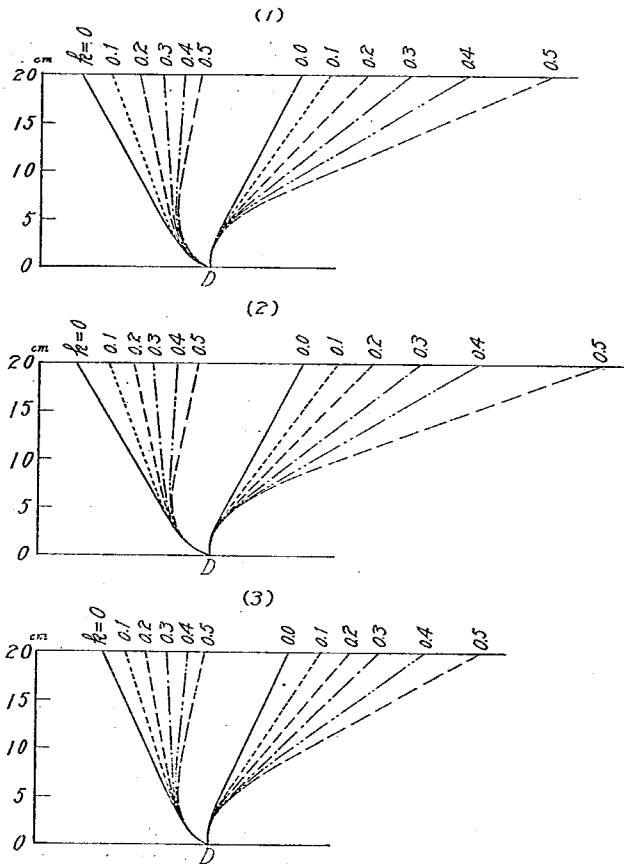
第29圖 種々の傾斜に對する崩壊面計算値 茲に k = \tan \theta (1) \varphi = 32^\circ 40' , \phi_0 = 30^\circ (2) \varphi = 35^\circ , \phi_0 = 30^\circ (3) \varphi = 40^\circ , \phi_0 = 30^\circ
