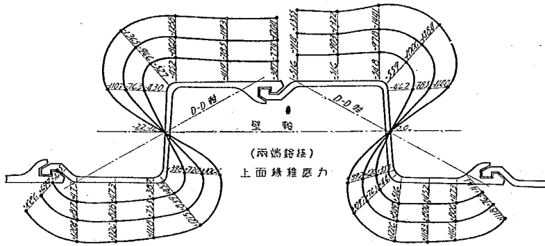
第 12 圖 Hoesch 鋼矢板壁抗曲試験縁維應力分布圖 (其五)
