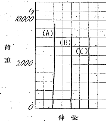
第7圖 抗張試験片荷重伸長曲線
