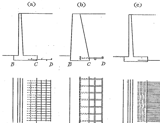
第 23 圖 異形鎮定材
