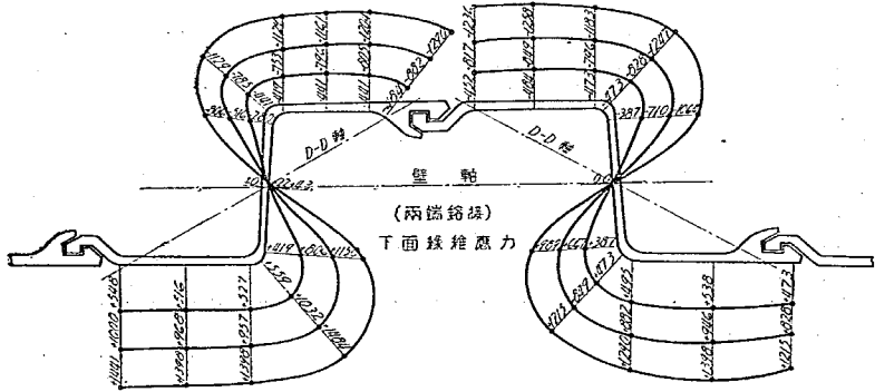
第 13 圖 Hoesch 鋼矢板壁抗曲試験縁維應力分布圖 (其六)
