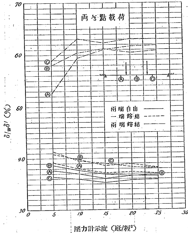
第 1 圖 Larssen Ia 型鋼矢板壁抗曲試験 \delta_w/\delta' 圖表
