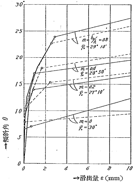
第 14 圖 1.2 米函に於ける滑出試験の結果
