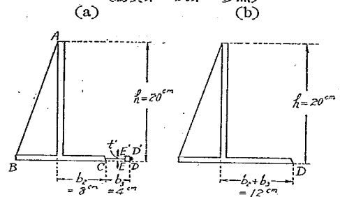
19 圖 鎮定材の有無による影響試験の模型 (寫眞第 6 及第 7 参照)
