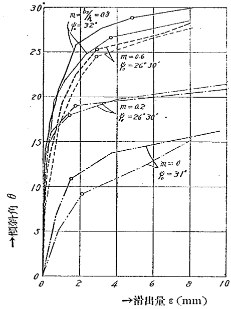
第 14 圖 1.2 米函に於ける滑出試験の結果
