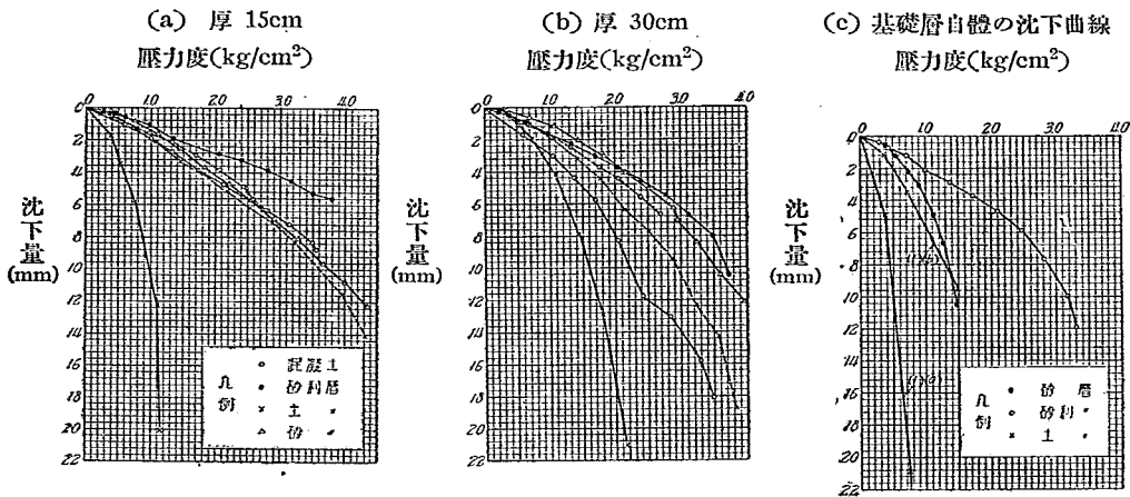
第 25 圖 単一粒度層の沈下曲線の基礎種別に由る比較
