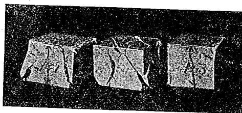
第2圖 A種抗壓試験片破壊状況
