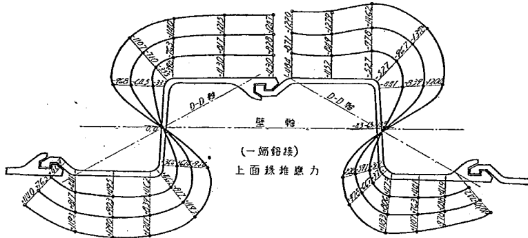
第 10 圖 Hoesch 鋼矢板壁抗曲試驗緣維應力分布圖 (其三)
