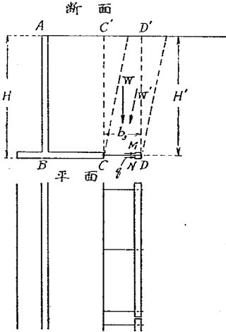
第 31 圖 鎮定材に作用する力の算定
