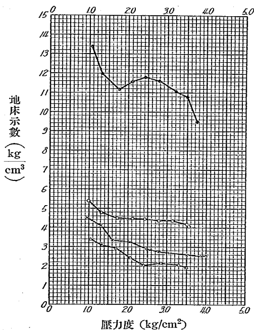
第 9 圖 地床示數の層厚別比較 撞き固めた層 加壓面直徑 20cm
