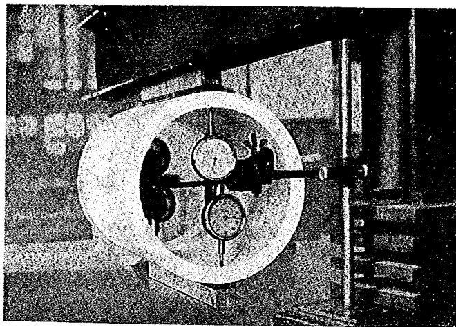
第 15 圖 直徑縮少測定装置
