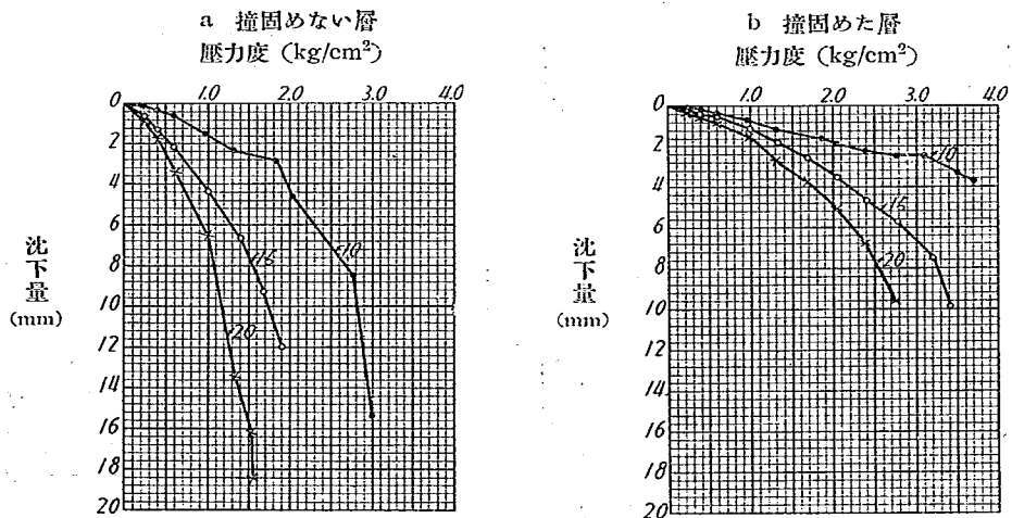
第 3 圖 粒度 20—10mm 砂利層の沈下曲線
