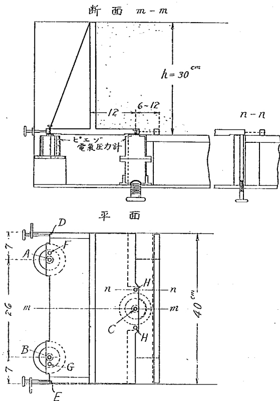
第 25 圖 地盤に及ぼす鉛直力試験装置
