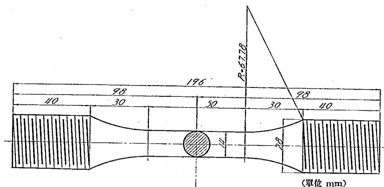
第6圖 抗張試験片
