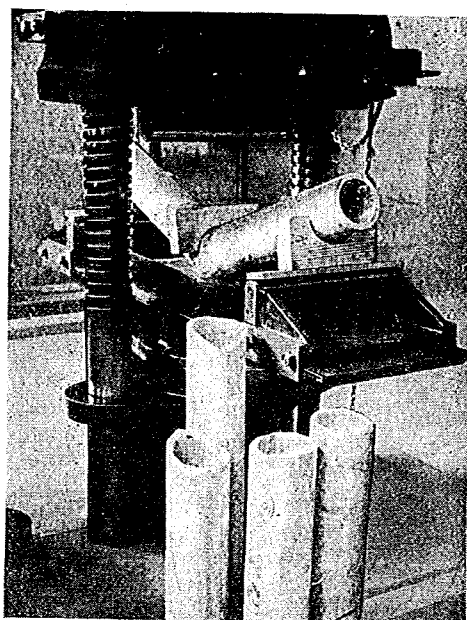
第 12 圖 管體彎折試験
