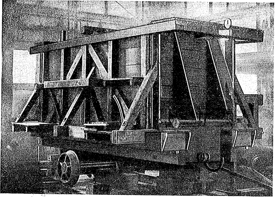
寫真第 4 及第 5 1.2米試驗函
