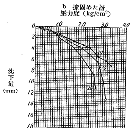
第4圖 粒度 10~5mm 砂利層の沈下曲線
