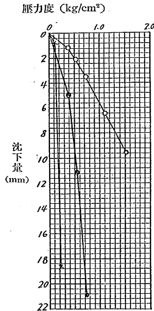
第 21 圖 土層の沈下曲線 厚 15cm, 加壓面直径 20cm
