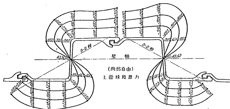
第 8 圖 Hoesch 銅矢板壁抗曲試験縁維應力分布圖 (其一)
