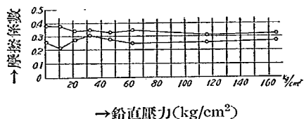
第4圖 鋼鐵と鉛の面の間の摩擦係數測定値
