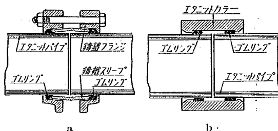
第 19 圖 エタニット・パイプ接手
