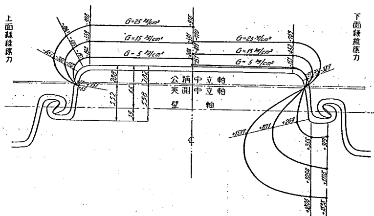
第 5 圖 Larssen 鋼矢板壁抗曲試験縁維應力分布圖 (一端銲接)
