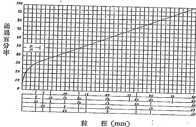
第1圖 Fuller氏砂利最大密度曲線
