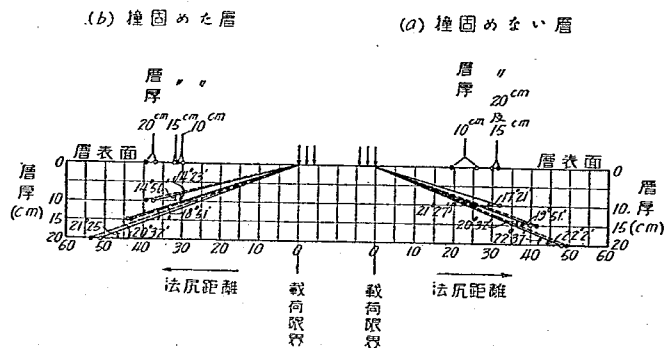
第 12 図 粒度 10—5mm 砂利層の感應距離
