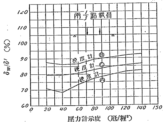
第 2 圖 Hoesch 鋼矢板壁抗曲試験 \delta_w/\delta' 圖表
