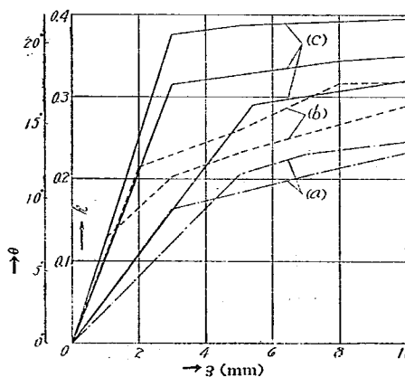
第 27 圖 振動試験に於ける震度と滑出量との關係は何れも鎮定材なしの鎮定材の位置
