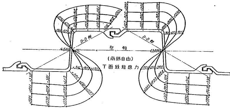
第 9 圖 Hoesch 鋼矢板壁抗曲試驗緣維應力分布圖 (其二)
