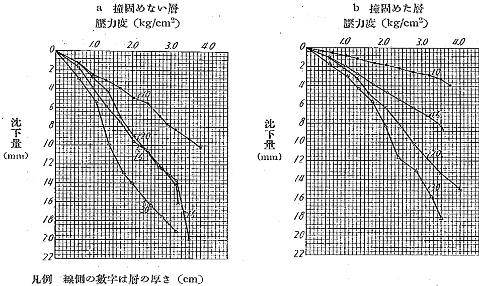
第 2 圖 粒度 40—20mm 砂利層の沈下曲線
