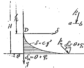
第28圖 箱が傾斜した場合の \delta 變化
