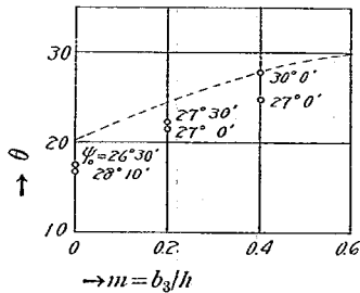
第 17 圖 鎮定材の位置の影響 (1.2 米函)
