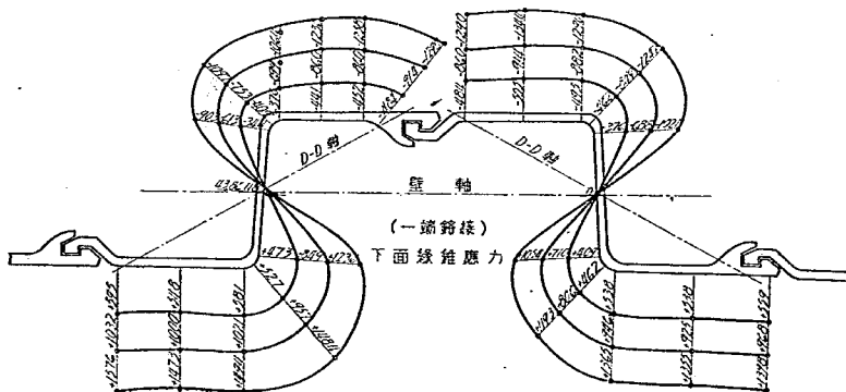
第 11 圖 Hoesch 鋼矢板壁抗曲試驗緣維應力分布圖 (其四)
