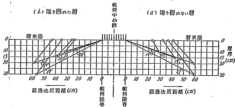
第 10 圖 粒度 40—20cm 砂利層の感應距離
