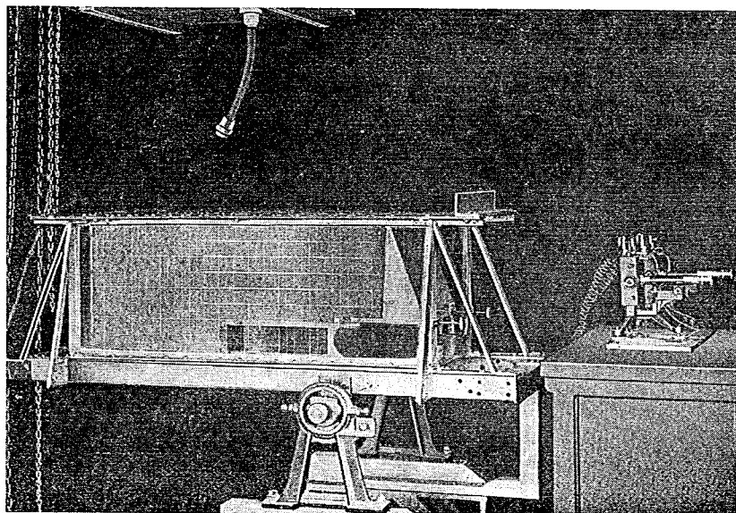
寫眞 第 15 及 第 16 地盤に及ぼす鉛直壓力試験
