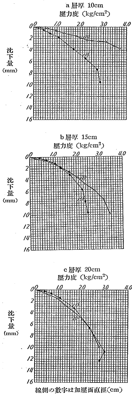
第6圖 粒度 20~10mm 砂利層の沈下曲線の加壓面積に依る比較 法肩距離60cm, 撞固めた層
