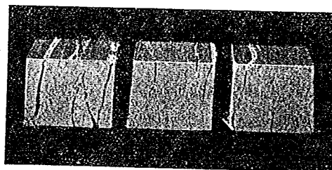
第4圖 C種抗壓試験片破壊状況
