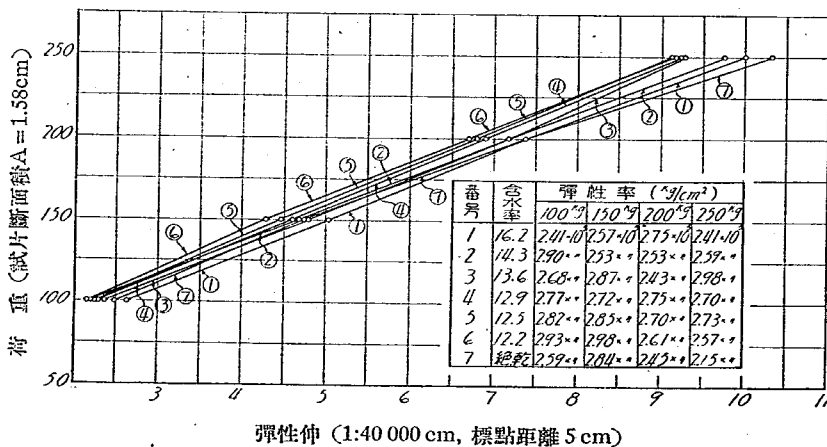
第9圖 含水率の變化と弾性率の關係
