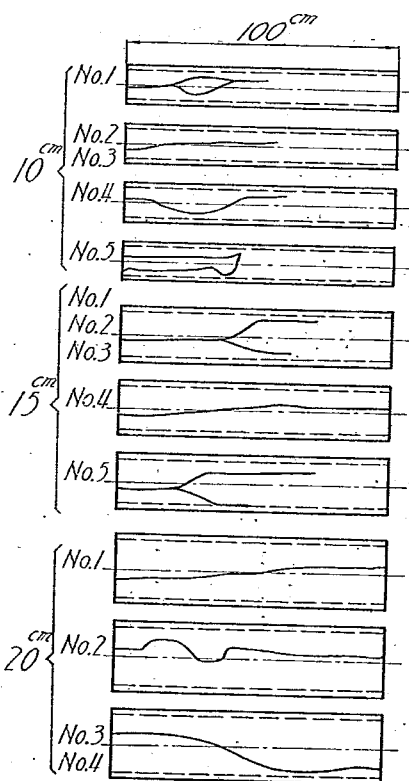
第 18 圖 1 米供試體破壞狀況
