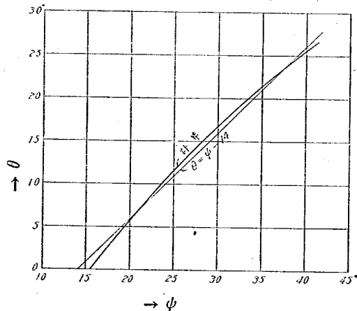
第 21 圖 \phi = 33^\circ の砂に對する計算値
