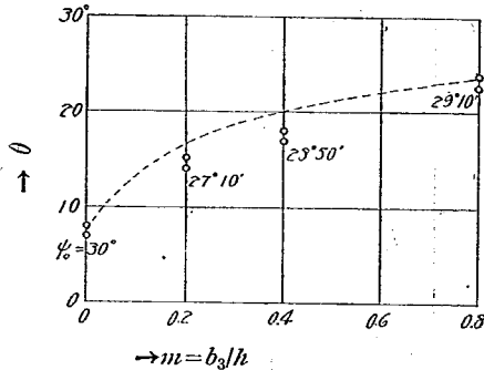
第 16 圖 鎮定材の位置の影響 (40 種函)
