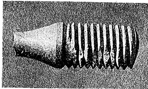
第 1 図 抗張試験片把握部の仕上
