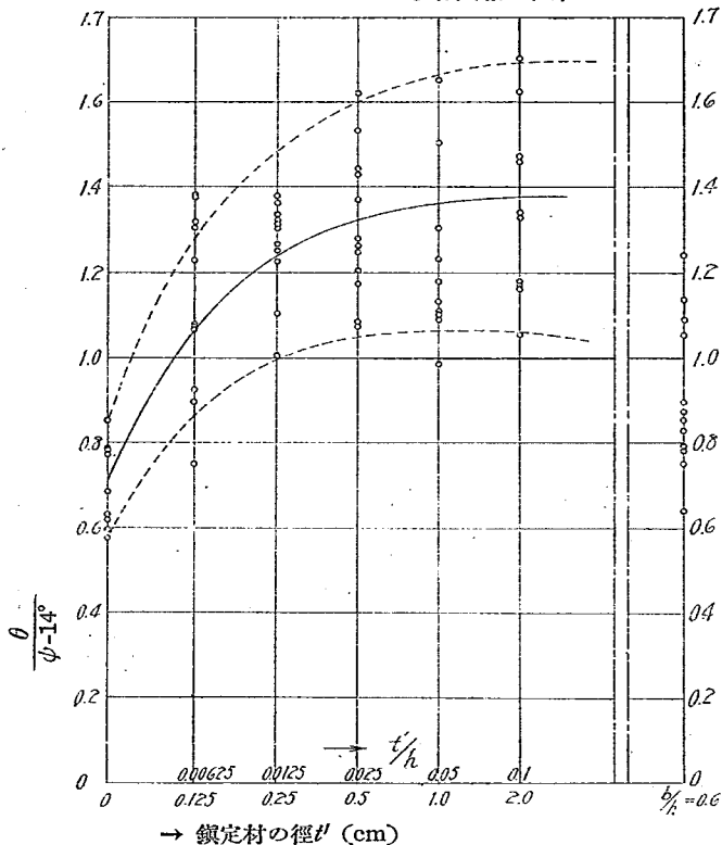
第 22 圖 鎮定材の径の大きさが滑出安定 度に及ぼす影響試験の結果
