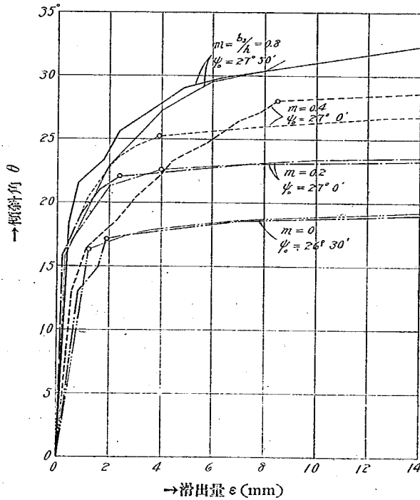
第 14 圖 1.2 米函に於ける滑出試験の結果
