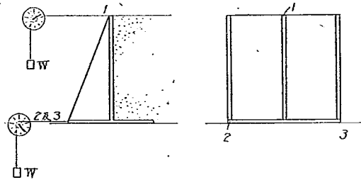
第8圖 1.2 米 試験函の \varepsilon の測點
