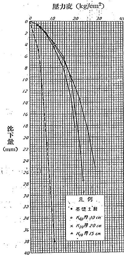
第 23 圖 各粒度最適層の比較
