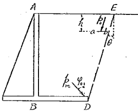
第 30 圖 崩壊面の算定
