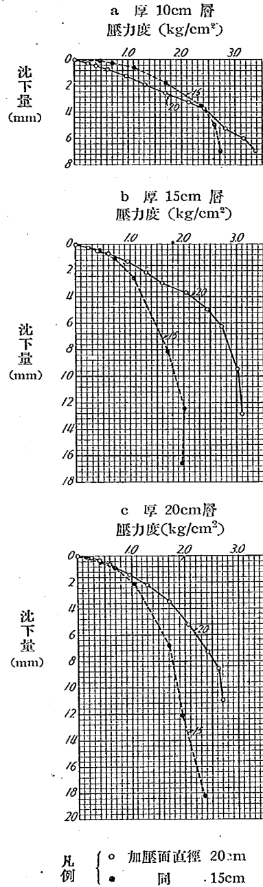
第7圖 粒度 10~5mm 砂利層の沈下曲線の加壓面積に據る比較 撞固めた層, 法肩距離 60cm
