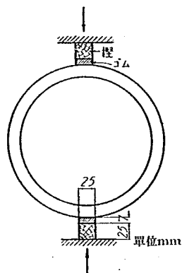
第 13 圖 外壓試験装置
