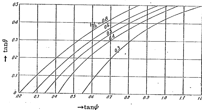
第2圖 滑出安定度の比較
