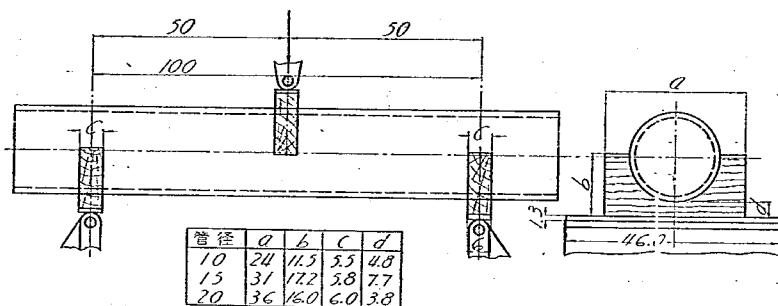
第 10 圖 彎折試験裝置
