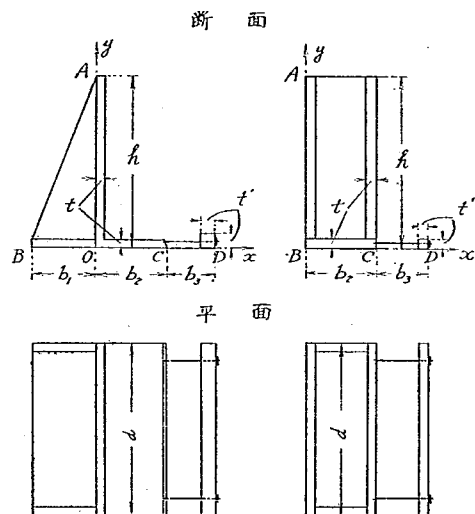
第 10 圖 擁壁模型断面及平面圖
