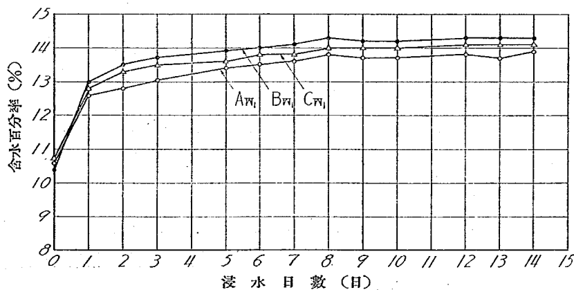
第 5 圖 浸水による含水百分率の増加曲線
