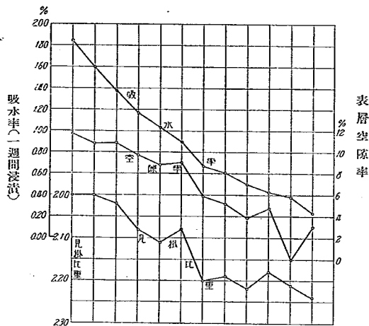
第 5 圖 シート・アスファルト表層の吸水率と空隙率との關係
