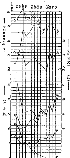
第 5 圖 シート・アスファルト表層の吸水率と空隙率との關係
