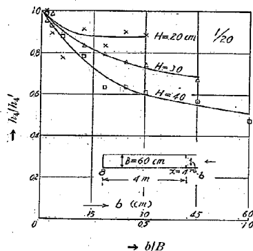
第 41 圖 同上底面勾配 1/20 の場合
