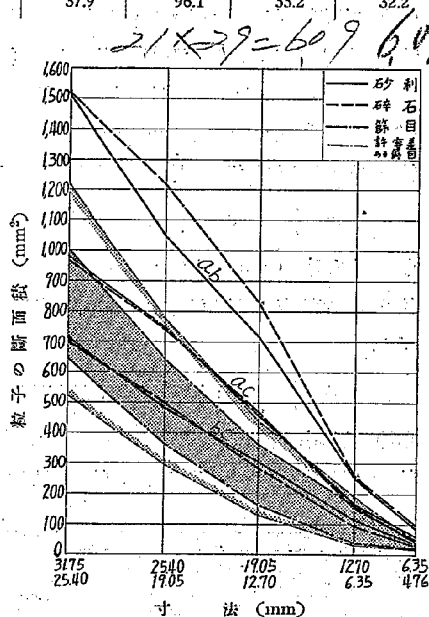
第 14 圖 粒子の断面面積と篩目面積との比較
