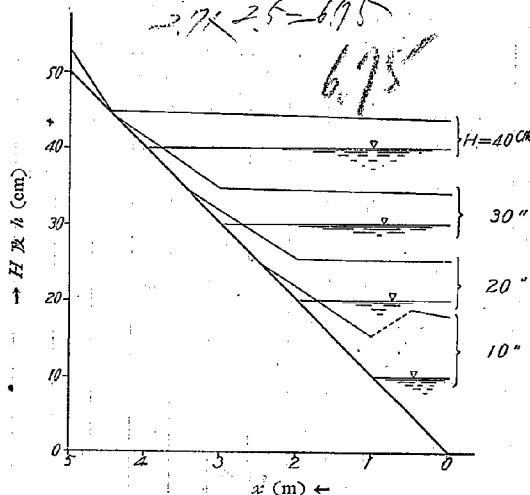
第 22 圖 底面勾配 1/10 の水路上を 波が走る場合の波形の變化
