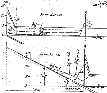
第 36 圖 開口を有する阻壁を A なる位置に鉛直に立てた場合の波の頂の軌跡
