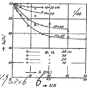
第 40 圖. 開口を有する阻壁位置に於ける高さと同じ位置に開口を有しない阻壁を有した場合の高さとの比 b/B との關係 底面勾配 1/40 の場合
