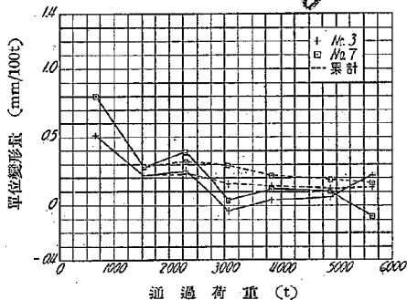
第 8 図 鐵輪帶に由る變形量に基く工法の比較
