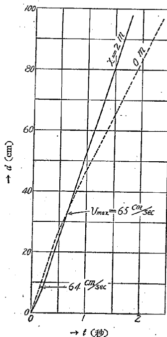
第17図 同上, 水深 10cm, 底面勾配 1/40
