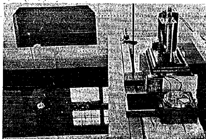
第2圖 波形観測の装置 (其一)
