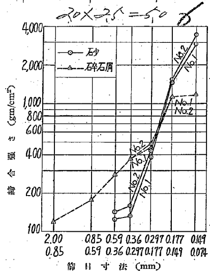
第 36 圖 砂及碎石屑の縮合強さ
