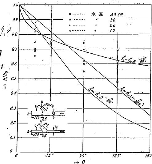
第 45 圖 波の進む方向と \theta なる角をなす灣内に於ける波高と \theta との關係。太い實線は茲に得た實驗式細い實線は廣井博士の式
