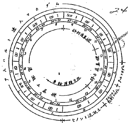
第 2 圖 試験路面配置
