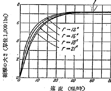
(3) 複式バルン・タイヤ (障害物の高さ 1.5")
