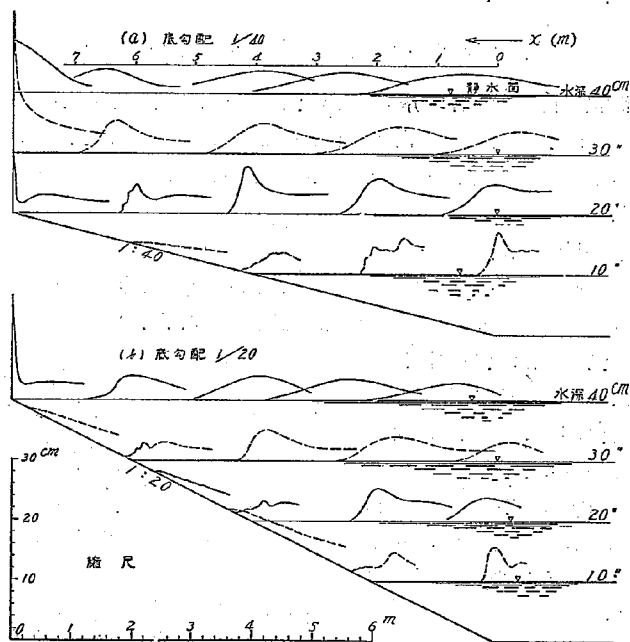
第 9 圖 1/40 及 1/20 の底面勾配上を波が走る場合の波形の變化 (本組終の寫眞第 1 乃至第 4 参照)
