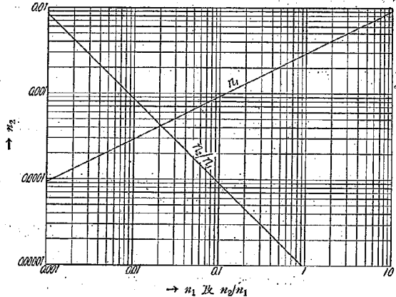
第 27 圖 波形の相似律が成立つ爲の n_1 と n_2 との関係。茲に模型の鉛直方向の縮尺を實物の n_1 倍、水平方向の縮尺を n_2 倍とする。
