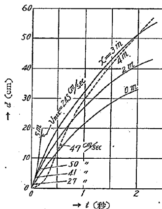
第16図 同上, 水深 20cm 底面勾配 1/40
