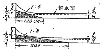
第 25 圖、水路底面が急勾配をなす場合の試験
