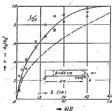
第 39 圖 同上 底面勾配 1/20 の場合
