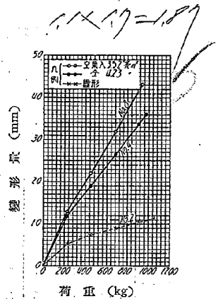
第 6 圖 輪帶の荷重と變形量
