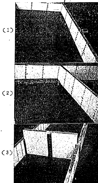
写真 第 10 開口を有する阻壁試験 1/40 勾配 水深 H=40\text{cm}
