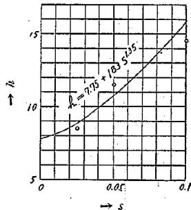
第 24 圖 底面勾配と波が達する高さとの関係
