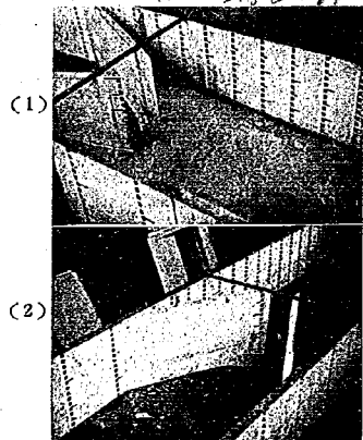
写真 第 13 八字形阻壁試験 1/40 勾配 水深 H=30\text{cm}
