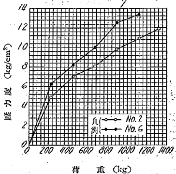
第 5 圖 輪帶の荷重と壓力度
