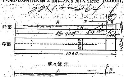
第1圖 試験用水槽
