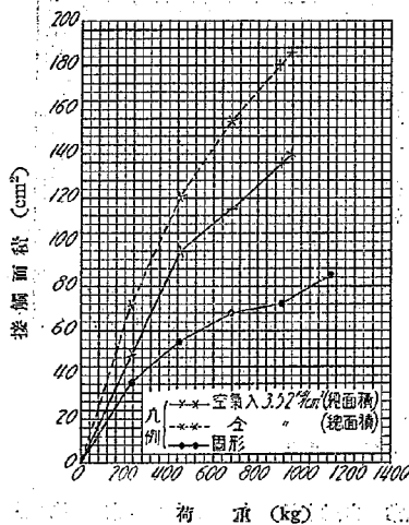
第 4 図 輪帯の荷重と接觸面積
