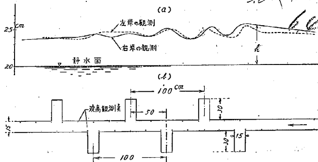
第 46 圖 特殊なる防波装置
