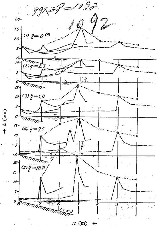
第 29 圖 阻壁試験
