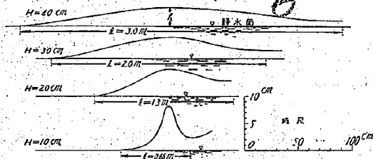
第6図 底面水平なる水路内に於ける波形(第1図参照) l_2=100\text{cm} , h''=10\text{cm} なる場合の水深 H=40, 30, 20, 10\text{cm} に於ける波
