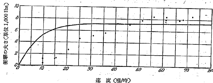
(4) 單式バルン・タイヤ (障害物の高さ 1.5")
