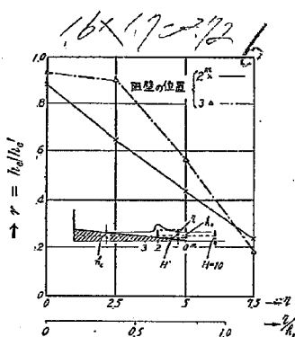
第 33 図 阻壁の水面上の高さの影響。 底面勾配 1/40, 水深 10cm
