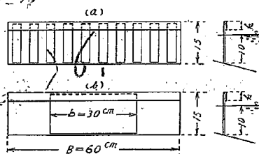
第 43 圖 特殊阻壁(a)と普通の開口を有する阻壁(b)
