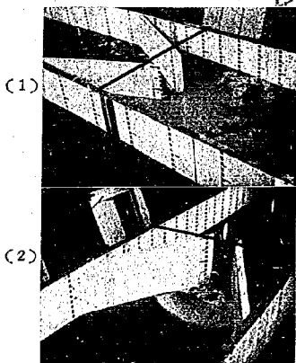
写真 第 12 八字形阻壁試験 1/40 勾配 水深 H=40\text{cm}
