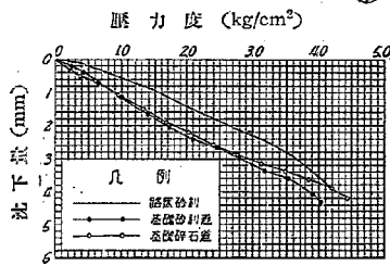
(b) 基礎碎石道
