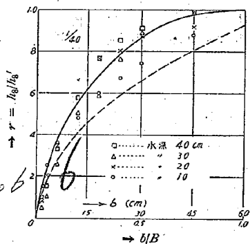
第 38 圖 同上 底面勾配 1/40 の場合
