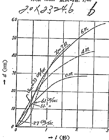
第14図 最初の各相富値所に水面上においた小浮子が波の進行と共に水平方向に變位する状態を活動寫眞(毎秒 64 齣のもの)に依り撮影した結果より得た時間 t と水平方向の變位 s との関係曲線 t=0 は撮影開始の時間で小浮子が運動を始めた時間と略一致する。
