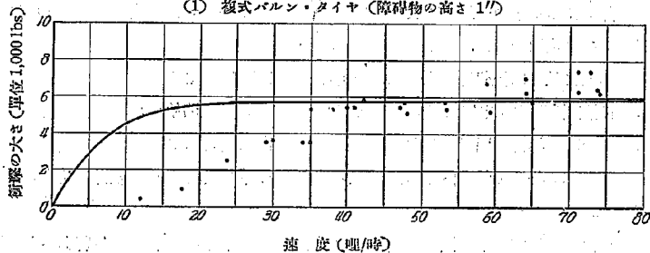
(1) 複式バルン・タイヤ (障害物の高さ 1")
