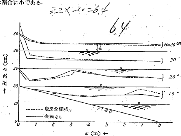
第 26 圖 水路底面の影響を見る爲に底面に一樣に金網を張つた状態で試験し、張らない場合の波形との変化と比較する
