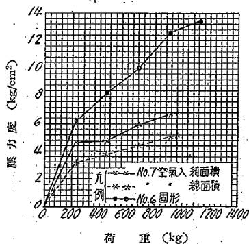
第 5 圖 輪帶の荷重と壓力度
