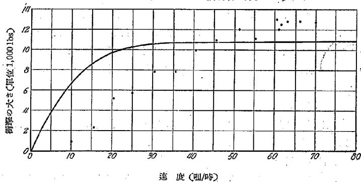
(3) 單式バルン・タイヤ (障害物の高さ 1")
