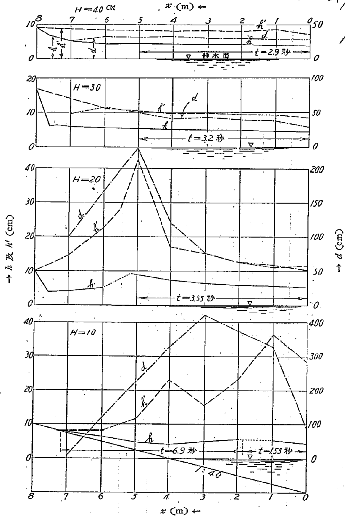
第 10 図 1/40 の底面勾配の水路上に於ける観測の結果
