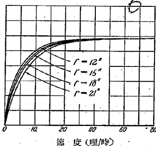
(4) 單式バルン・タイヤ (障害物の高さ 1.5")
