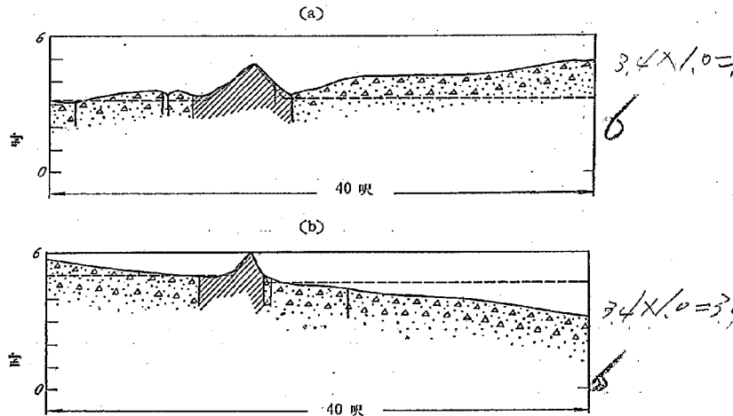
第 27 圖 自然路面の凹凸の形狀 —— 路面の形狀 ----- 計算に用ひた假想路面
