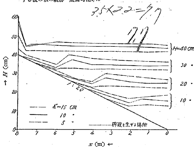
第 13 図 同上、底面勾配 1/20
