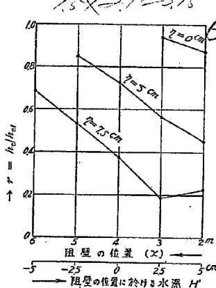
第 34 図 阻壁の位置の影響 底面勾配 1/40, 水深 10cm
