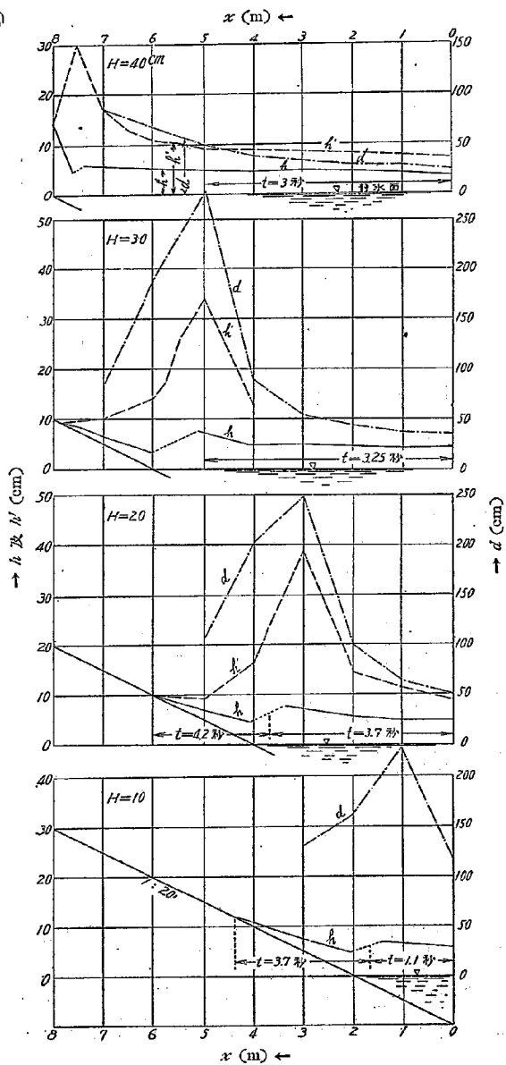
第 11 圖 1/20 の底面勾配の水路上に於ける観測の結果, 記號はすべて第 10 圖と同様
