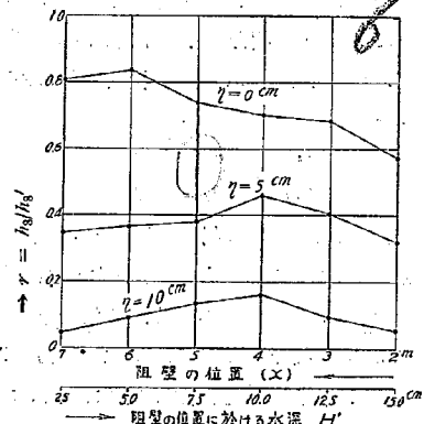
第32図 阻壁の位置の影響
