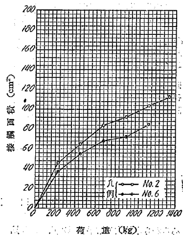
第 4 図 輪帶の荷重と接觸面積
