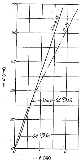
第17図 同上, 水深 10cm, 底面勾配 1/40
