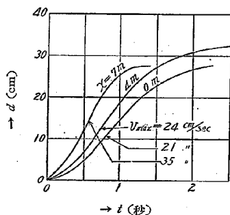
第14図 最初の各相富値所に水面上においた小浮子が波の進行と共に水平方向に變位する状態を活動寫眞(毎秒 64 齣のもの)に依り撮影した結果より得た時間 t と水平方向の變位 s との関係曲線 t=0 は撮影開始の時間で小浮子が運動を始めた時間と略一致する。
