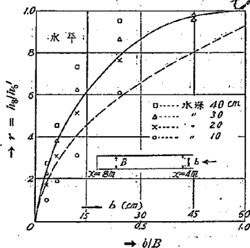
第 37 圖 開口を有する阻壁試験の結果。 開口の幅 b の内部の波の高さに及ぼす影響。 x は全然壁のない場合の x=8m に於ける値と b なる幅の開口を有する壁を立てた場合の同じ場所の値との比 實線はこの実験の近似式
