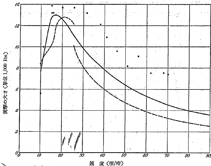
矩形障碍物の drop の値 (高さ 1.5") 複式バルン・タイヤ
