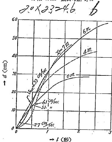
第15図 同上, 水深 30cm, 底面勾配 1/40
