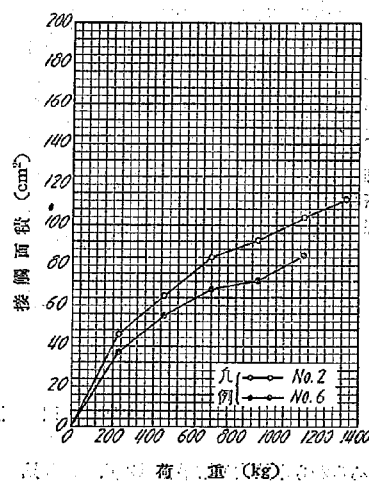
第 4 図 輪帶の荷重と接觸面積
