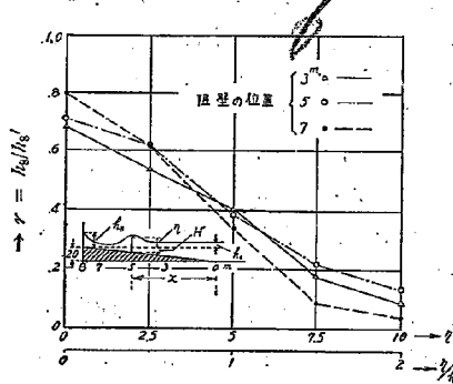
第 31 図 阻壁の水面上の高さの影響 x=8 m に於ける高さ h_0 と阻壁のない場合 の高さ h_0' との比 r をとり之と \eta との関 係を示す。
