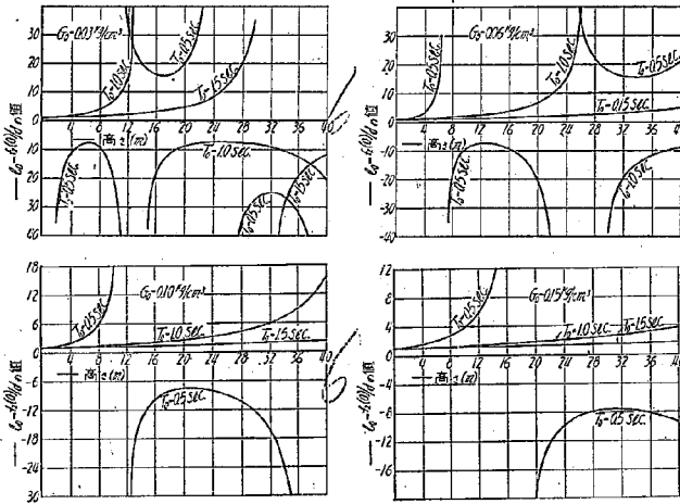
第 9 圖 強制振動による頭部の變形 (剛性係数が一定に比例する場合)
