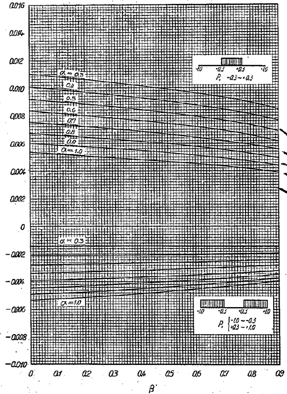
第 36 圖 鉛直等布部分荷重 拱頂彎曲率 M_c
