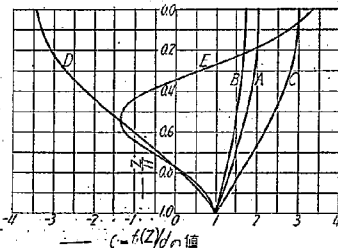
第 8 図 中立軸の變形曲線 (G が深さに無関係の場合)
