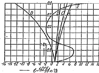
第 10 圖 中立軸の變形曲線 (剛性係数が一定に比例する場合)
