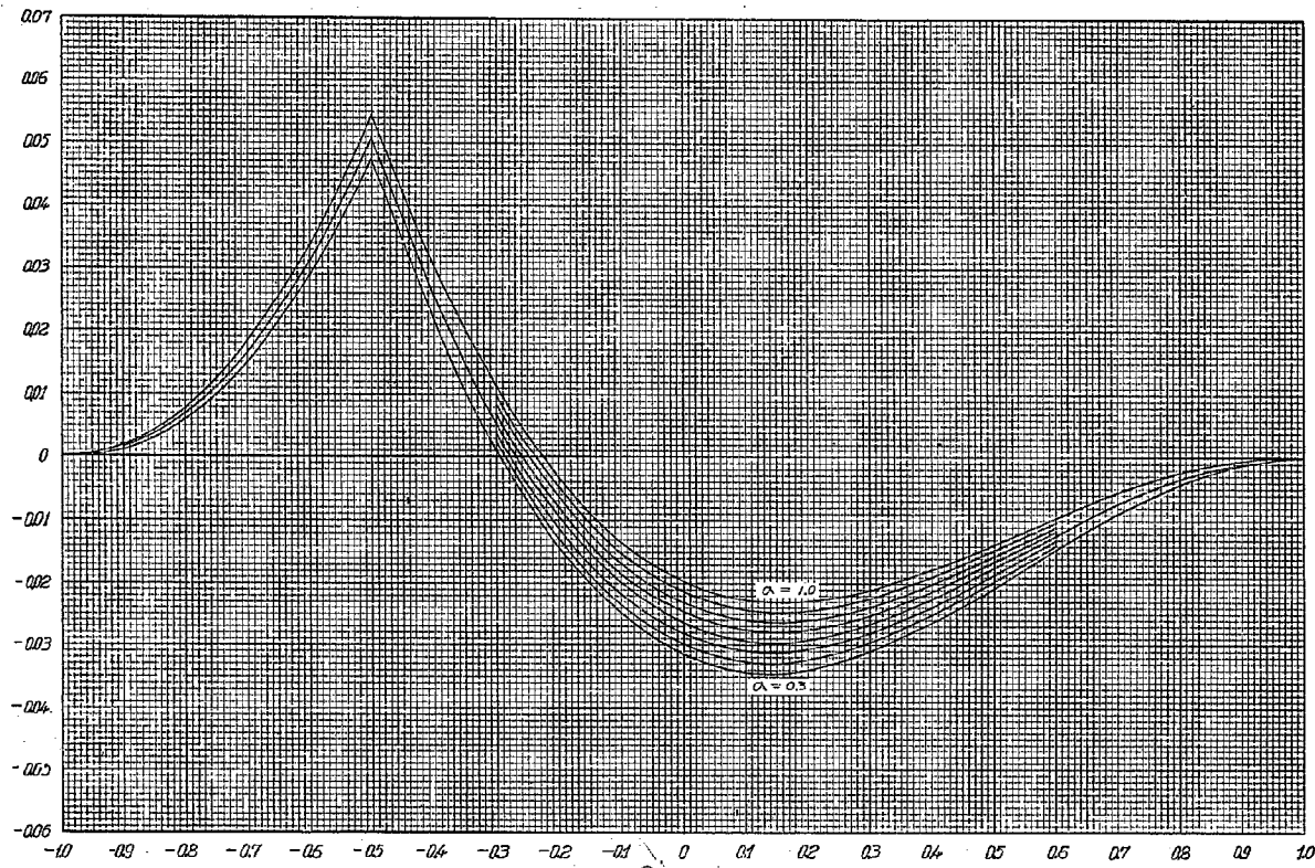
第 18 圖 鉛直荷重 1/4 波彎曲率影響線 M/H ( \beta=0.6 \alpha=1.0, 0.9, 0.8, 0.7, 0.6, 0.5, 0.4, 0.3 )
