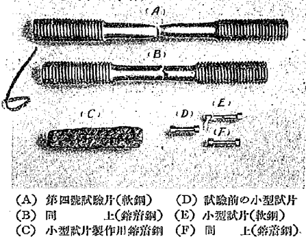
第 11 圖 第四號試片と小型試験片
