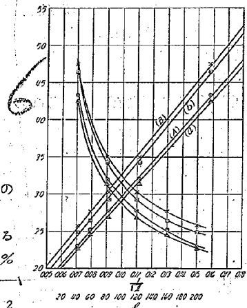
第 8 圖 \varphi と l との關係
