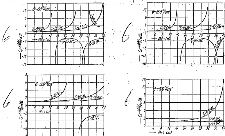
第 7 図 強制振動による頭部の變形 (剛性係数が深さに無関係の場合)
