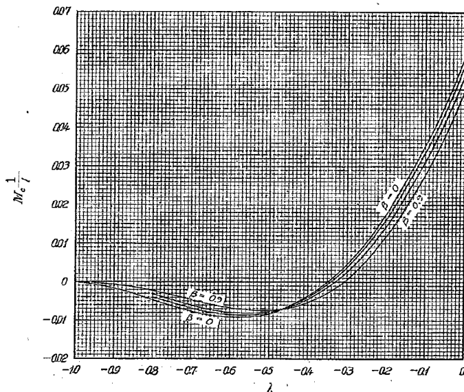
第 19 圖 鉛直荷重 拱頂彎曲率影響線 M_c ( \alpha=0.6 \beta=0, 0.3, 0.6, 0.9 )
