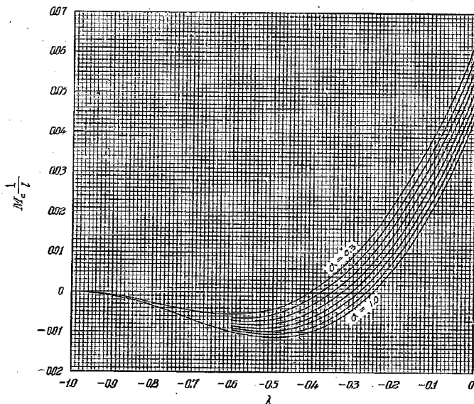
第 20 圖 鉛直荷重 拱頂彎曲率影響線 M_c ( \beta=0.6 \alpha=1.0, 0.9, 0.8, 0.7, 0.6, 0.5, 0.4, 0.3 )
