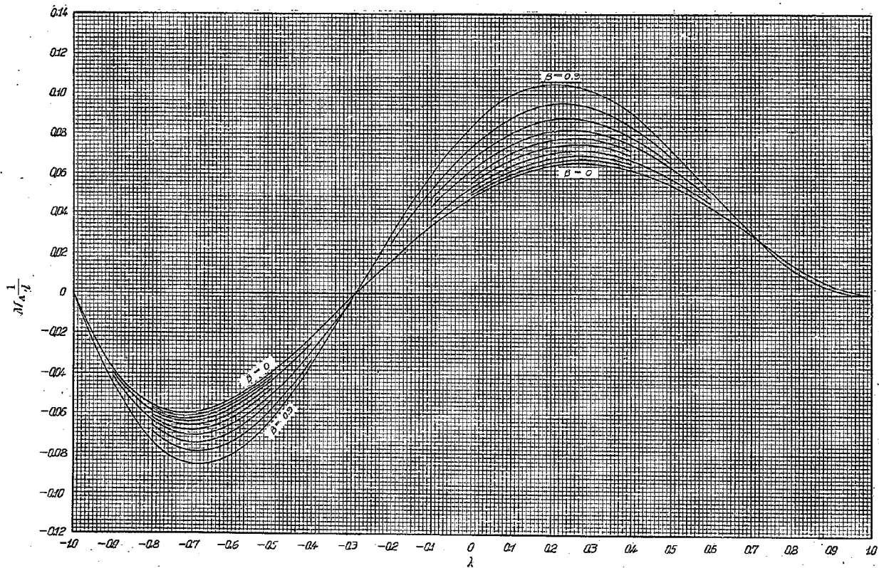
第 15 圖 鉛直荷重 起拱點彎曲率影響線 M_A ( \alpha=0.6 \beta=0, 0.1, 0.2, 0.3, 0.4, 0.5, 0.6, 0.7, 0.8, 0.9 )
