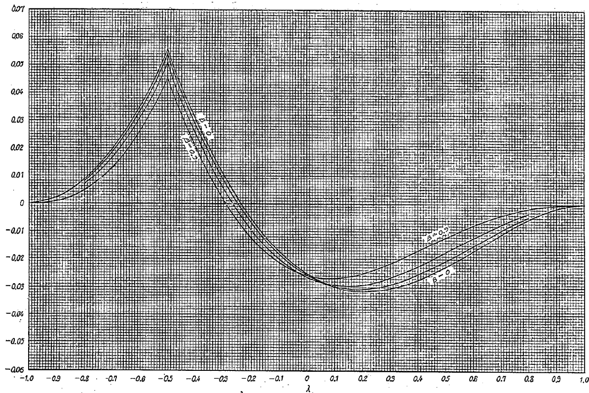
第 17 圖 鉛直荷重 1/4 點彎曲率影響線 M/M_u ( a=0.6 \beta=0, 0.3, 0.6, 0.9 )
