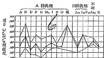
試料 第3圖 4°/25°C 比粘度の比
