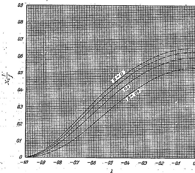
第 23 圖 水平荷重 鉛直反力影響線 X_2 = A ( \alpha = 0.6 \beta = 0, 0.3, 0.6, 0.9 )
