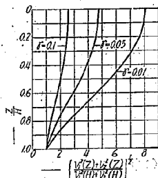
第 12 圖 共振時の各高さの最大變位 ( G, \eta 高さに無関係の場合)
