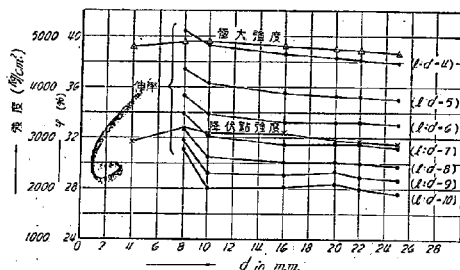
第6圖 l:d の増加に伴ふ極大強度降伏強並に \varphi の變化
