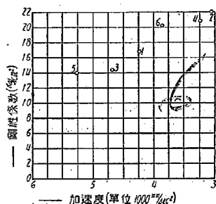
第 44 圖 生形砂と砂との混合物の剛性係數
