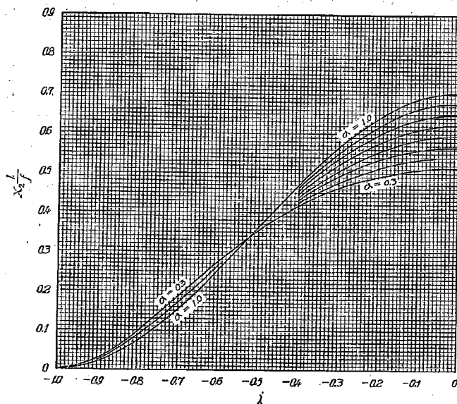
第 24 圖 水平荷重 鉛直反力影響線 X_2 = A ( \beta = 0.6 \alpha = 1.0, 0.9, 0.8, 0.7, 0.6, 0.5, 0.4, 0.3 )
