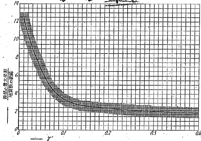
第 13 圖 共振時の頭部の最大變形 ( G, \gamma が深さに比例する場合)
