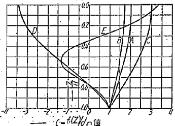
第 8 圖 中立軸の變形曲線 ( G が深さに比例する場合)
