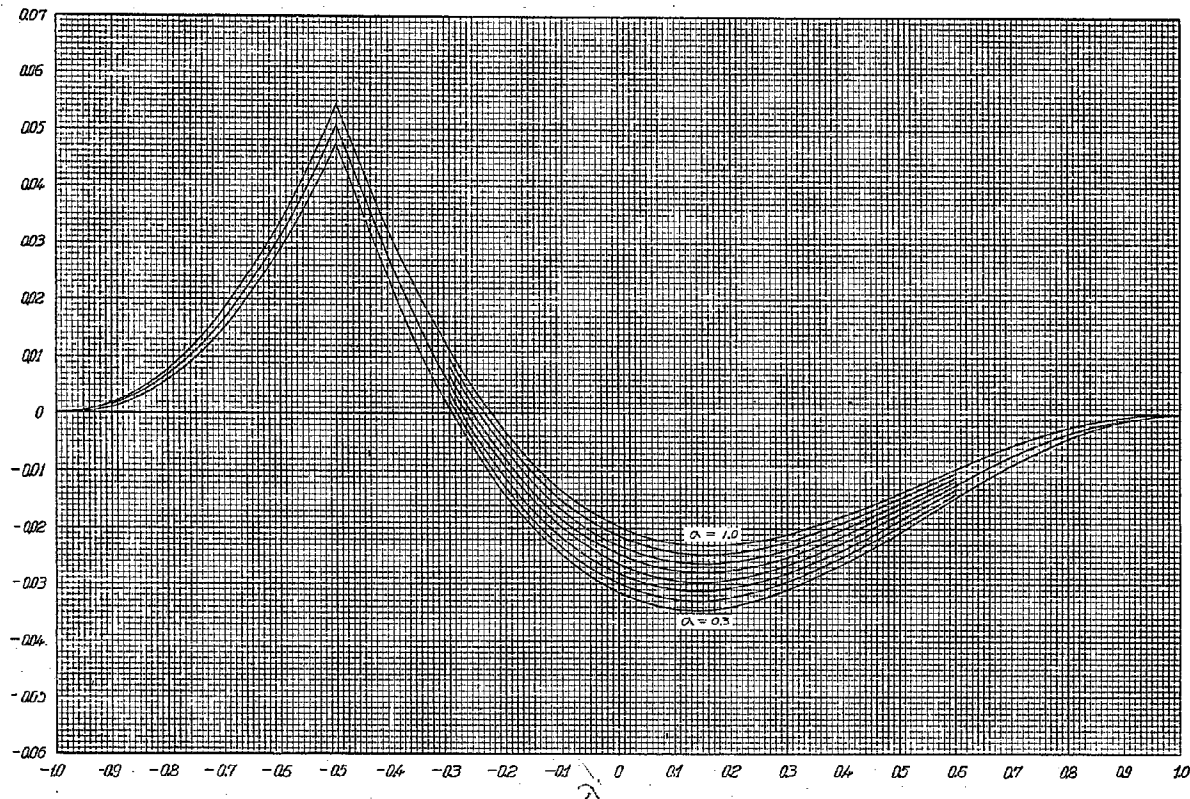
第 18 圖 鉛直荷重 1/4 點彎曲率影響線 M/M_1 ( \beta=0.6 a=1.0, 0.9, 0.8, 0.7, 0.6, 0.5, 0.4, 0.3 )
