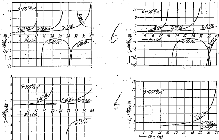
第 7 図 強制振動による頭部の變形 (剛性係数が深さに無関係の場合)
