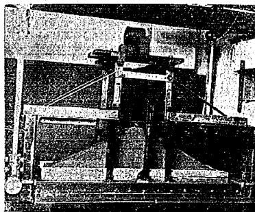
第 37 圖 頭部の變位測定裝置
