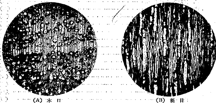
第2圖 Kapor 材の組織 (倍率約 25)
