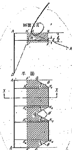
第 32 図 控版が壁に接近して深い位置にある場合の圖。
