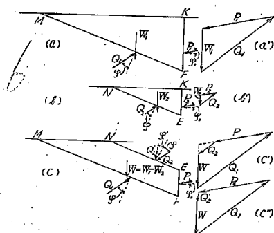
第2圖 控版 EF に働く力の平衡状態
