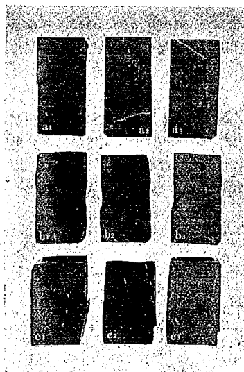
第 12 圖 壓縮試験片(乙) 炭塊状況-ターペンタイン材(氣乾)
