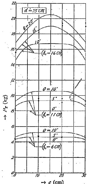
第 23 圖 同上 d=35 cm の場合
