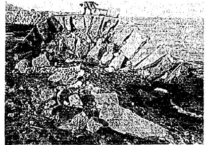
第 18 圖 淡路島東岸鹽田村防波堤の一部決壊せる部分
