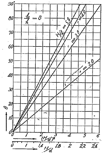
第37圖 同上 h_1/h=8 の場合。
