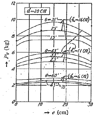
第 21 圖 同上 d=20 cm の場合
