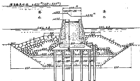
第 15 圖 木津川口新防波堤断面。津浪による被害はない
