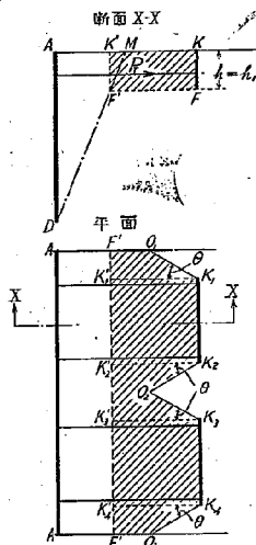
第 6 圖 控版が連続版でない場合の新計算法 (控版の位置が壁に接近して置かれてある場合)
