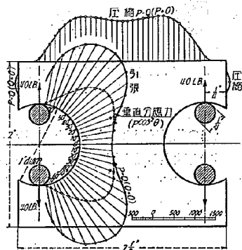
第16圖 引張試片の緣應力分布圖 (E. G. Coker)
