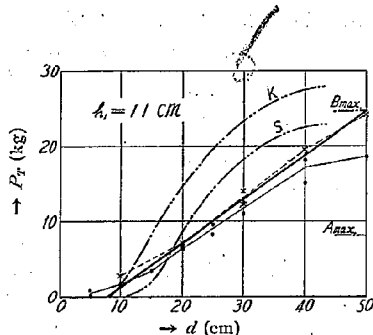
第 13 圖 同上 h_1 = 11 cm
