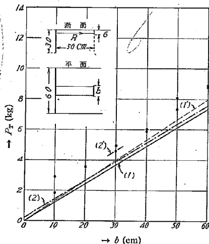
第 39 圖 擁壁から十分遠方にある控版の支持力が兩側の土砂より受くる影響試験の結果。(1)は兩側の影響を考へない場合の計算値、(2)は從來普通に行はれてゐる本文(5)式(第 I 章(2))による兩側の影響を之に加へたもの、(1')は安藤博士の計算法による兩側を考へない場合の計算値、(2')は h/3 の幅だけ版の長さが兩側に大になつたとした場合の計算値。
