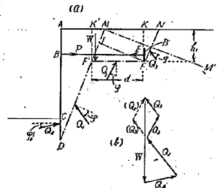
第 5 圖 新しく提案した計算法に依る力の平衡状態 (控版が壁に接近して置かれてある場合)
