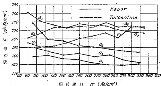
第 27 圖 壓縮による E と應力強度との關係 (其一)
