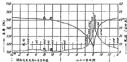
第 2 圖 府立大阪測候所に於ける気壓、風速及風向、風速は 21 日 午前 8 時～9 時の間測定値がないから破線にて結ぶ
