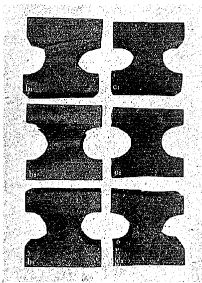
第 17 圖 引張試験片切断状況 カポール村(氣乾)
