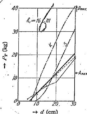
第 14 圖 同上 h_1 = 16 cm
