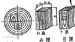
第 4 圖 收縮率測定試片製作用材
