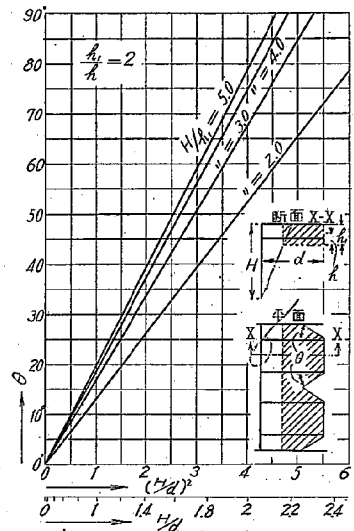
第35圖 第27圖及第33圖の試験結果より得たる H/d と \theta との関係、 h_1/h=2 の場合。
