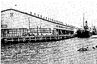
第 22 圖 大阪港第 7 號繫船岸上屋壁鐵骨にモルタルスレートを張つた構造であつたがスレートは漂流物の爲に寫眞の如く破損して落ちた。(9 月 27 日撮)
