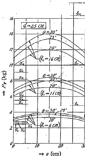
第 22 圖 同上 d=25 cm の場合
