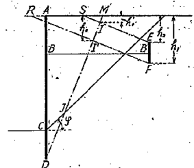
第 4 圖 控版が壁に接近して置かれてある場合の力の平衡状態
