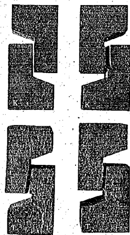
第 22 圖 剪断試片破壊狀況 (K—カボル材)(T—ターペンタイン材)
