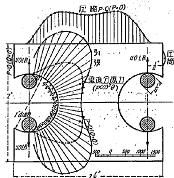
第16圖 引張試片の縁應力分布圖 (E. G. Coker)
