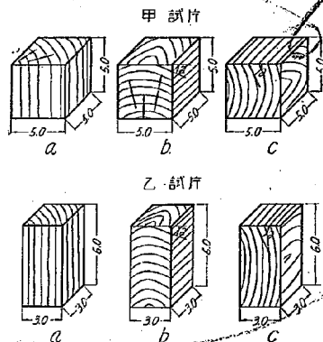
第6圖 壓縮試験片
