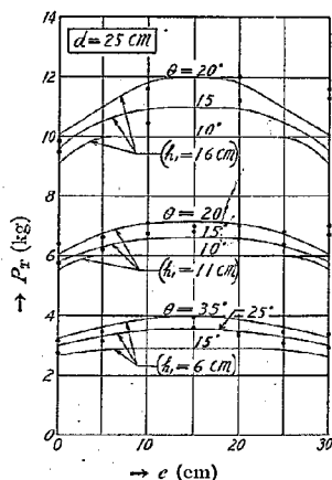
第 30 図 連続版でない控版が深い位置にある場合の版の間隔 c との影響試験の結果。記入の曲線は第 32 図に於て斜線を施した部分の砂が控版の支持力に影響するとして算式 (4) により \theta の種々の値に對する P_z を示す。 d=25 cm
