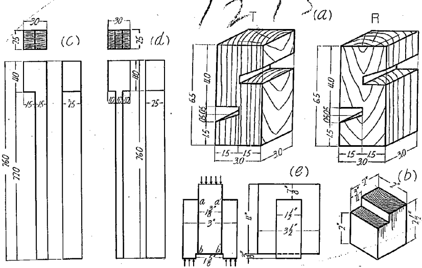
第 20 圖 剪断試験片
