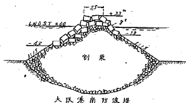
第 11 圖 大阪港南防波堤斷面
