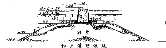
第 16 圖 神戸港南防波堤断面。津浪により頭部が約 15cm 港内へ移動した
