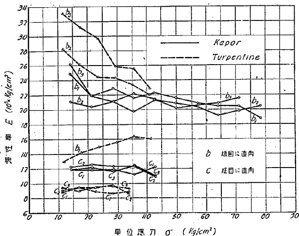
第 28 圖 壓縮による E と應力強度との關係 (其二)
