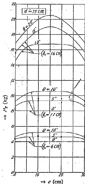
第 23 圖 同上 d=35 cm の場合
