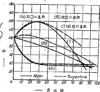
第 13 圖 壓縮強と含水率との關係
