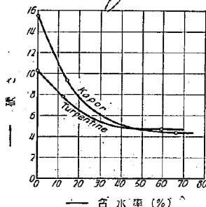
第 24 圖 硬さと含水率との關係
