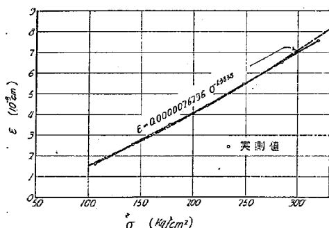
第 29 図 Kapur a 3 試片につきて E と \sigma との関係
