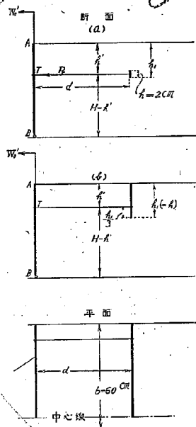
第 11 圖 控版模型試験の二つの場合
