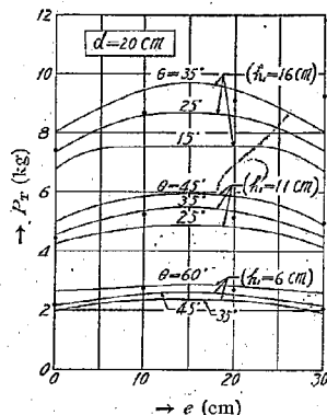
第 21 圖 同上 d=20 cm の場合
