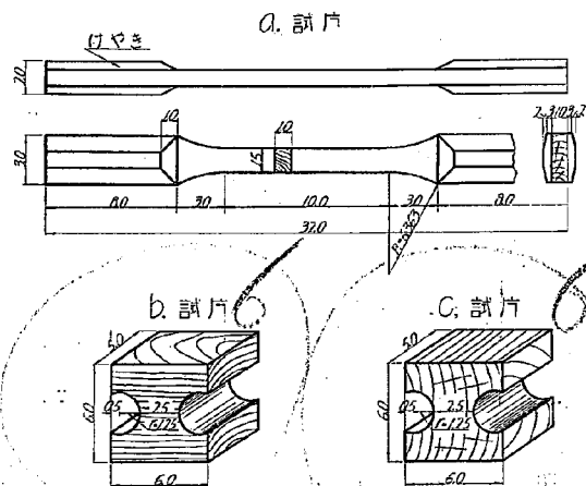
第14圖 引張試験片
