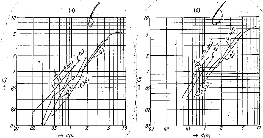
第 17 圖 控版に作用する力を P_0 = \frac{1}{2} C_0 \gamma h_1^2 とし C_0 と d/h_1 との關係を h_1/H の種々の場合に就て示す。第 12~16 圖の試験結果による。(a) は第 11 圖 A の場合。(b) は第 11 圖 B の場合。
