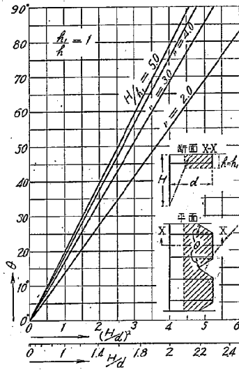
第34圖 第27圖の試験結果より得たる h_1/h=1 の場合の H/d と \theta との関係。
