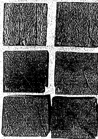
第 8 圖 壓縮試験片(甲)破壊状況—ターペン タイン材(絶對乾燥)
