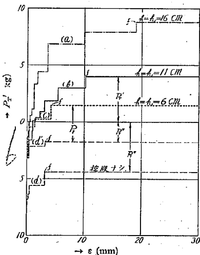
第 10 圖 控版に加はる力 P_T' と壁の頂 A の水平移動量との關係
