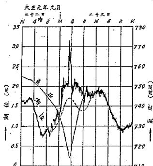
第 10 圖 大正元年 9 月 23 日の 大阪に於ける暴風津浪の築港内 に於ける檢潮儀記錄
