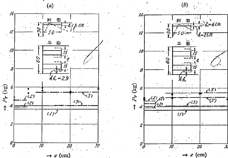
第 40 図 間隔 e を隔てて置いた二枚の控版による試験により第 39 圖の試験結果を憶えた。 (2)' 及 (3)' は上記の結果から豫期される値であつて測定點はこの計算値と略一致する。
