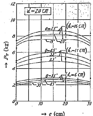
第 29 圖 同上 d = 20 cm
