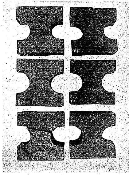
第 18 圖 引張試験片切断状況 ターペンタイン村(氣乾)
