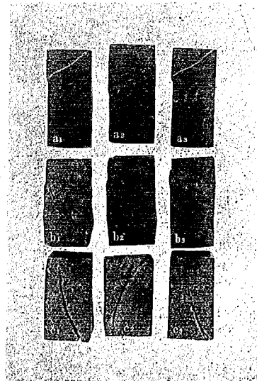
第 11 圖 壓縮試験片(乙) 破壊状況—カボール材(氣乾)
