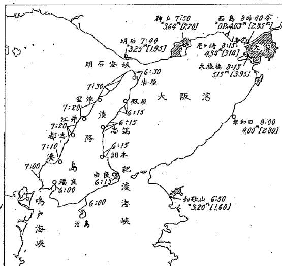
第 9 圖 大阪湾附近各地に於て最高水位に達した時刻及潮位上昇
