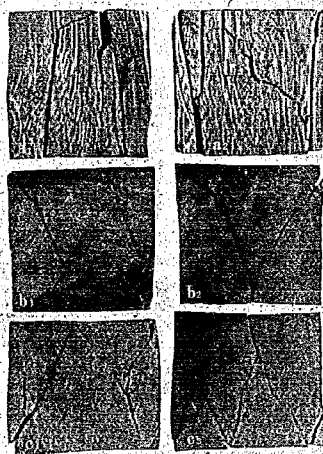
第 7 圖 壓縮試験片(甲)破壊状況—カボール材 (絶對乾燥)
