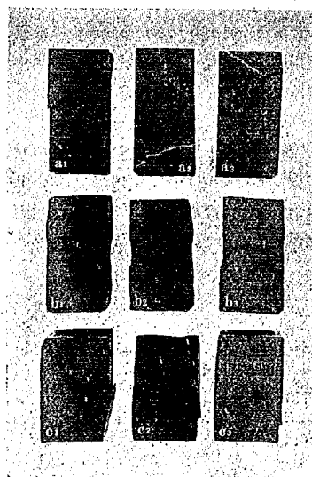
第 12 圖 壓縮試験片(乙) 破壊状況—ターペンタイン材(氣乾)
