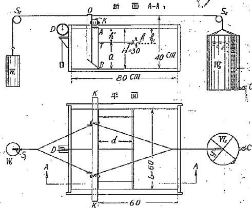
第 8 圖 試験装置
