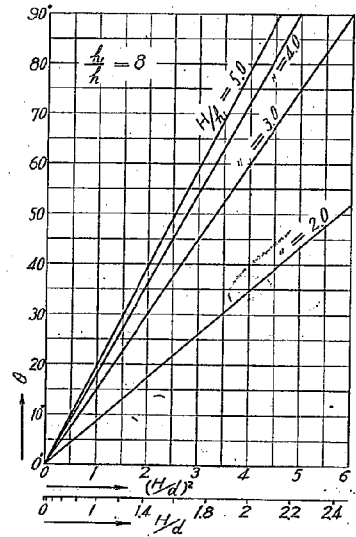
第37圖 同上 h_1/h=8 の場合。
