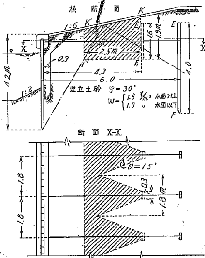
第 38 圖 實際の矢板物揚場に新計算法を適用して版控の位置及寸法を決定した一例。EF は實際に施工されたもの、新計算法に依れば E_1F_1 で十分である。
