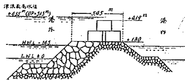
第 13 圖 内港防波堤断面
