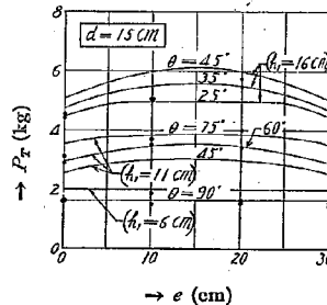
第 28 圖 連続版でない控版が深い位置にある場合の版の間隔 e の影響試験の結果、記入の曲線は第 32 圖に於て斜線を施した部分の砂が控版の支持力に影響するとして算式 (4) により \theta の種々の値に對する P_T を示す。 h = 2 cm, d = 15 cm の場合
