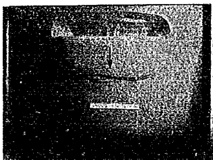
第 41 図 試験後の砂の表面、版が壁より十分遠方にある場合 h=h_1=6\text{ cm} , e=0
