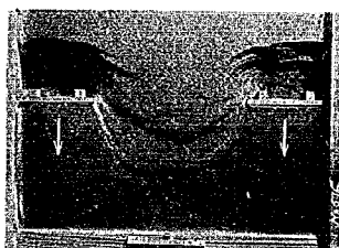
第 26 圖 同上 e=30 cm
