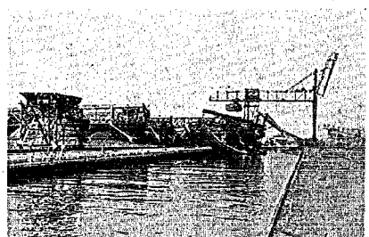
第 23 圖 大阪港梅町棧橋附近のトランスポータークレーンの崩壊(9 月 27 日撮)。漂流船による被害と推定される
