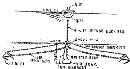
第20図 大阪港内繫船浮標の構造
