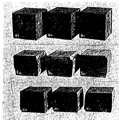
第 10 圖 壓縮試験片(甲)破壊狀況ターペンタイン材(氣乾)
