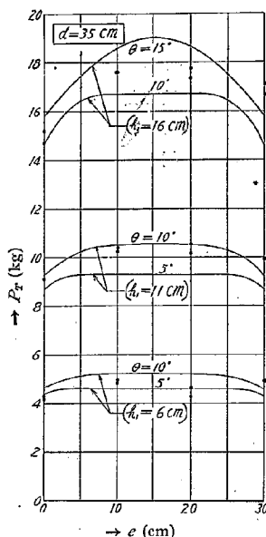
第 31 図 同上 d=35 cm
