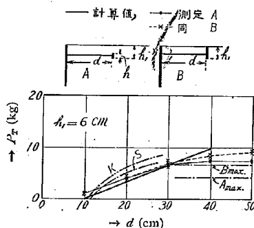
第 12 圖 壁に近い位置にある控版の支持力 試験結果 h_1 = 6 cm
