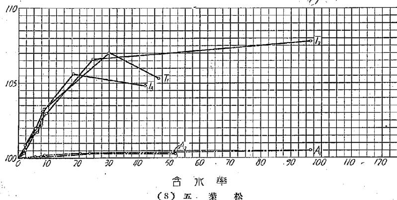
第2表 飽水状態より絶対乾燥に至るまでの収縮率
