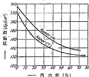
第 23 圖 カボル剪断強と含水率との關係
