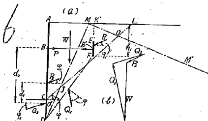
第3圖 控版が壁に最も接近して置かれてある場合の力の平衡状態
