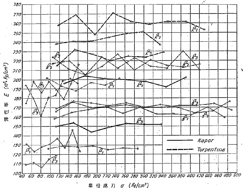
第 30 圖 應力強度の増減に伴ふ引張彈性率の變化
