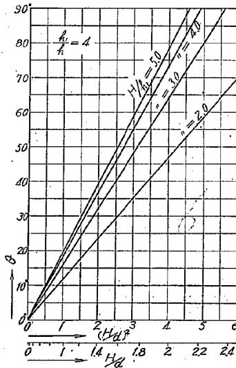
第36圖 同上 h_1/h=4 の場合。
