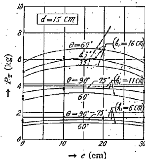
第 20 圖 控版の間隔 e の影響試験の結果、記入の曲線は第 6 圖に於て斜線を施した部分の砂が控版の支持力に影響するとして算式 (4) により \theta の種々の値に對する P_T を示す。 d=15 cm. の場合
