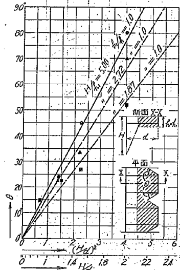
第 27 圖 控版が壁に接近して置かれてある場合二枚の控版の間隔 e の影響を試験した結果、太い直線は \theta = k(H/d)^2 と假定し試験した結果の各の平均値を表はす。
