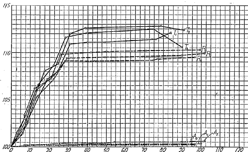
第 5 圖 含水率と收縮率との關係
