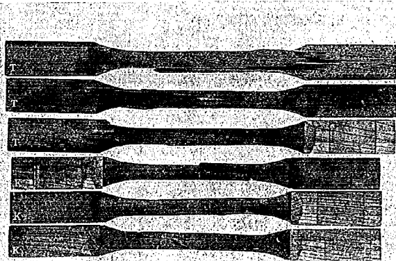
第15圖 氣乾狀態引張試片の切斷狀況 (K-カボール材)(T-ターペンタイン材)
