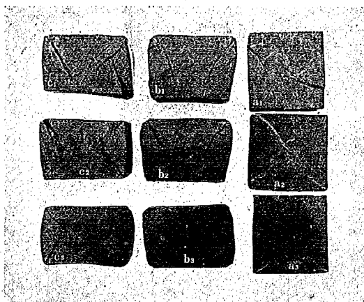
第 9 圖 壓縮試験片(甲)破壊狀況カボール材(氣乾)
