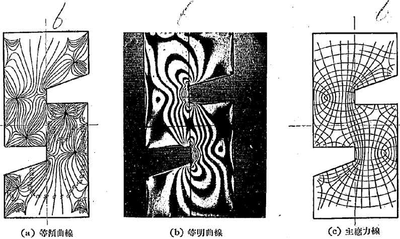
第 21 圖 木村剪断試験片應力分布圖
