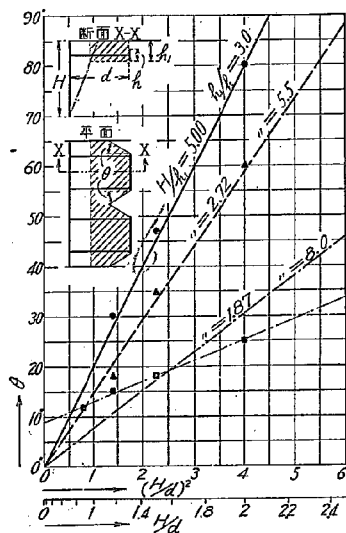
第 33 図 第 32 図の場合に間隔 c の影響を試験した結果。 \theta = k(H/d)^2 と假定し k に適當の値を與へて試験した結果の各の平均値を圖の太い直線に表はす。
