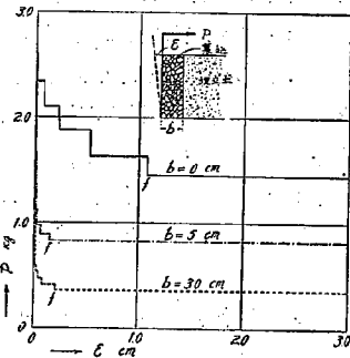
第5圖 壁の動き( e )と力( P )との關係
