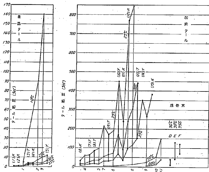
第2図 各温度に於けるターール粘度
