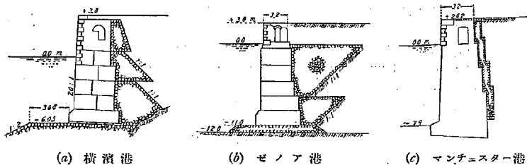
第 1 圖 岸壁及裏込断面
