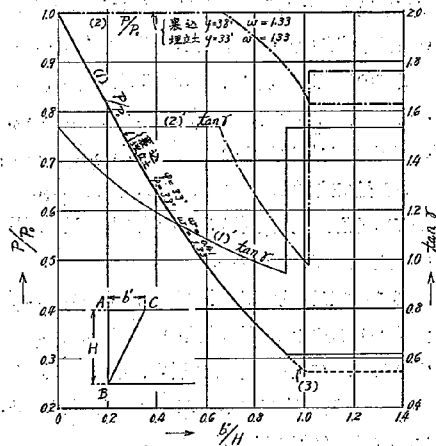
第 14 圖 裏込と埋立土の w 或は \varphi 何れかの一のみが異つた場合に對する計算値。但し裏込の斷面は ABC なる直角三角形の場合
