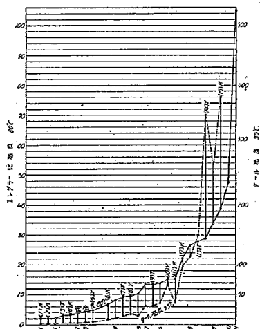
第4図 比粘度 80°C 及ターール 粘度 35°C の比較
