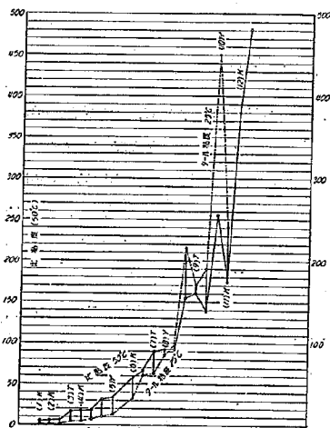
第3図 比粘度 50°C 及ターール 粘度 25°C の比較
