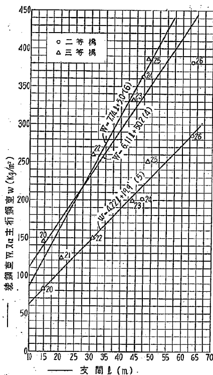
第 2 圖 上路直弦鋼構橋の鋼重
