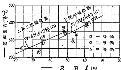
第7圖 上路二鈹鋼筋拱橋及び上路腔槽拱橋の鋼重
