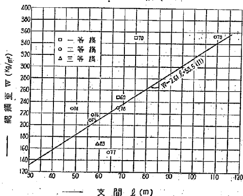
第5圖 3 徑間ゲルバー型上路級桁橋の鋼重
