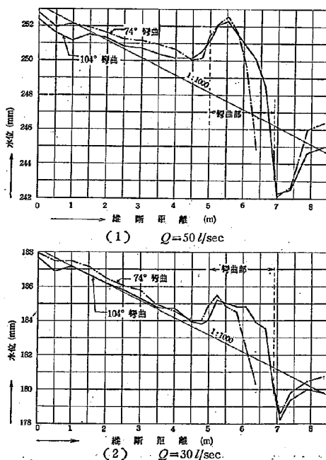
第17圖 水面の縦断形 (梯形水路)
