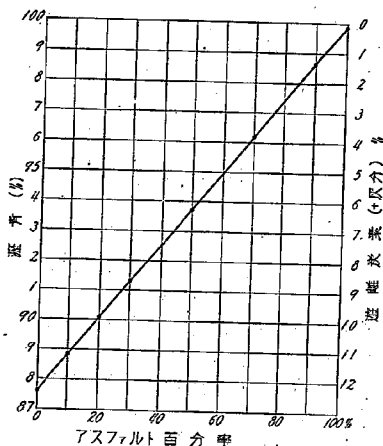
第 13 図 タール・アスファルト混合物の凝固點及遊離炭素量
