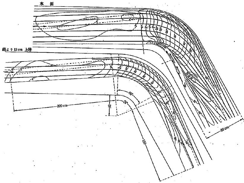
第 16 圖 彎曲部附近の流向 梯形断面 74° 彎曲 Q=50 \text{ l/sec}
