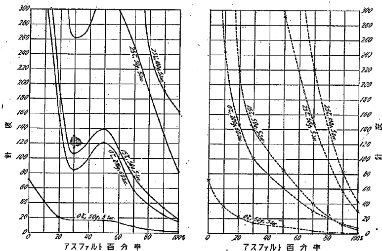
第 11 圖 タール・アスファルト混合物
