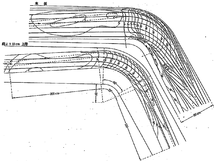
第 16 圖 彎曲部附近の流向 梯形断面 74°彎曲 Q=50 l/sec
