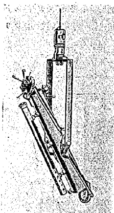
第2図 エクマン 可逆採水器
