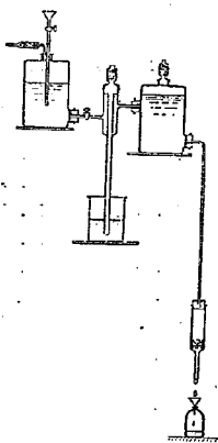
第 4 圖 透水實驗裝置
