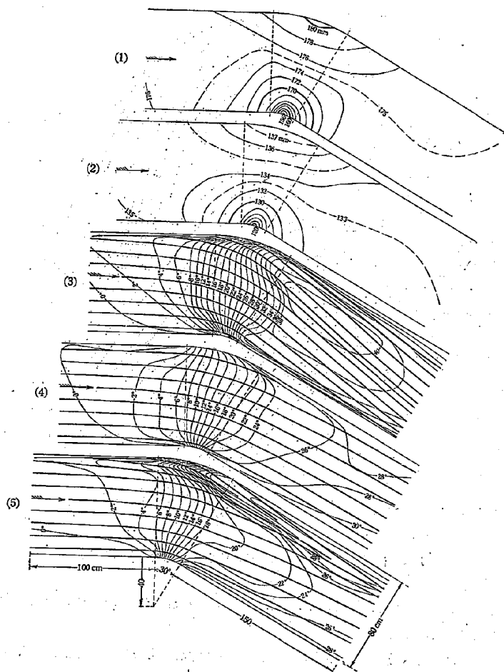
第 11 圖 彎曲部附近の流向及び水面形，矩形断面 30°彎曲
