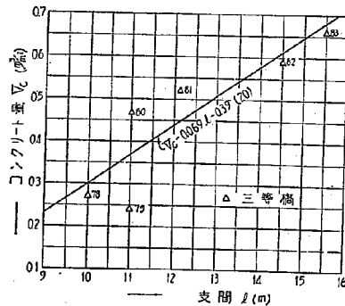
第13圖 2徑間連續鐵筋コンクリート桁橋のコンクリート量
