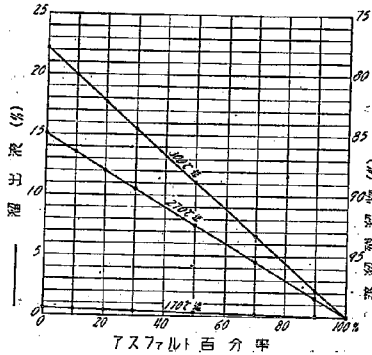
第 14 圖 タール・アスファルト混合物溜出液量及蒸溜残留物量計算値、(但しアスファルト中 300°C 迄は溜出成分なしと假定す)
