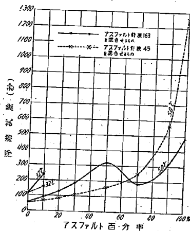
第9圖 タール・アスファルト 混合物浮游試験
