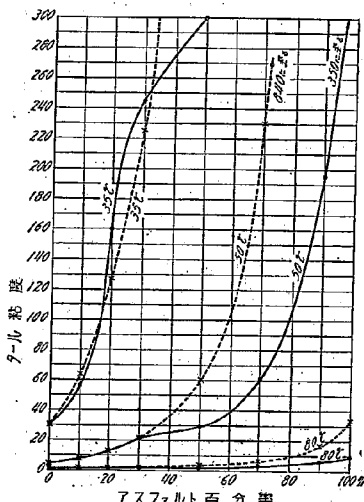
第 8 図 タール・アスファルト 混合物タール粘度
