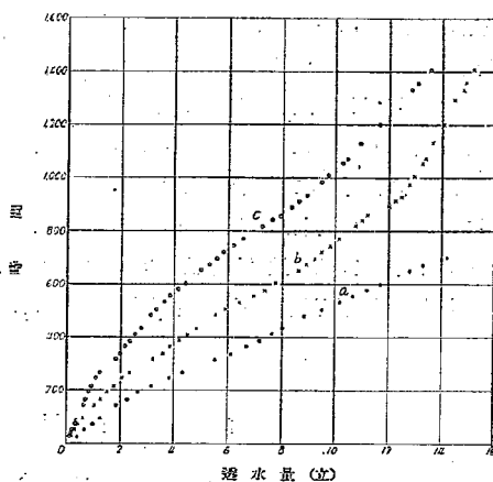
第 5 圖 透水速度
