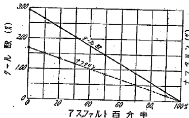
第 12 図 タール・アスファルト混合物中タール酸及ナフタリンの量
