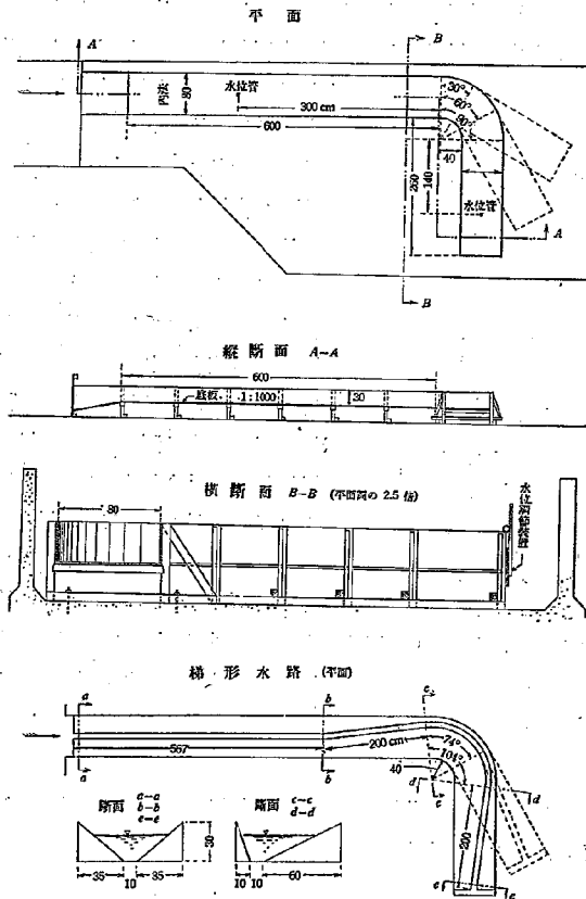
第2圖 彎曲水路實驗設備
