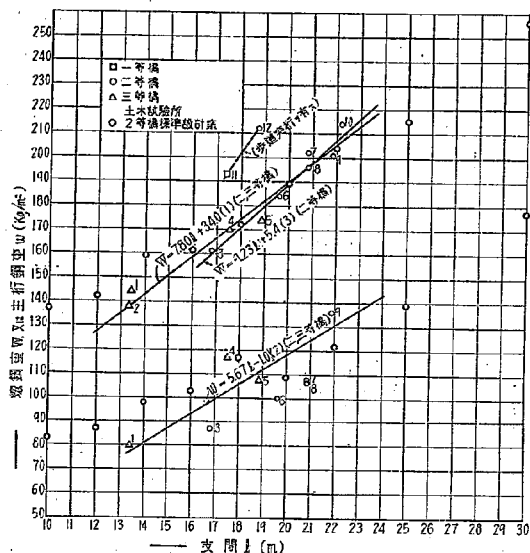
第 1 圖 上路鋼桁橋の鋼重
