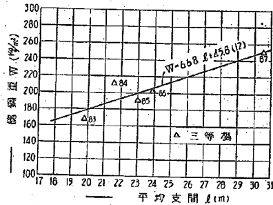
第6圖 三等橋ゲルバー型鉸拱橋の鋼重
