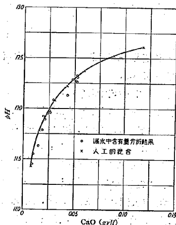
第 6 圖 漏水の石灰含有量と pH
