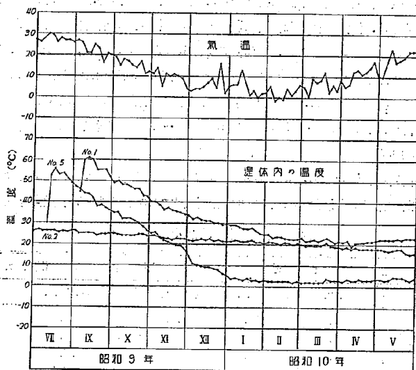
第 4 圖 堤體内部の温度
