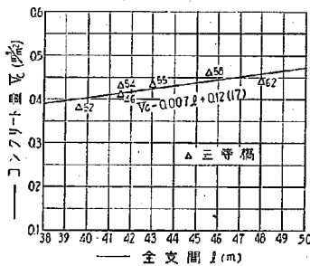
第 10 圖 3 標間ゲルバー型鉄筋コンクリート桁橋のコンクリート量
