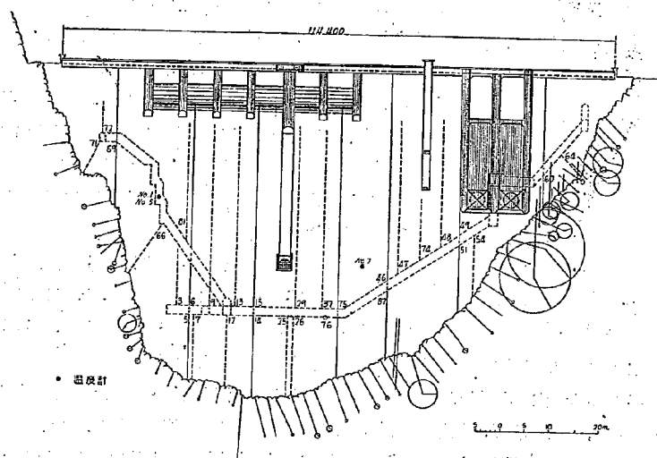
第1図 王泊堰堤上流面図
