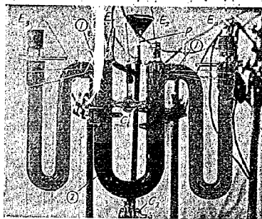
写真第 8 タール乳剤電気泳動實驗用管
