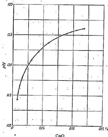
第 1 圖 石灰溶液の pH
