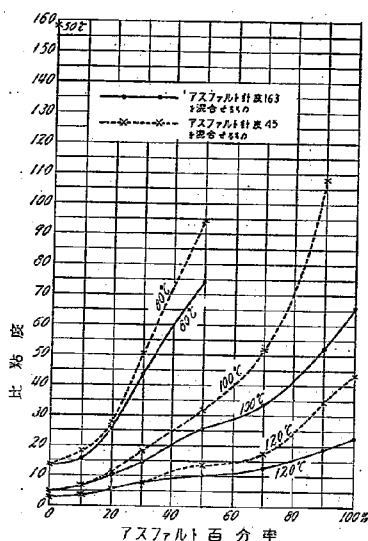
第 7 圖 アスファルト混合物比粘度
