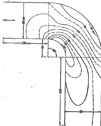
第8圖 彎曲部附近の水面形矩形断面 90°彎曲 Q=32 l/sec 金網張り
