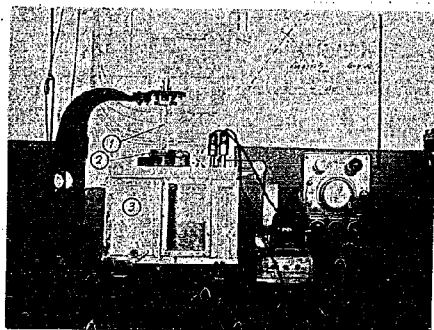
写真第 7 回轉圓筒粘性係數實驗裝置
