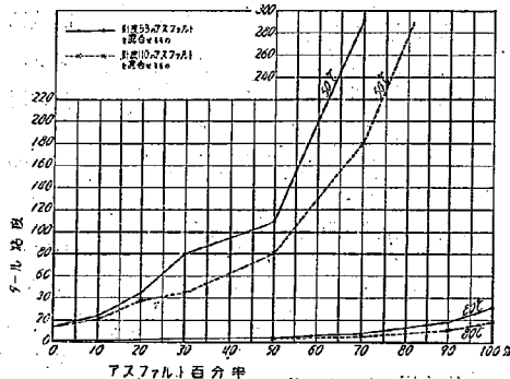
第2圖 アスファルトの混合量とタール粘度
