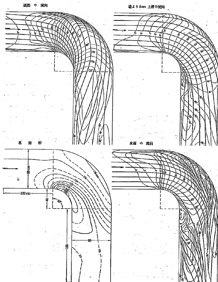
第7圖 彎曲部附近の流向及び水面形, 矩形 90°彎曲 Q=47 l/sec 金網張り
