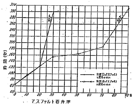
第3図 アスファルト混合量と浮游試験 (50°C)
