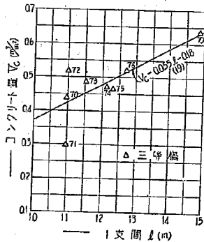
第12圖 3徑間連續鐵筋コンクリート桁橋のコンクリート量
