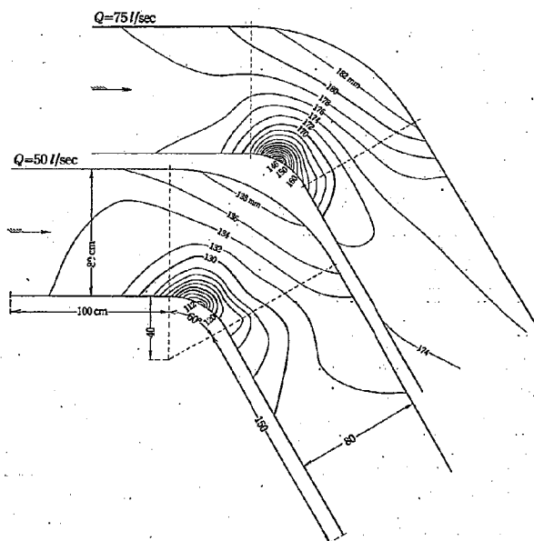
第 9 圖 彎曲部附近の水面形、矩形断面 60°彎曲
