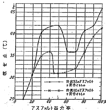
第4図 タール及アスファルト混合物 軟化点 (タール No. 1991)
