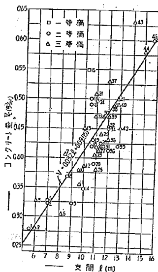
第8圖 丁型鉄筋コンクリート単桁橋のコンクリート量
