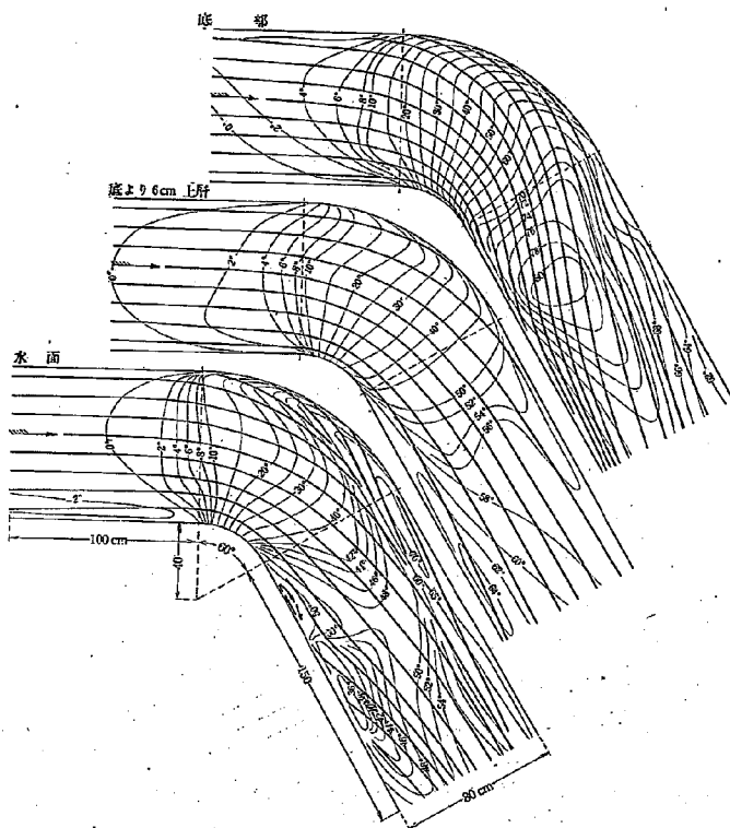
第 10 圖 彎曲部附近の流向，矩形断面 60^\circ 彎曲 Q=50 \text{ l/sec}
