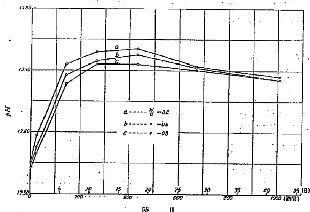
第3圖 硬化セメントの溶液に於ける pH の時間的變化
