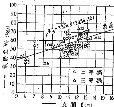
第9圖 丁型鉄筋コンクリート単桁橋の鉄筋量
