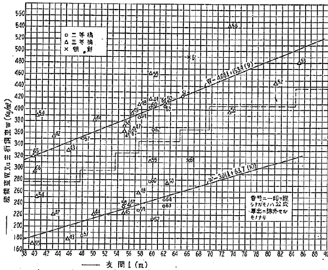
第4圖 下路曲弦鋼構橋の鋼重
