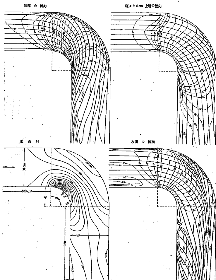
第 5 図 彎曲部附近の流向及び水面形，矩形断面， 90^\circ 彎曲， Q=75 \text{ l/sec}
