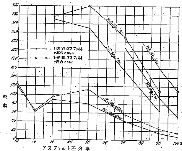
第 5 圖 アスファルト混合量と針度
