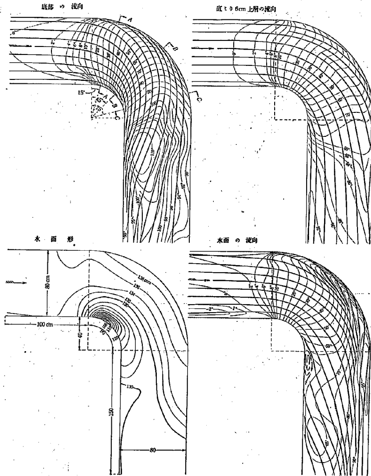
第4圖 彎曲部附近の流向及び水面形, 矩形断面 90°彎曲 Q=50 //sec
