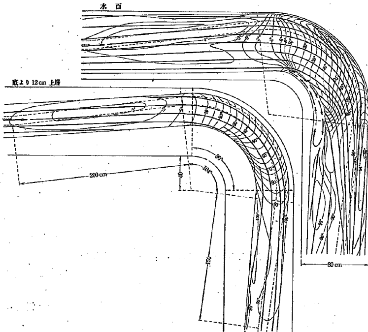
第 14 圖 彎曲部附近の流向 梯形断面 104°彎曲 Q=50 l/sec
