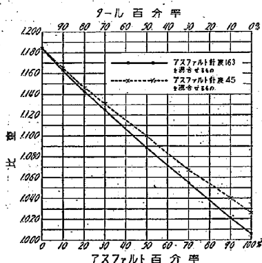
第 6 圖 タール・アスファルト混合物比重計算値(但し混合の際容積の變化なきものと假定す)
