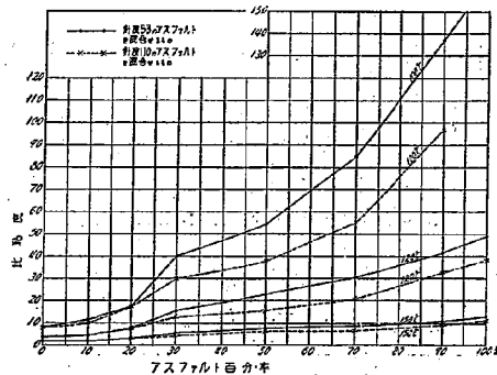
第1圖 アスファルトの混合量と比粘度
