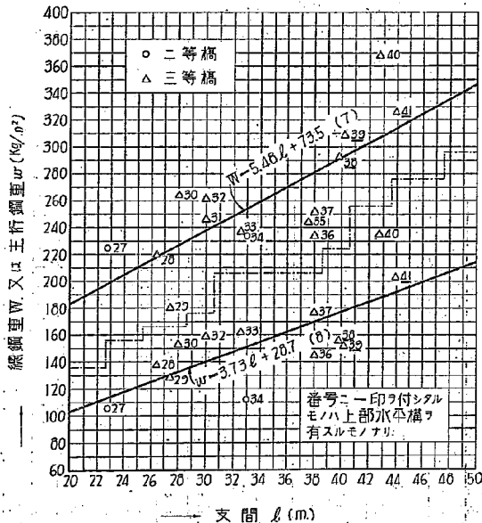
第3圖 下路直弦鋼構橋の鋼重
