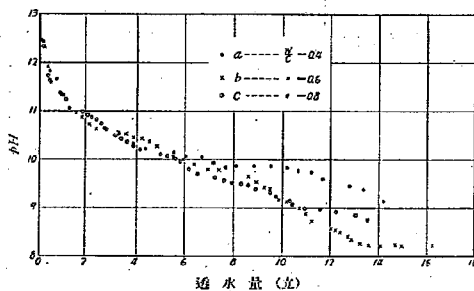
第 6 圖 硬化セメントに於ける透水量と其の pH との関係
