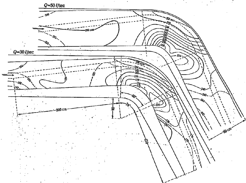
第 15 圖 彎曲部附近の水面形，梯形断面 74^\circ 彎曲
