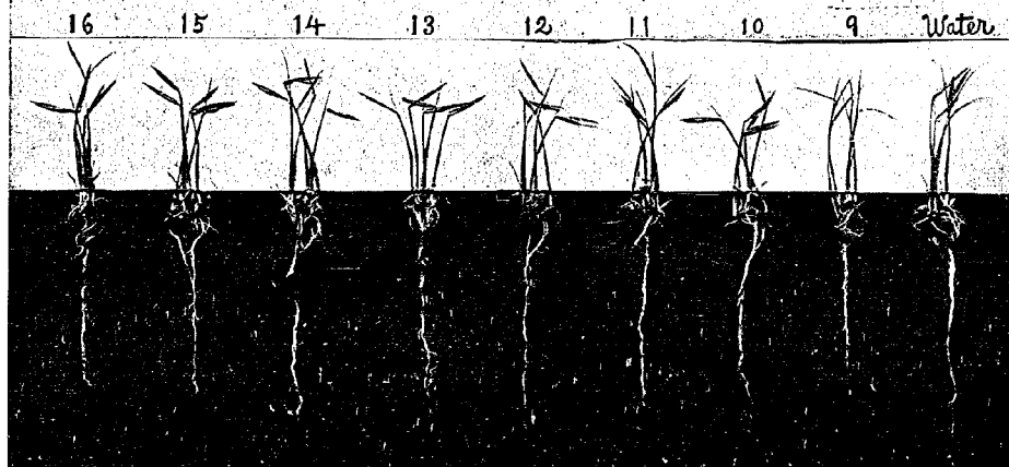
寫眞〔XV〕 タール酸含有量 0.88% 及 0.41% のタールを用ゐたるタール舗装上を流るゝ水の影響(土耕)
