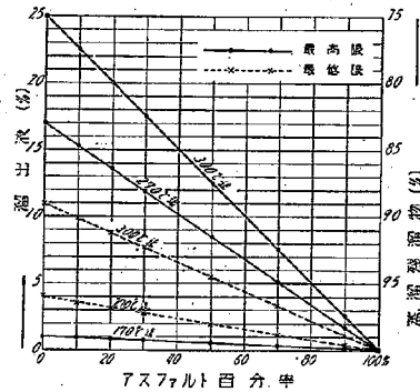
第 15 圖 規格案 E タールにアスファルトを混合せるものゝ溜出液量計算値
