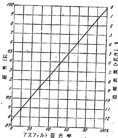
第 13 図 タール・アスファルト混合物の凝固點及凝固炭素量
