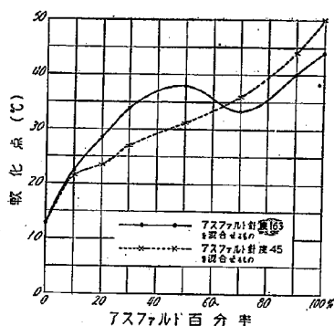
第 10 圖 タール・アスファルト混合物軟化點 (R&B).....°C
