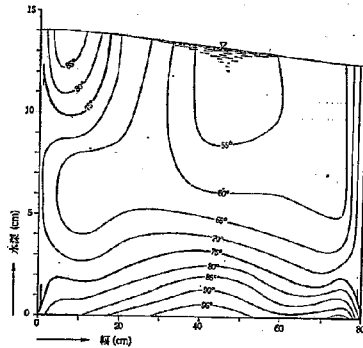
(c) 斷面 C-C
