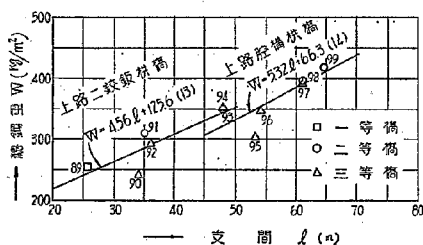
第7圖 上路二鈹拱橋及び上路腔槽拱橋の鋼重
