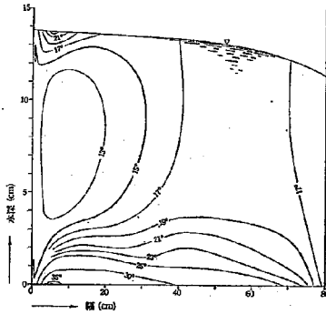
(a) 斷面 A-A
