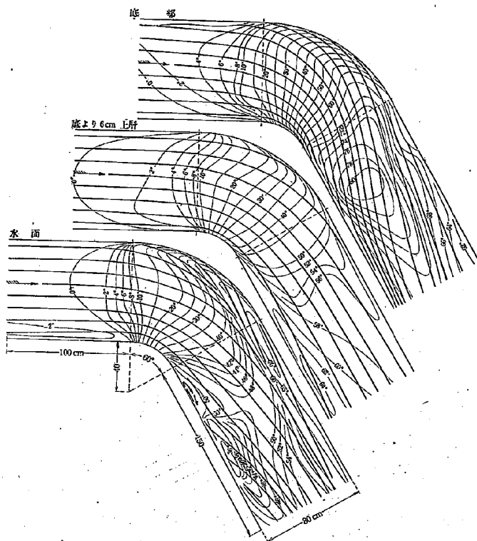
第 10 圖 彎曲部附近の流向，矩形断面 60^\circ 彎曲 Q=50 \text{ l/sec}
