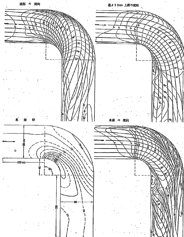
第7圖 彎曲部附近の流向及び水面形, 矩形 90°彎曲 Q=47 l/sec 金網製リ
