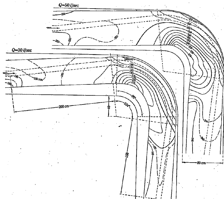
第13圖 彎曲部附近の水面形、梯形斷面 104^\circ 彎曲
