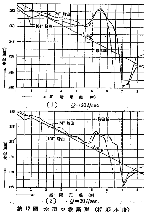
第17圖 水面の縦断面形 (梯形水路)
