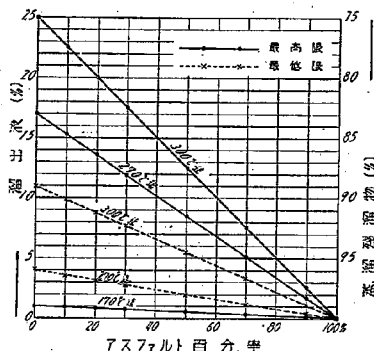
第 15 圖 規格案 15 タールにアスファルトを混合せるものゝ溜出液量計算値
