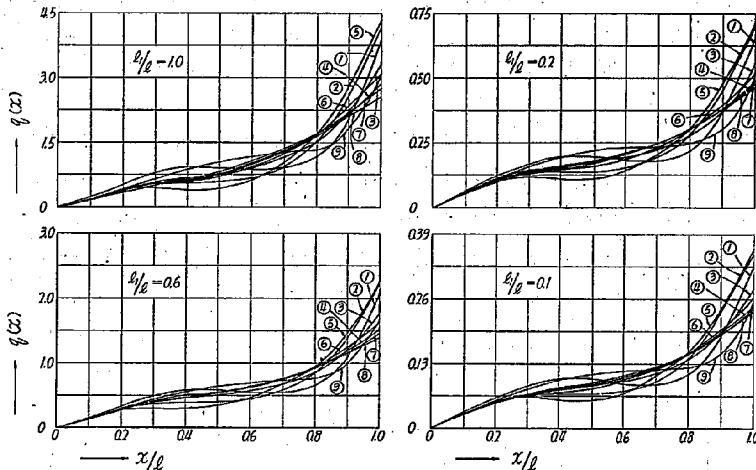
第 3 圖 (a) 地盤反力の値 (但し圖中の値は q_0 の係數を示す)
