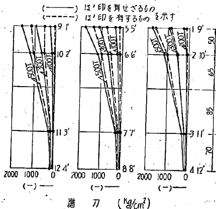
第 31 圖 主肋鋸縁應力の變化
