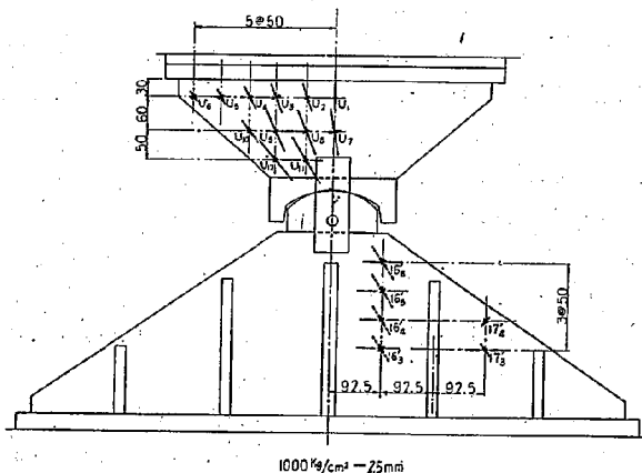
第17圖 主肋板に於ける主應力
