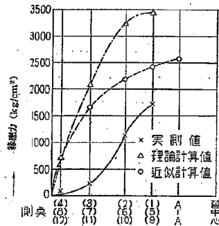
第33圖 主肋鉄線應力の分布
