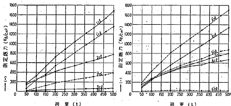
第9圖 主肋鈹縁應力
