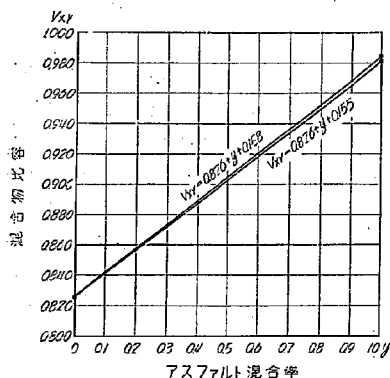
第 1 圖 アスファルト混合タールの比重
