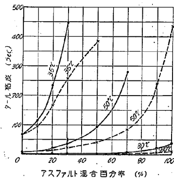
第 3 圖 タール・アスファルト 混合物タール粘度 (備考は第 2 圖と同じ)
