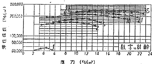
第 17 圖 上層コンクリートの引張に對する弾性係數
