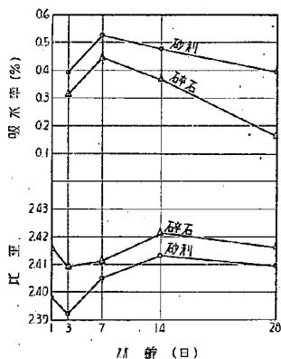
第 22 圖 砂利及砕石コンクリートの比重及吸水率
