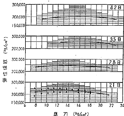
第 16 圖 上層コンクリートの引張に對する弾性係數
