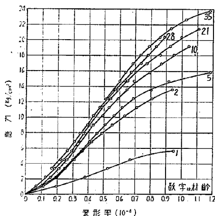
第 15 圖 上層コンクリートの引張に對する變形率
