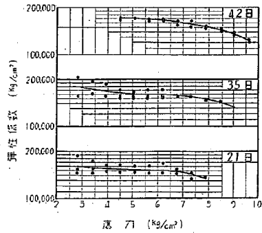
第8図 基層コンクリートの引 張に対する弾性係数
