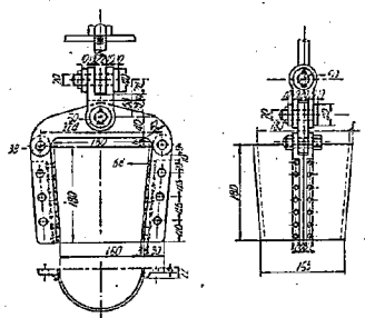
第 2 圖 引張試験個金物
