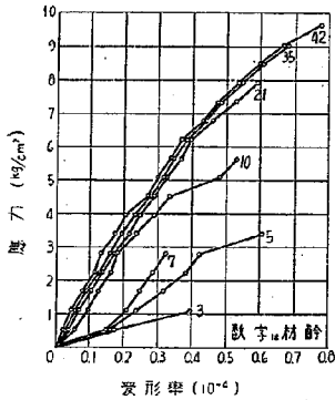
第7図 基層コンクリートの 引張に対する変形率
