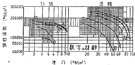
第10図 基層コンクリートの引張及 壓縮に対する弾性係數
