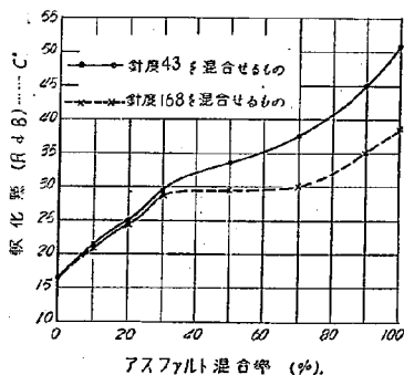
第 5 圖 軟化點
