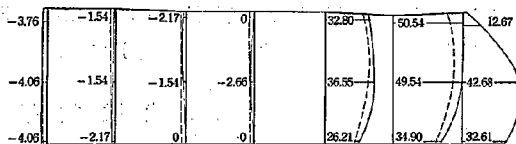
第 7 圖 断面 2
