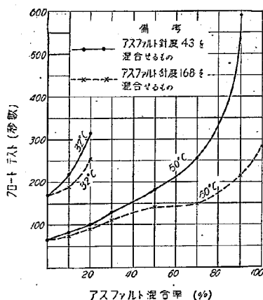
第 4 圖 浮游試験
