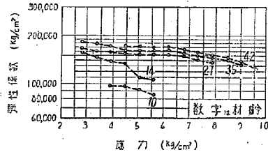
第9図 基層コンクリートの引 張に対する弾性係數
