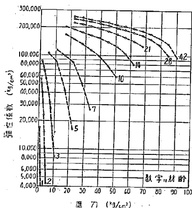
第6図 基層コンクリートの壓縮に に対する弾性係数
