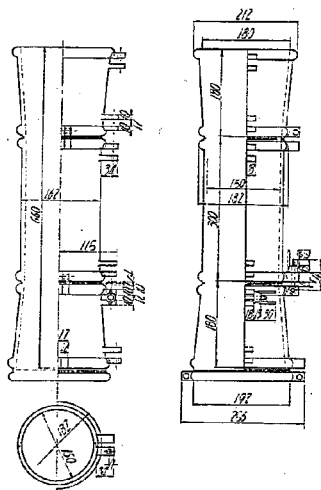
第 1 圖 引張試験體型
