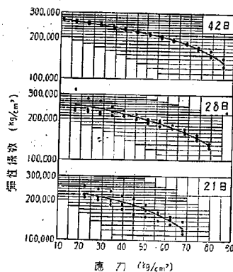
第5図 基層コンクリートの壓縮 に対する弾性係数
