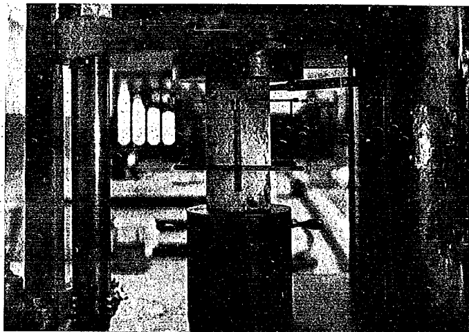
第 23 圖 コンクリートの圧縮試験装置
