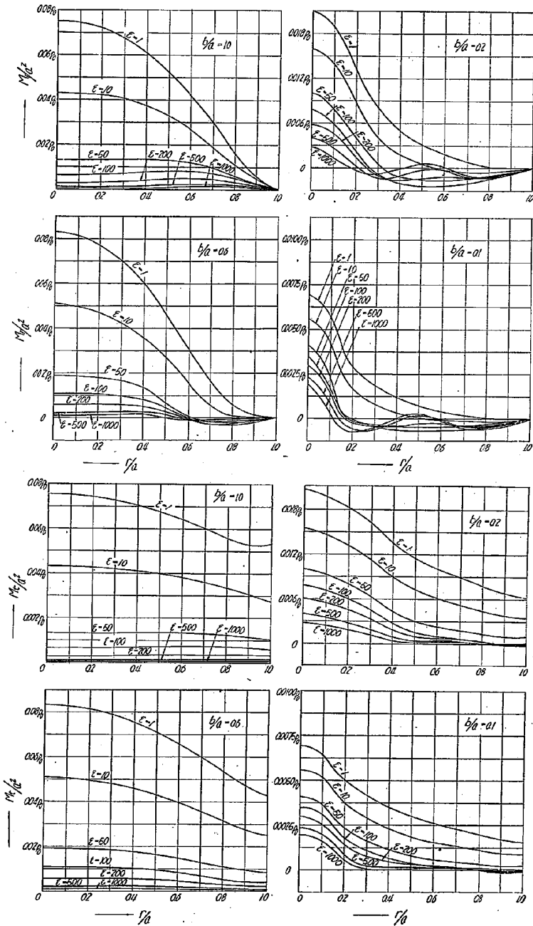
第5圖(2), \epsilon の変化による影響 ( \epsilon=0\sim1000 )
