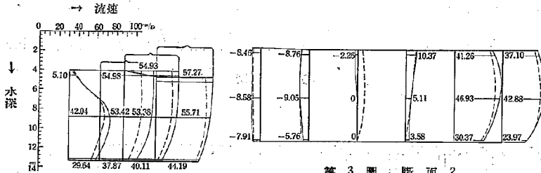
第 3 圖 断面 2
