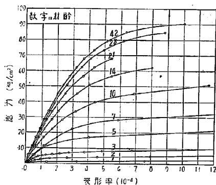
第4図 基層コンクリートの壓縮 に対する變形率
