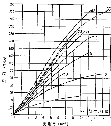
第 12 圖 上層コンクリートの壓縮に對する變形率 ( 9 )
