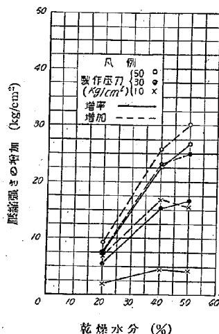
第 6 圖 壓縮強さの増加と乾燥水量
