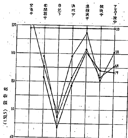
第 8 圖 ストレート・アスファルト (40~50) 25°C 稠度変化 但し、(1mm, 50g, 5sec) の微針度
