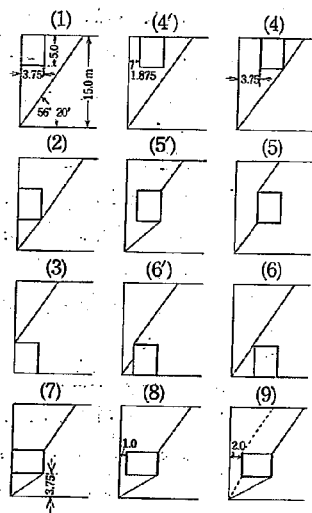
第 6 圖 清水港の場合に就て方塊の種々の位置が崩壊面に及ぼす影響を算定する。細い斜線は崩壊面を示す
