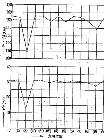
第 7 圖 第 6 圖の崩壊面による岸壁への壓力及その岸壁前趾の周りの力率
