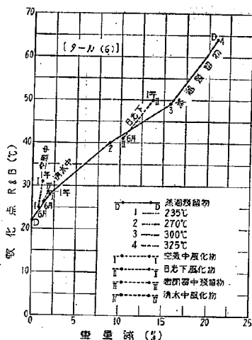
第 37 圖 タール (6) 蒸溜殘留物及風化殘留物の軟化點と重量變化との比較
