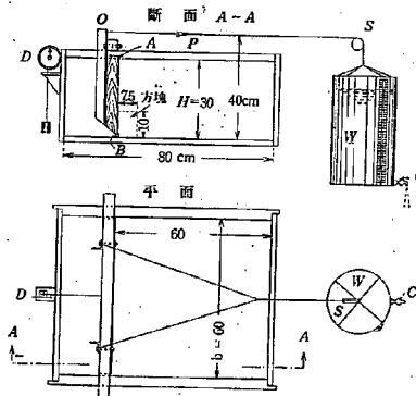
第 2 圖 試験装置
