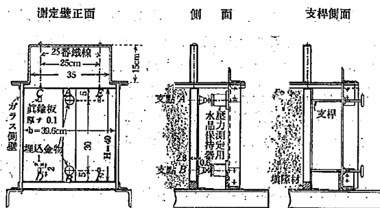
第 9 圖 振動試験の壓力測定裝置
