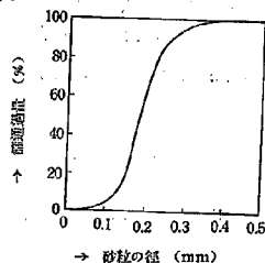
第4圖 試験砂篩分
