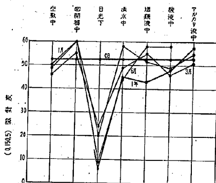
第 15 図 ブローン・アスファルト (10~20)
