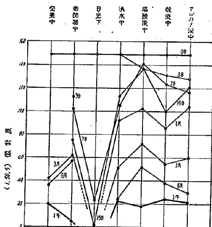
第23圖 加熱混合マカダム用タール(6)
