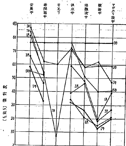
第 10 図 ストレート・アスファルト (150~200) 25°C 稠度変化 但し, (5mm, 50g, 5sec) の微針度
