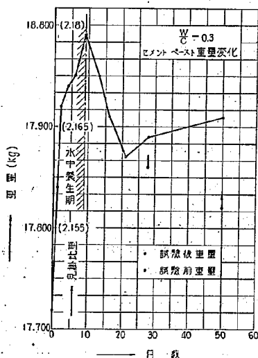
第19圖 w/c=0.3 セメントペースト 實驗中の重量變化
