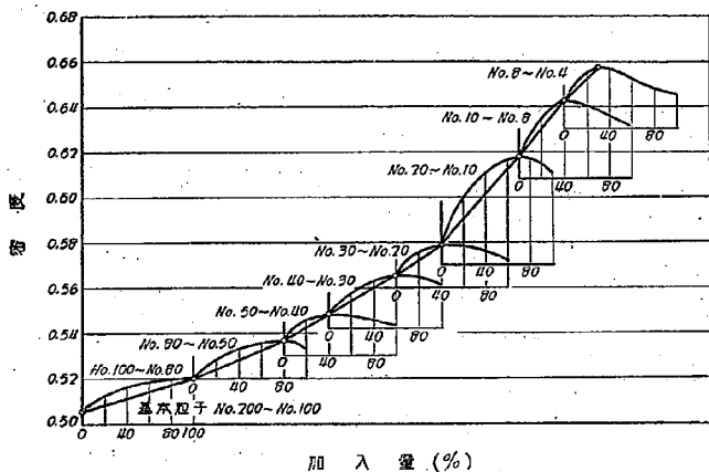
第 2 図 砂の最大密度曲線(フローテール30回)
