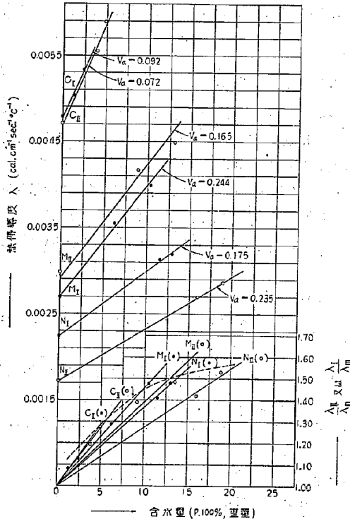
第 26 図 コンクリート、モルタル、セメントペースト熱伝導度と含水量の関係を示す
