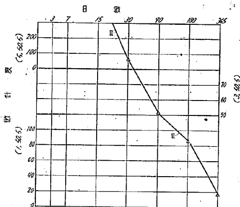
第 19 圖 加熱路面處理用タール (5) 25°C 微針度 (日光下試料)
