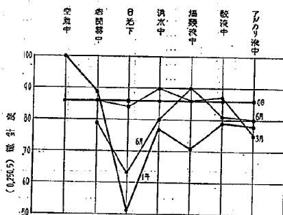
第 13 図 ストレート・アスファルト (150~200) 1.0°C 稠度変化 但し, (0mm, 250g, 5sec) の微針度
