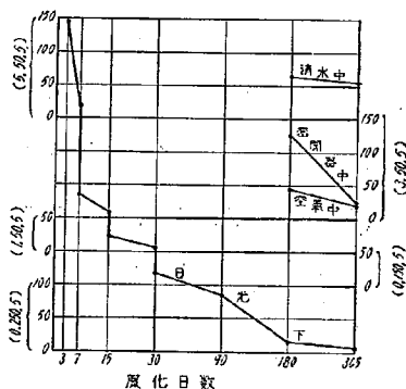
第 21 圖 加熱路面處理用タール (5) 1.0°C 稠度變化
