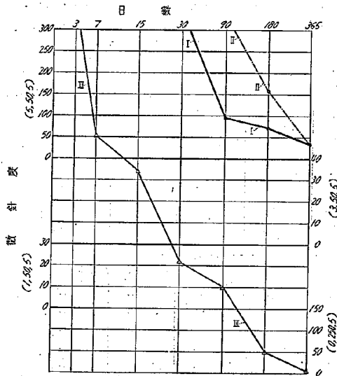
第 18 圖 常溫用タール(4) 1.0°C 微針度
