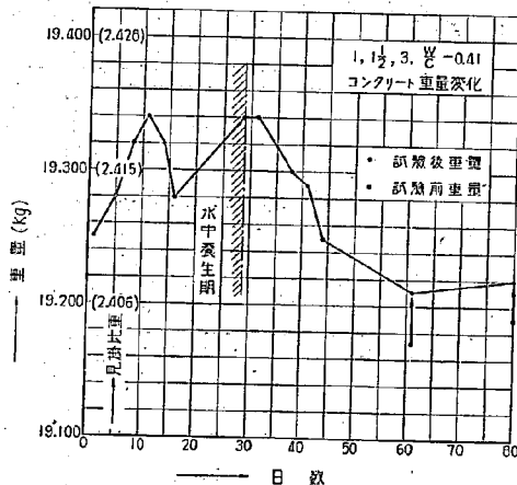
第15図 実験中に於ける供試體重量変化
