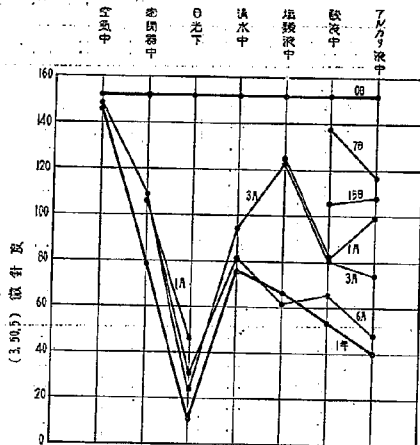
第 11 図 ストレート・アスファルト (150~200) 25°C 稠度変化 但し, (3mm, 50g, 5sec) の微針度
