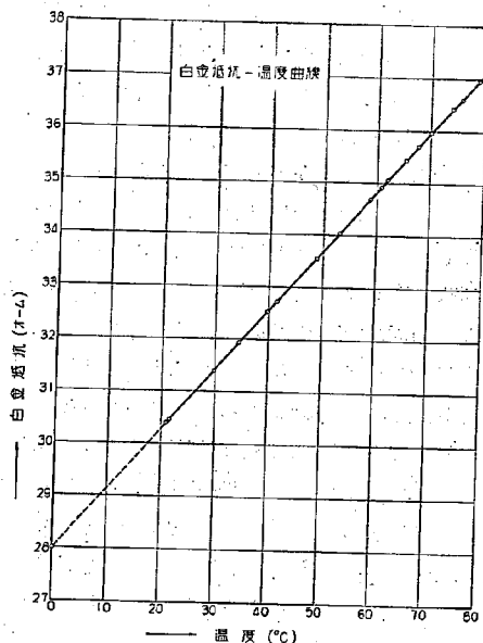
使用白金抵抗温度計の電気抵抗と温度との関係 第 3 圖
