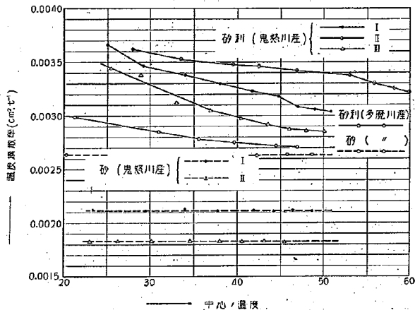
第23圖 鬼怒川産及び多摩川産砂利、砂の温度擴散率—中心温度との關係
