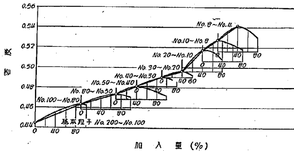
第 5 圖 (碎石屑フローテブル30回)
