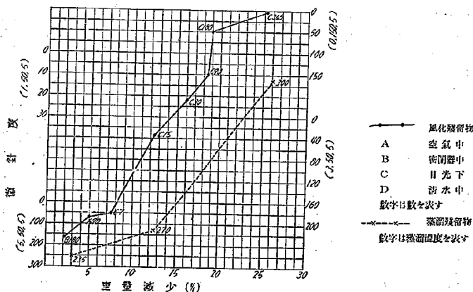
第 39 圖 タール(4) 蒸溜残留物、風化残留物 1.0°C 微針度と重量變化
