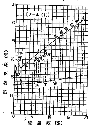
第34圖 タール(7)の蒸溜残留物及炭化 残留物中遊離炭素量と重量変化との比較
