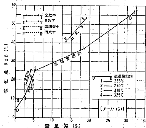
第 36 圖 タール (5) 蒸溜残留物及風化残留物の軟化点と重量變化との比較
