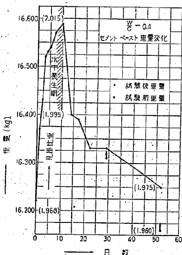
第20圖 w/c=0.4 セメントペースト 實驗中の重量變化
