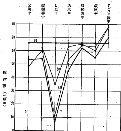
第 14 図 ブローン・アスファルト (10~20)
