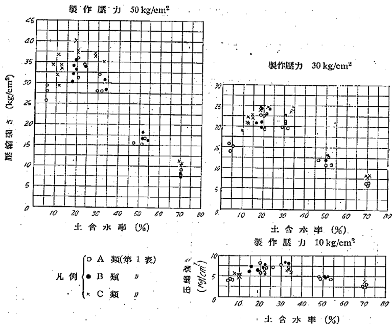
第 1 圖 土の乾燥に伴ふ壓縮強さの變化
