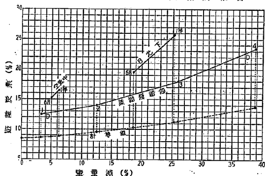
第31圖 タール(4)の蒸溜残留物及炭化残留物 中遊離炭素量と重量変化との比較
