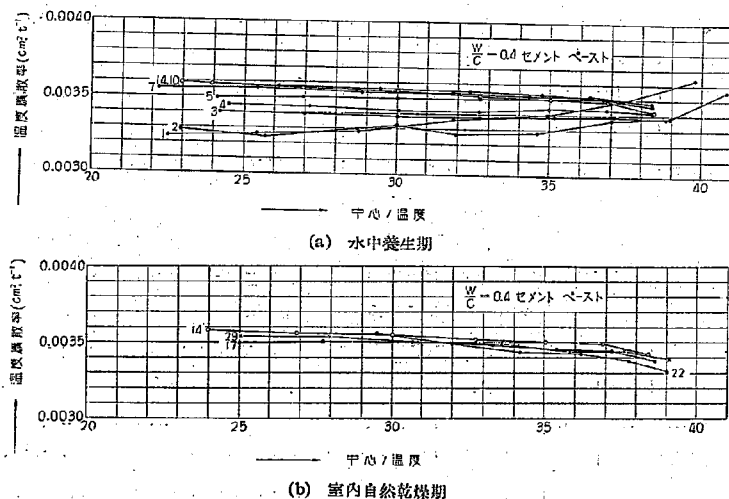
第 22 圖 w/c=0.4 セメントペースト温度擴散率と中心温度關係 (高温恒温槽約 40^{\circ}\text{C} )
