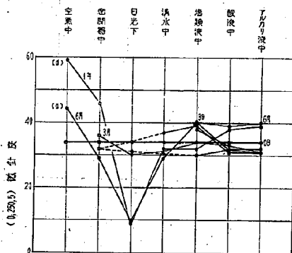
第 9 圖 ストレート・アスファルト (40~50) 1.0°C 稠度変化 但し、(0mm, 250g, 5sec) の微針度
