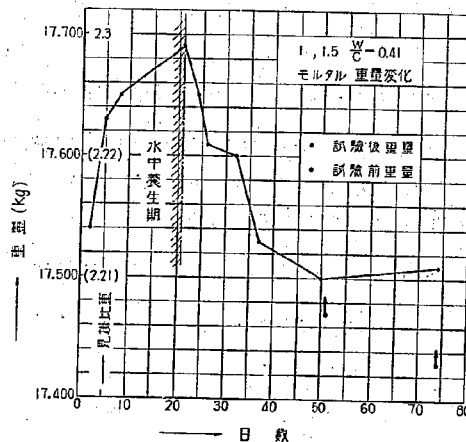
第 17 圖 實驗中に於ける供試體重量變化
