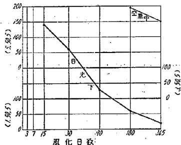
第 22 図 加熱混合マカダム用タール(6) 25°C 微針度、日光下及空空中試料
