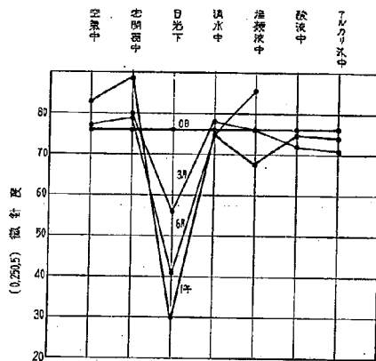
第 16 圖 ブrown・アスファルト (10-20) 1.0°C 稠度變化 但し、(0mm, 250g, 5sec) の微針度
