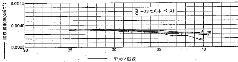
(b) 室内自然乾燥期 (高温恒温槽約 45^{\circ}\text{C} )
