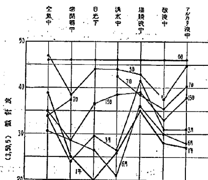
第 7 圖 ストレート・アスファルト (40~50)
