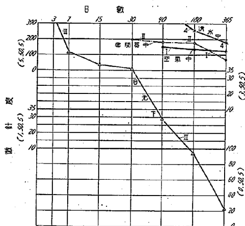
第 25 圖 加熱混合用タール (7) 25°C 微針度
