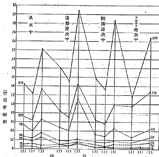
第3圖 アスファルト薄層重量變化 清水中、鹽液中、酸液中、アルカリ液中 試料は第1圖と同じ
