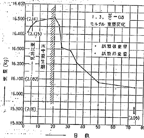
第 13 圖 實驗中に於ける供試體重量變化
