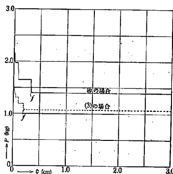
第 3 圖 P と壁の移動量 \varepsilon との関係
