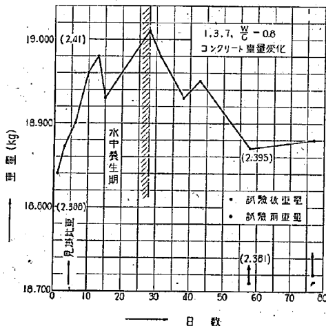
第 11 圖 實驗中に於ける供試體重量變化
