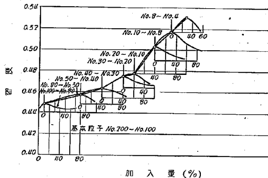
第 4 圖 碎石屑(フローテブル20回)
