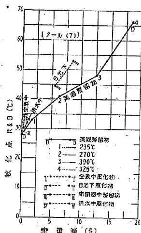
第 38 圖 タール (7) 蒸溜殘留物及風化殘留物の軟化點と重量變化との比較
