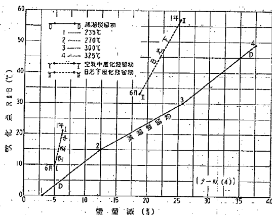
第 35 圖 タール (4) 蒸溜残留物及風化残留物軟化点と重量變化との比較
