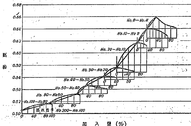
第 1 圖 砂の最大密度曲線(フローテーブル20回)
