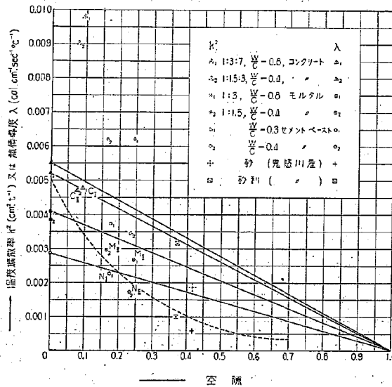
第 24 圖 鋪装コンクリート、モルタル等の温度擴散率、熱傳導度と空隙關係
