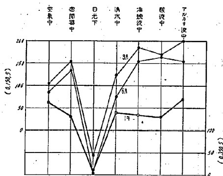
第 27 圖 加熱混合用タール (7) 10°C 稠度變化 但し、(0, 150, 5) 及 (0, 350, 5) 微針度
