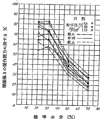
第 4 圖 壓縮強さの製作壓力に対する比率
