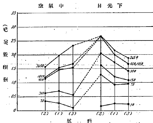
第 1 圖 アスファルト薄層重量變化 但し、實驗室 空氣中、及、日光下
