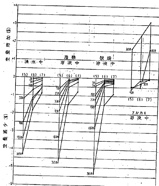
第 6 圖 鉛装用タール重量變化。清水中、鹽液中、酸液中、アルカリ液中
