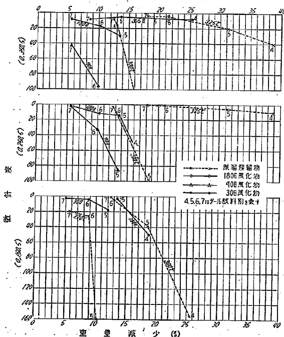
第 43 圖 各種タール蒸溜残留物及日光下風化残留物 1.0°C 微針度比較
