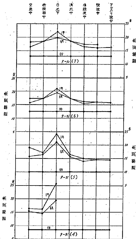
第 28 圖 各種タール風化残留物中の遊離炭素の量
