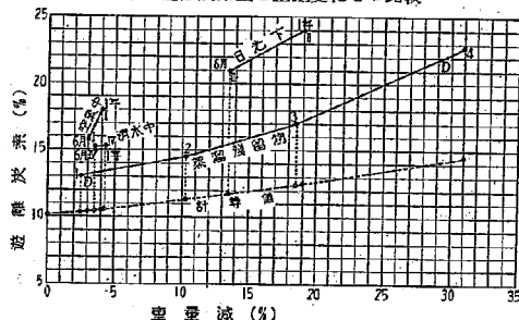
第32圖 タール(5)の蒸溜残留物及炭化残留物 中遊離炭素量と重量変化との比較
