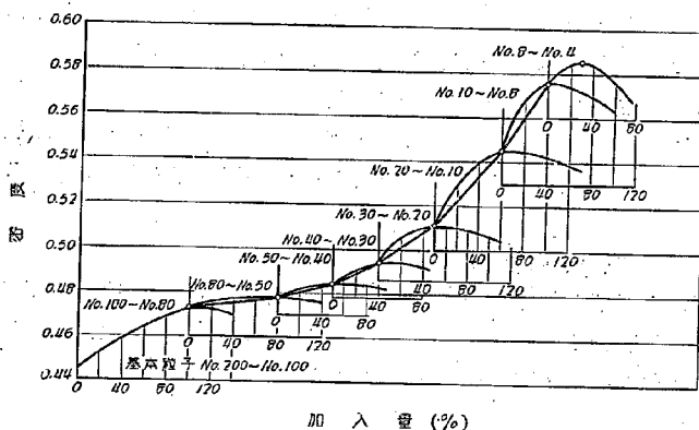
第 6 図 碎石屑(フローテーブル50回)
