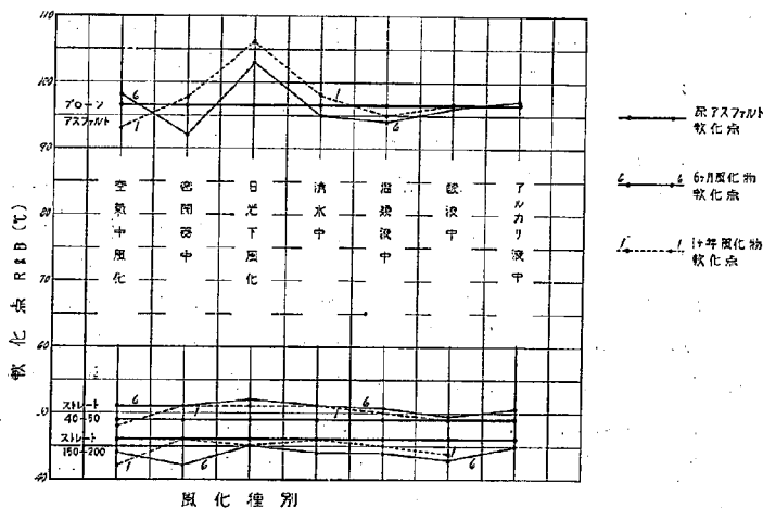
第30圖 各種アスファルト風化殘留物の軟化點變化
