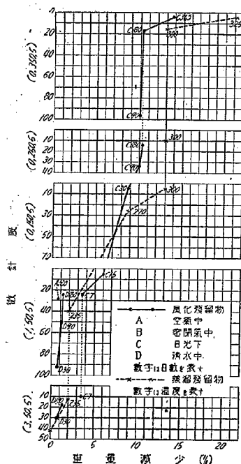
第 41 圖 タール(6)蒸溜残留物及風化残留物 1.0^{\circ}\text{C} 微針度と重量變化
