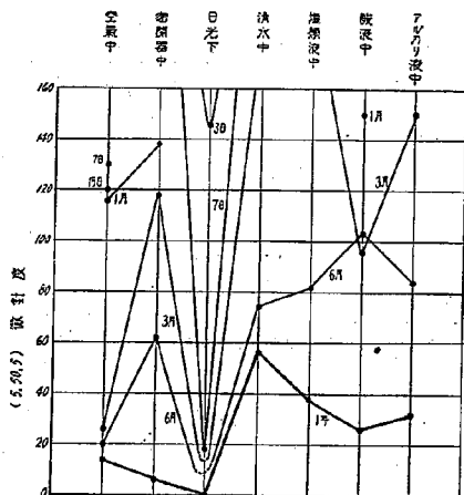
第 20 圖 加熱路面處理用タール (5) 1.0°C 稠度變化 但し、(5mm, 50g, 5sec) 微針度
