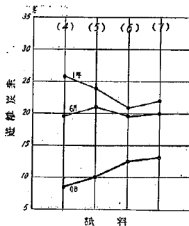
第 29 圖 各種タール日光下風化残留物中の遊離炭素の量
