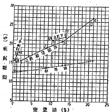
第33圖 タール(6)の蒸溜残留物及炭化残 留物中遊離炭素量と重量変化との比較
