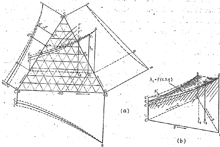
第 25 圖 三角座標にて示せるコンクリート熱傳導度と骨材等の關係
