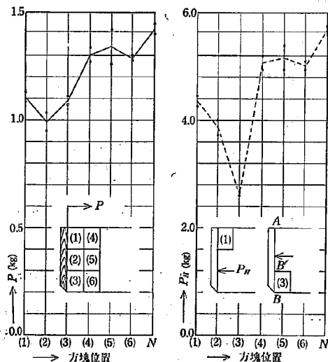
第5圖 方塊の位置による P 及 P_H の變化、方塊位置 (1) (2) 等はカットに示す通りであり、 N は方塊のない状態である
