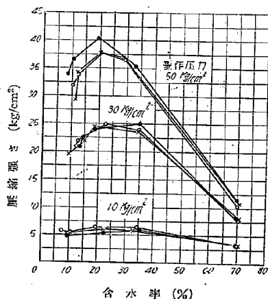
第 2 圖 平均壓縮強さの變化
