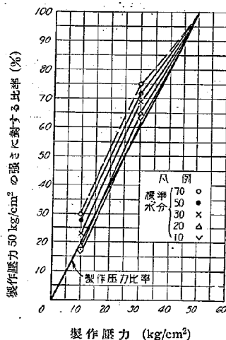
第 5 圖 壓縮強さの製作壓力別比率
