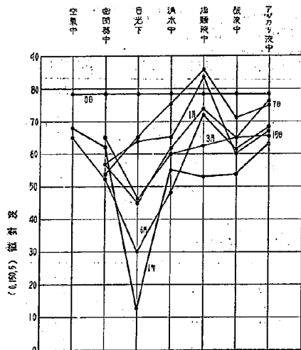
第 12 図 ストレート・アスファルト (150~200) 1.0°C 稠度変化 但し, (0mm, 150g, 5sec) の微針度
