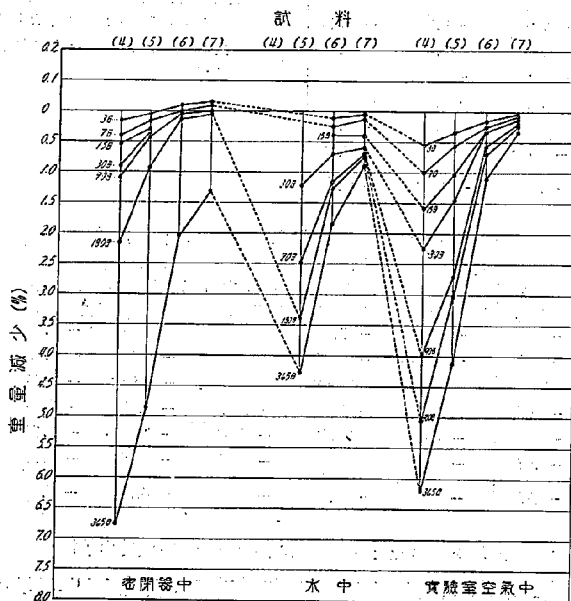
第4圖 鋪装用タール薄層重量變化 密閉器中, 水中, 實驗室空氣中
