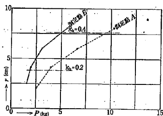
第 10 圖 振動中の壓力の變化の狀態 (方塊のない場合)
