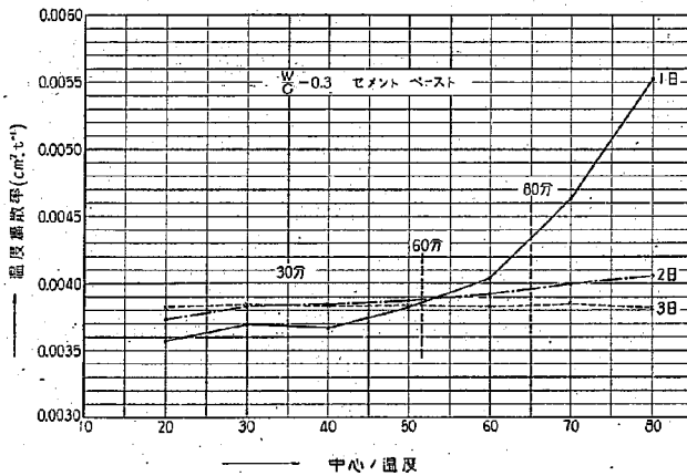
(c) 水中養生期 (高温恒温槽約 70^{\circ}\text{C} )
