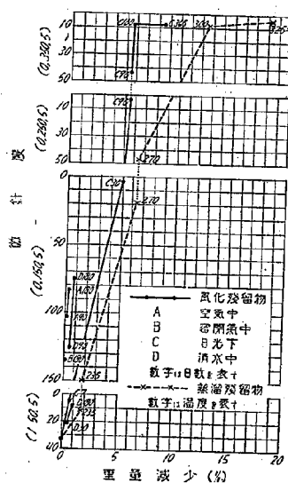
第 42 圖 タール(7)蒸溜残留物及各種風化残留物 1.0^{\circ}\text{C} 微針度變化と重量變化
