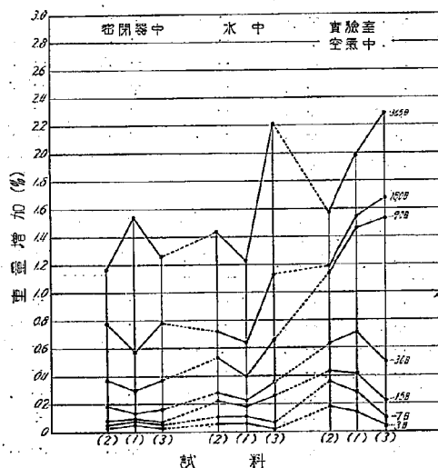
第 2 圖 アスファルト薄層重量變化 密閉器中、水中、實驗室空氣中
