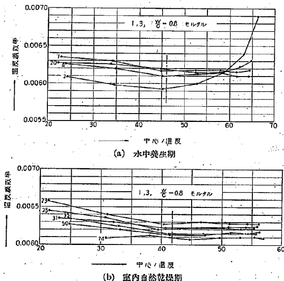
第 14 圖 1:3, w/c=0.8 モルタル温度擴散率と試料中心温度との關係
