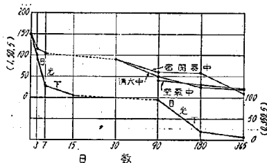
第24圖 加熱混合マカダム用タール(6)
