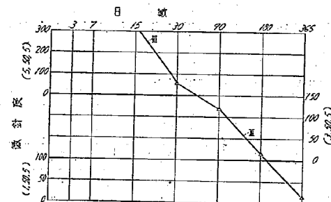
第 17 図 常温用タール (4) 25°C 微針度 (日光下試料)
