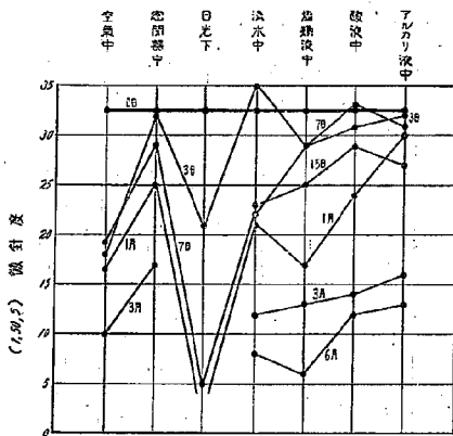
第 26 圖 加熱混合用タール (7) 1.0°C 稠度變化 但し、(1, 50, 5) 微針度
