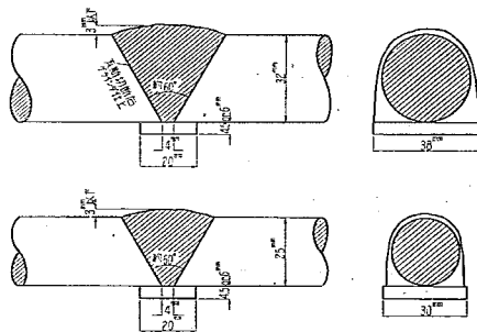
圖-37 底鈹附 V 形銲合熔接接手
