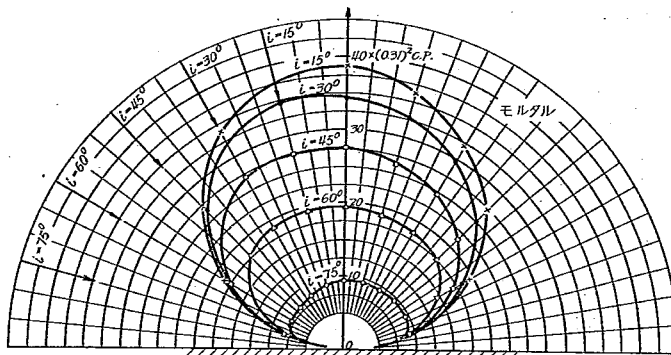
図-18 モルタル仕上コンクリートブロック反射光度分布
