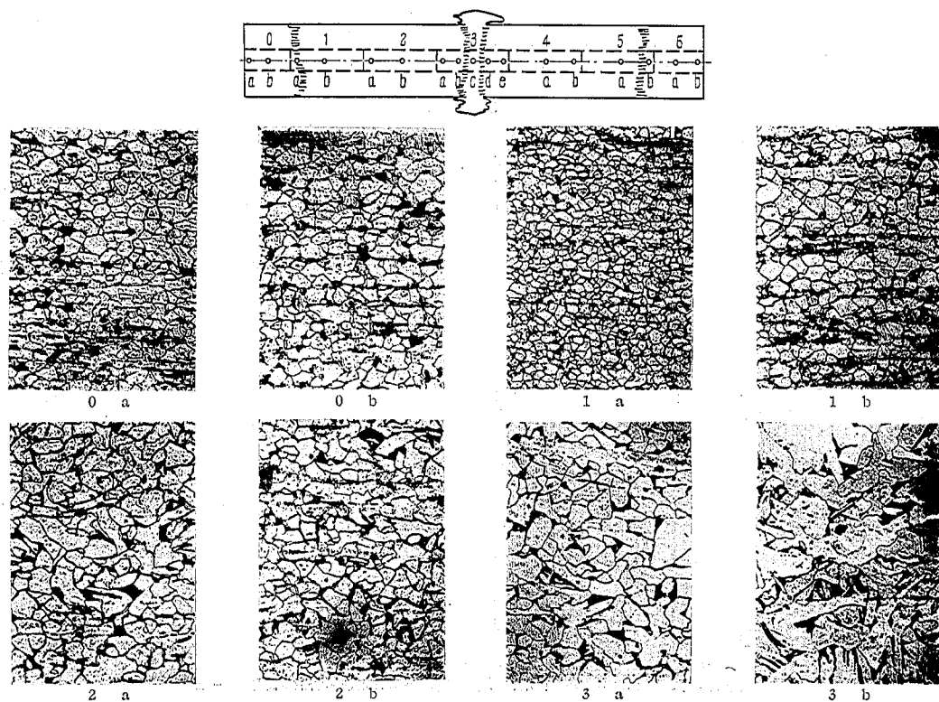
圖-4 丸鋼火花熔接試片鋼材組織寫眞 (4% Nital 原圖 \times 245 を \frac{1}{2} に縮寫)
