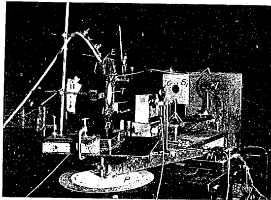
寫眞-1 光反射分布試験室內用裝置
