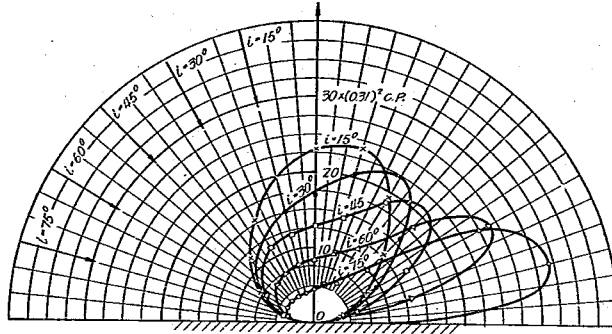
図-17 1:2 膠石コンクリート反射光度分布
