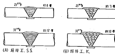
図-39 底鉋附 V 形銲合熔接 手試片ビードの盛り方
