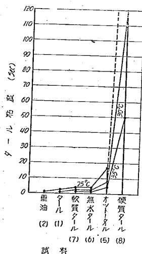
圖-3 タール粘度
