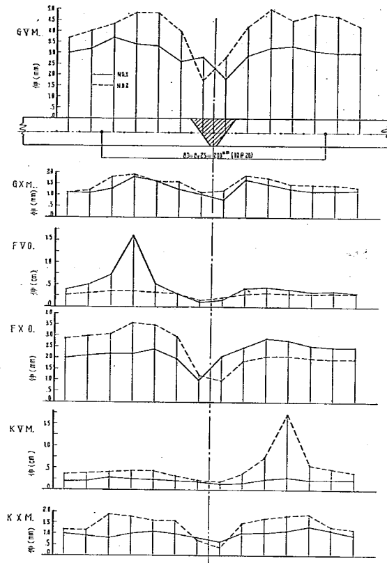
圖-29 熔接工 U による銲合熔接試片の延伸圖
