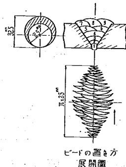
圖-17 熔接工 S の V 形銑合接手施工順序
