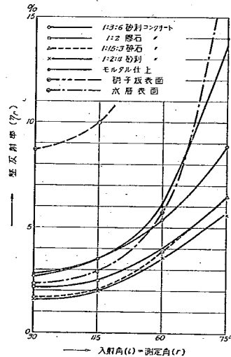
圖—47 路面の流水狀態に於ける整反射率( \eta_r )と反射角(入射角)との關係
