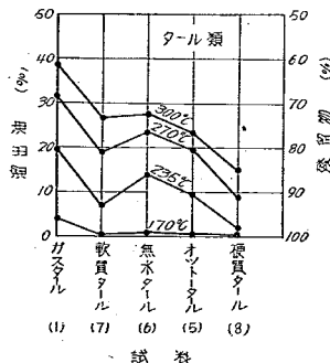
圖-5 B 蒸溜試験
