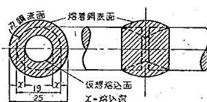
圖-7 I 形銑合熔接端面圖
