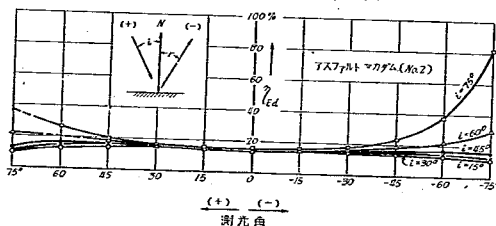
圖—41 同價擴散反射率 \eta_{Ed} 圖
