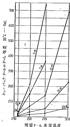
圖-23 残留タールの蒸溜 温度とカット・バック・タ ールのタール粘度(35°C)
