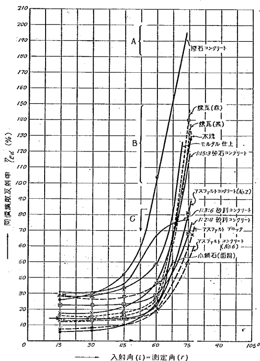
圖—45 測定方向、入射角と同値擴散反射率 \eta_{Ed} との関係
