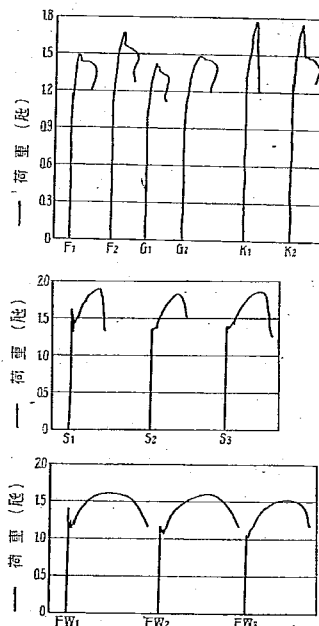
圖-13 熔着鋼引張試験荷重伸長曲線
