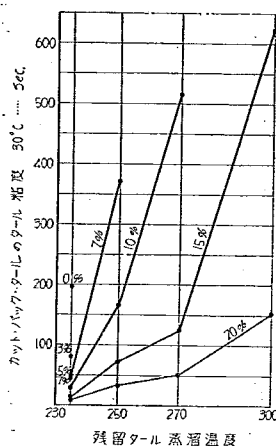
圖-22 残留タールの蒸 溜温度とカット・バック・ タールのタール粘度 (30°C)
