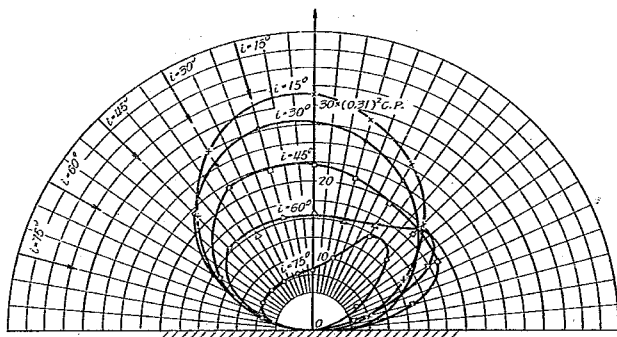
図-14 1:3:6 砂利コンクリート反射光度分布
