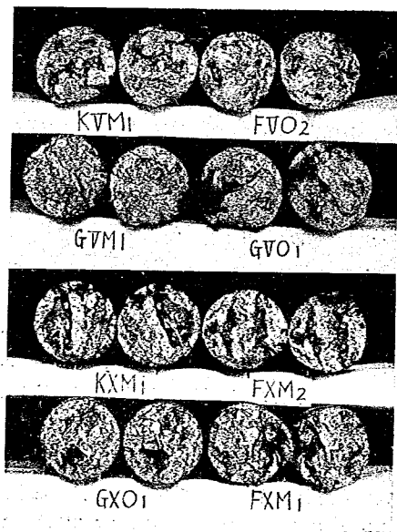
圖-28 同前の試片の切斷面
