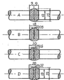
圖-6 I形銲合熔接試片 (三浦氏による)
