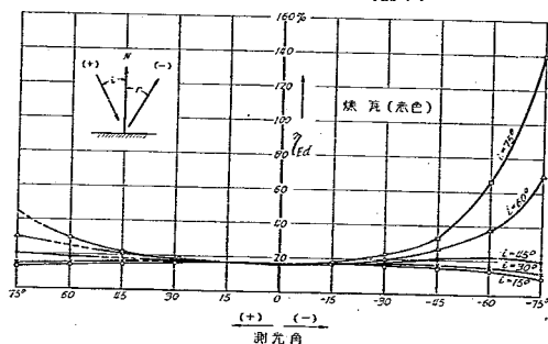
圖—42 同價擴散反射率 \eta_{Ed} 圖
