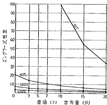
図-14 A 235°C 残留タールの カット・バック・タール比粘度
