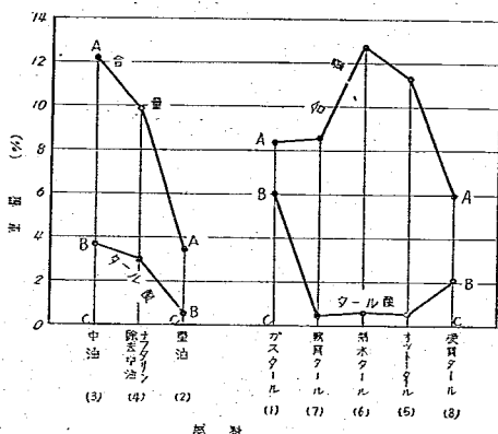
図-10 タール酸及ナフタリン 曲線 AA=ナフタリン+タール酸の含量 BB=タール酸 ABの距離はナフタリンを表す
