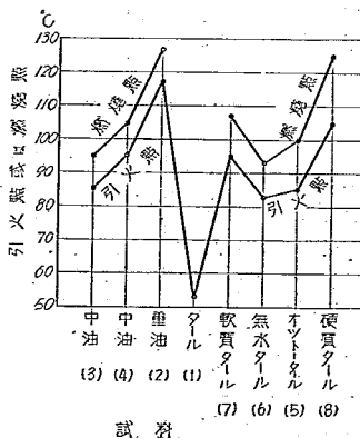
圖-4 引火點及燃焼點
