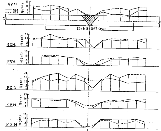
図-26 熔接工 S による銲合熔接試片の延伸図
