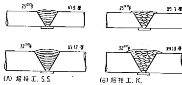
図-39 底鈹附 V 形銲合熔接 手試片ビードの盛り方
