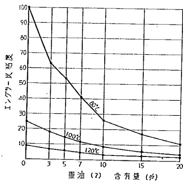
図-16 A 270°C 残留タールの カット・バック・タール比粘度
