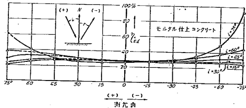
圖-39 同値擴散反射率 \eta_{Ed} 圖
