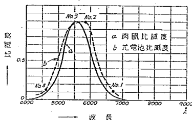
圖-10 使用堰層光電池の比感度
