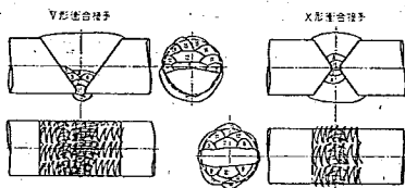
圖-19 熔接工 U の銜合接手施工順序
