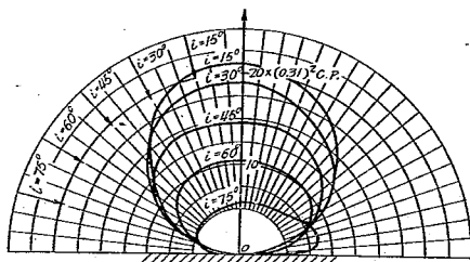
圖-19 アスファルトコンクリート (No. 2) 反射光度分布
