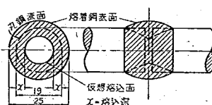
圖-7 I 形銑合熔接端面圖
