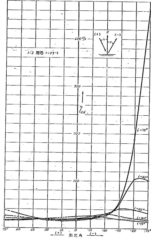
圖-38 同値擴散反射率 \eta_{Ed} 圖
