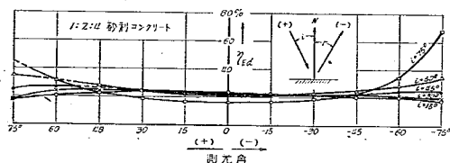
圖—36 同價擴散反射率 \eta_{Ed} 圖
