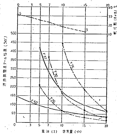
図-15 B 250°C 残留タールの カット・バック・タール稠度
