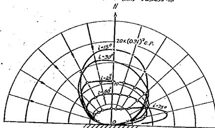
圖-22 煉瓦(黒) 光度分布
