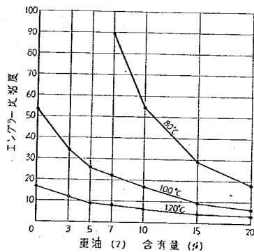
図-17 A 300°C 残留タールの カット・バック・タール比粘度
