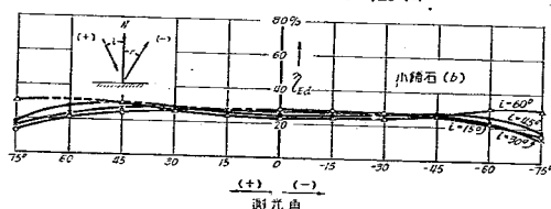
圖—42 同價擴散反射率 \eta_{Ed} 圖
