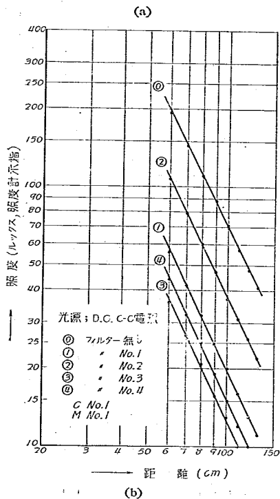
図-9 遮光フィルター使用せし場合の照度計指示性能を示す
