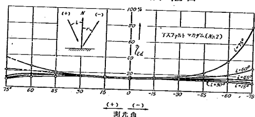
圖—41 同價擴散反射率 \eta_{Ed} 圖
