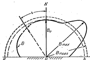
圖-3 反射擴散能説明圖
