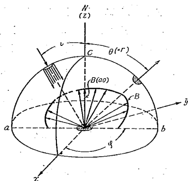
圖-2 反射光線分布測定方向を示す
