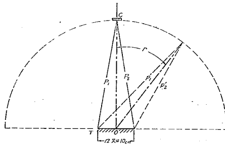
寫真-1 光反射分布試験室內用裝置
