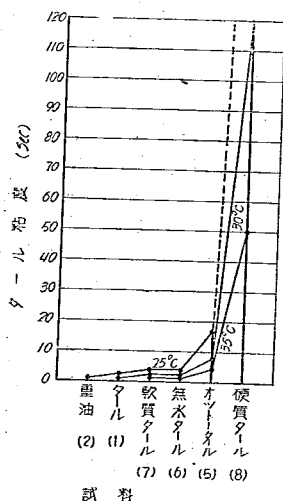
圖-3 タール粘度
