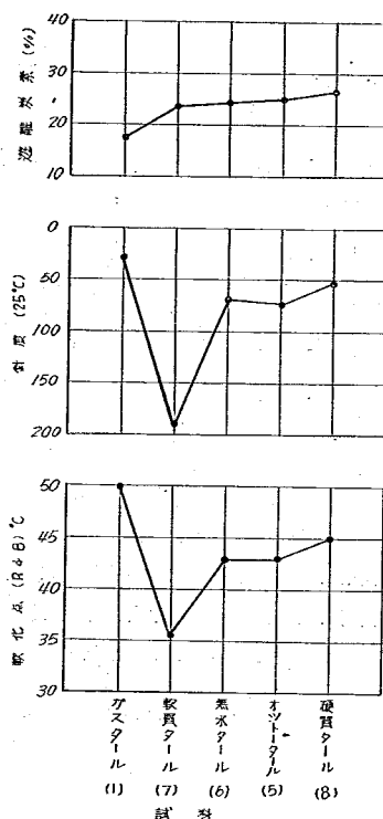
圖-9 300°C 蒸溜残留物性質
