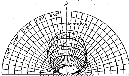
圖-16 1:1.5:3 碎石コンクリート反射光度分布
