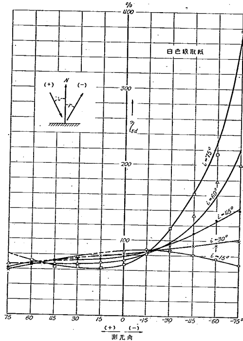
圖-43 同値擴散反射率 \eta_{Ed} 圖
