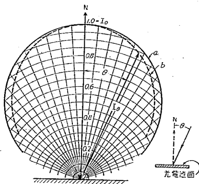
圖-11 受光面に対する投射光方向と光電池指向との關係
