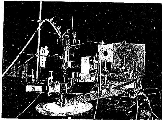
寫真-1 光反射分布試験室內用裝置
