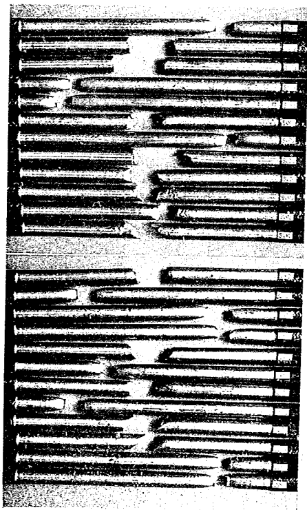
圖-30 熔接工 K による試片の切断状況 S : S 社製 E 印電極棒使用 L : L 社製 FW 電極棒使用
