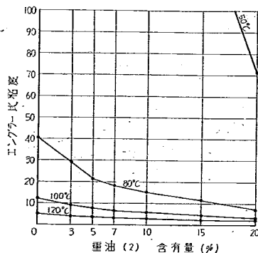
図-15 A 250°C 残留タールの カット・バック・タール比粘度
