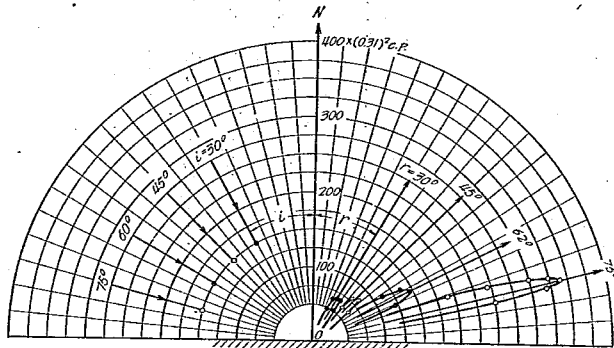
圖—28 モルタル仕上コンクリートの流水状態に於ける整反射
