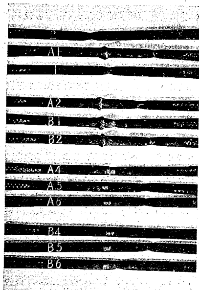
圖-3 丸鋼火花熔接試片 縦断面マクロ寫眞
