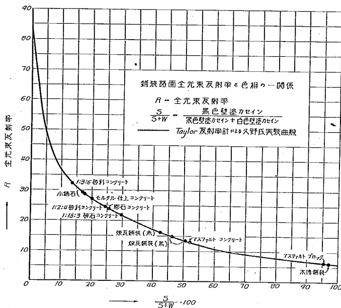
圖一46 舗装面全光束反射率と色相との一關係
