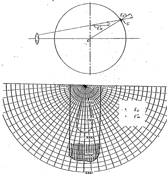
圖 13 試料面上照度分布圖
