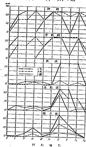
圖-3 折曲試驗成績
