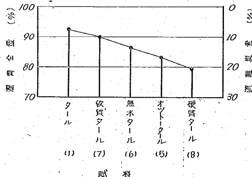
図-11 瀝青全量及游離炭素 (+灰分)
