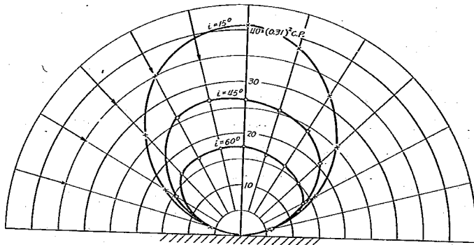
圖—25 小 鋪 石 反 射 光 度 分 布
