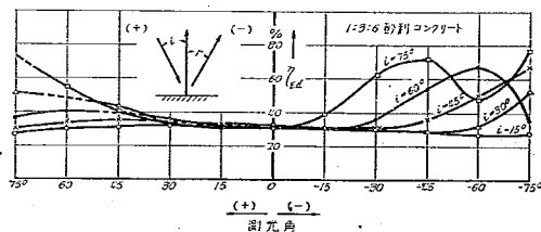
圖—37 同價擴散反射率 \eta_{Ed} 圖
