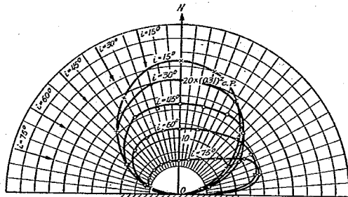
圖-23 煉瓦(赤) 反射光度分布
