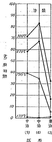
圖-5 A 蒸溜試験
