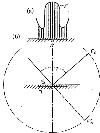
圖-5 整反射率測定に於ける光路を示す
