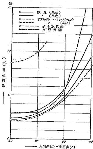
圖一47 路面の流水狀態に於ける整反射率( \eta_r )と反射角(入射角)との關係
