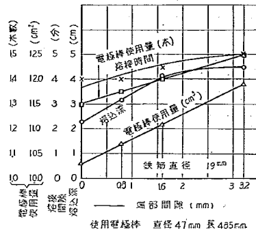
圖-8 端部間隙と熔込深、熔接時間、電極棒消費量。
