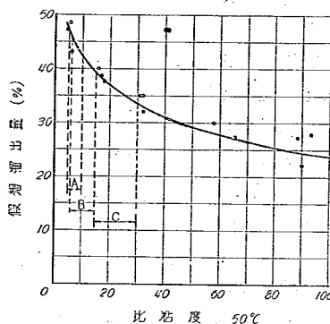
圖-7 比粘度( 50^{\circ}\text{C} )と假想溜出量との關係
