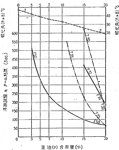
図-17 B 300°C 残留タールの カット・バック・タール稠度
