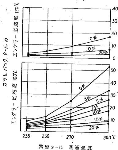
図-20 残留タール蒸溜温度と カット・バック・タールのエングレー比粘度 (100°C 及 120°C)
