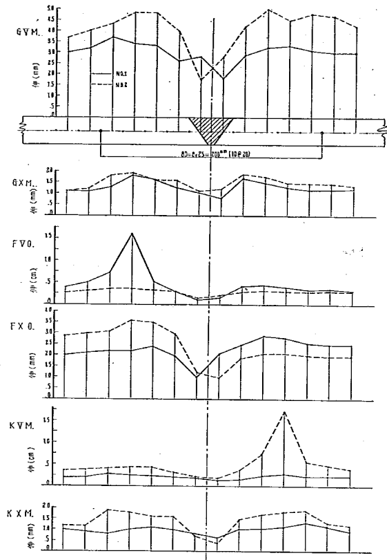
圖-29 熔接工 U による銜合熔接試片の延伸圖
