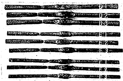
圖-36 V形銲合熔接試片切斷狀況 (庄川用水)
