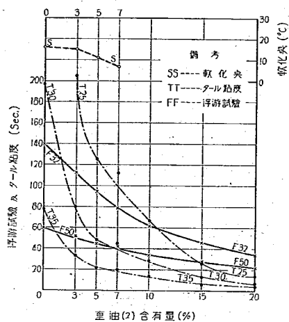
図-14 B 235°C 残留タールの カット・バック・タール稠度
