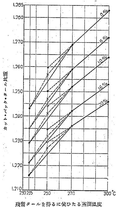
圖-13 カット・バック・タールの比重 と残留タールの蒸溜温度
