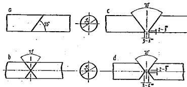
圖-12 熔着鋼試験片寸法
