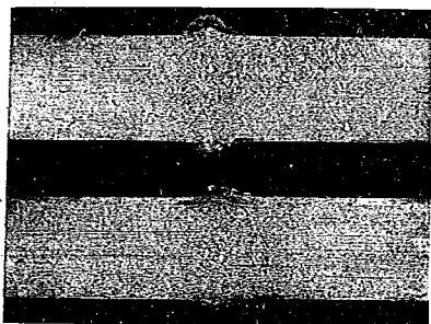
圖-3 丸鋼火花熔接試片 縦断面マクロ寫眞
