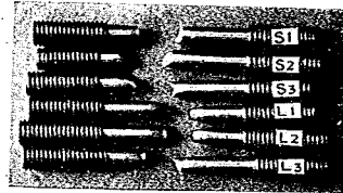
圖-14 E 印及 FW. の切斷狀況 S: S 社の E 印 L: L 社の FW.
