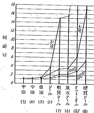
圖-2 エンゲラー比粘度
