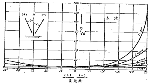
圖-44 同値擴散反射率 \eta_{Ed} 圖
