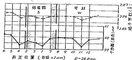
圖-9 V 形熔合熔接部断面に於ける 燒鈍後の格子常数分布圖
