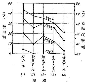
圖-6 タール類の 300°C 蒸溜残留物を 60°C としたる場合の假想溜出量 (%)
