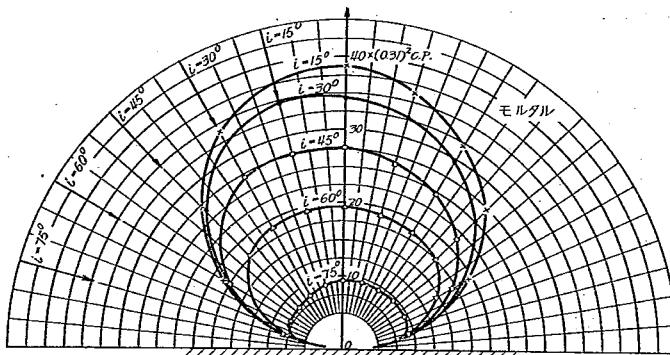
圖一八 モルタル仕上コンクリートブロック反射光度分布
