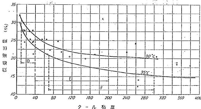
圖-8 タール粘度( 30^{\circ}\text{C} 及 35^{\circ}\text{C} )と假想溜出量との關係
