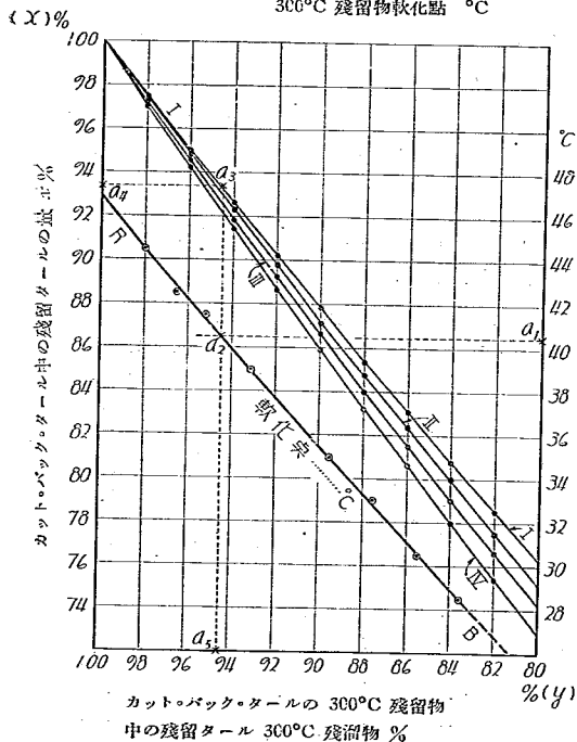
図-18 カット・バック・タールの配合と 300℃ 残留物軟化点 °C
