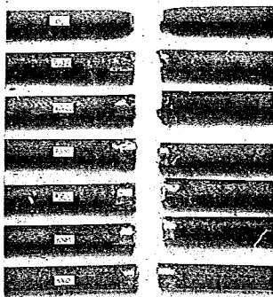
圖-24 同前試験片の切断面 (V 形溶接接手)
