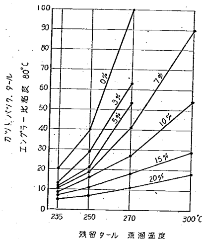
図-19 残留タール蒸溜温度と カット・バック・タールのエングレー比粘度 (80°C)
