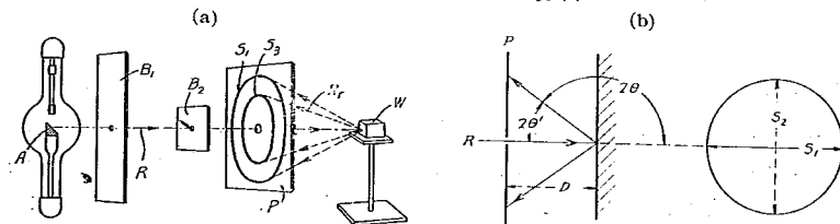
圖-3 X 線反射法説明圖
