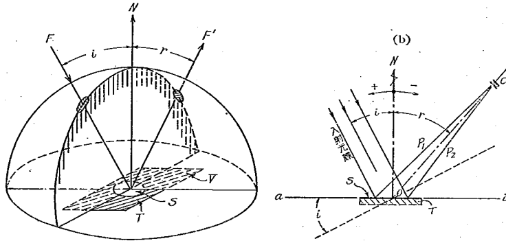
圖-4 反射光分布試験に於ける入射角と測定方向の關係を示す (a)
