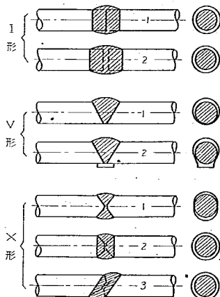
圖-5 丸鋼の銲合熔接接合の種類
