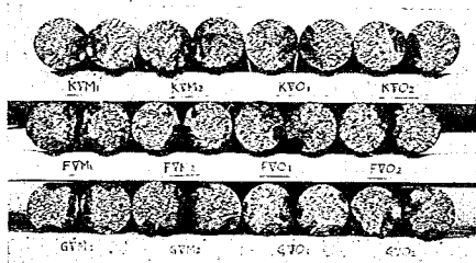
圖-25 同前試験片の切断面 (X 形溶接接手)
