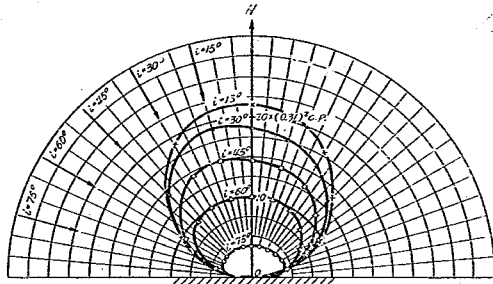
圖-15 1:2:4 砂利コンクリート反射光度分布
