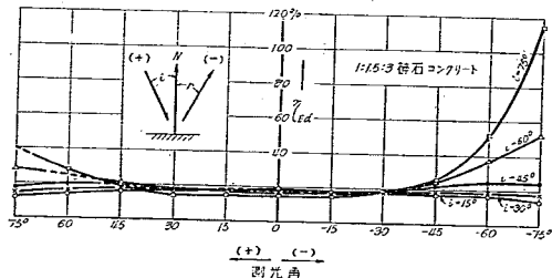
圖—37 同價擴散反射率 \eta_{Ed} 圖
