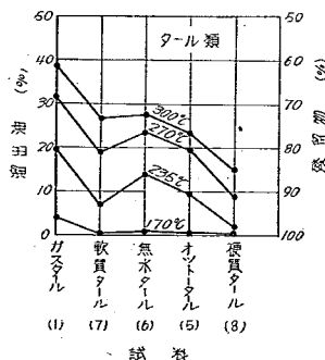
圖-5 B 蒸溜試験
