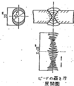
圖-18 熔接工 S の X 形銲合接手施工順序
