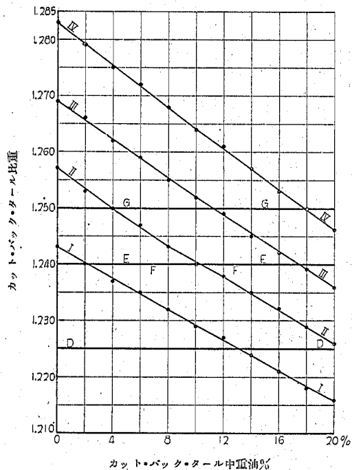
圖-12 カット・バック・タールの比重と カット・バック 油の量との關係
