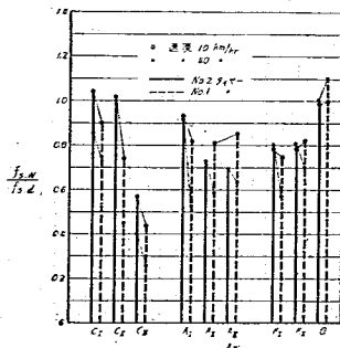
図-49 各種路面に於ける f_{s-w}/f_{s-d} 比率
