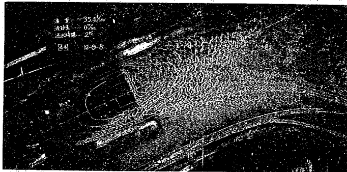
圖—112 第 1 案に依る阻柱無き場合の洗掘状態、流出状態 圖—59 (b)
