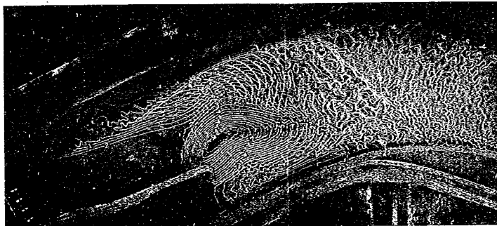
圖—90 流れが右岸寄りに集中する場合の洗掘状態、流出状態 (a), 水叩水平
