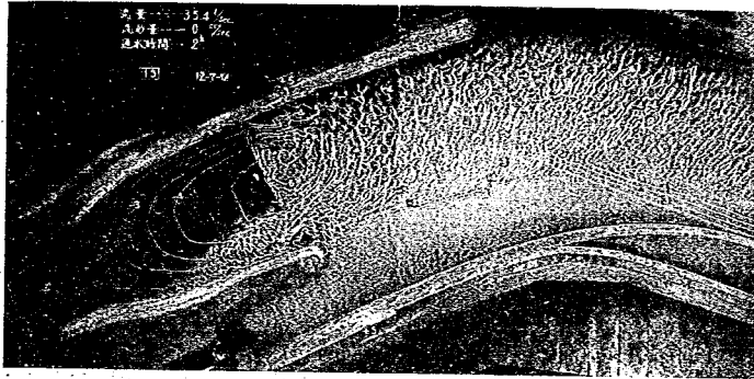
図一110 左岸法先及び導流堤先端法先に沈床を設置せる場合の洗掘状態、 流出状態 図一39 (b)
