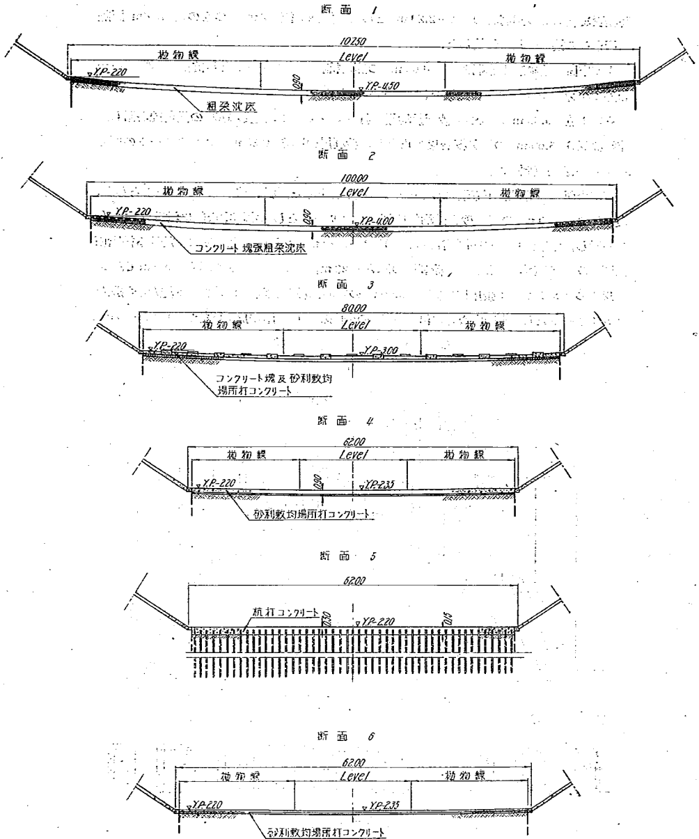
圖—37 水門上下流横断面圖
