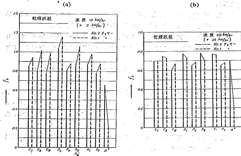
圖—47 タイヤー種別と f_b 係数との関係(乾燥状態)
