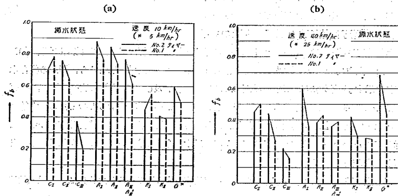
圖—48 タイヤー種別と f_b 係数との関係(撤水状態)
