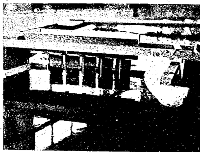
圖-48 給砂装置
