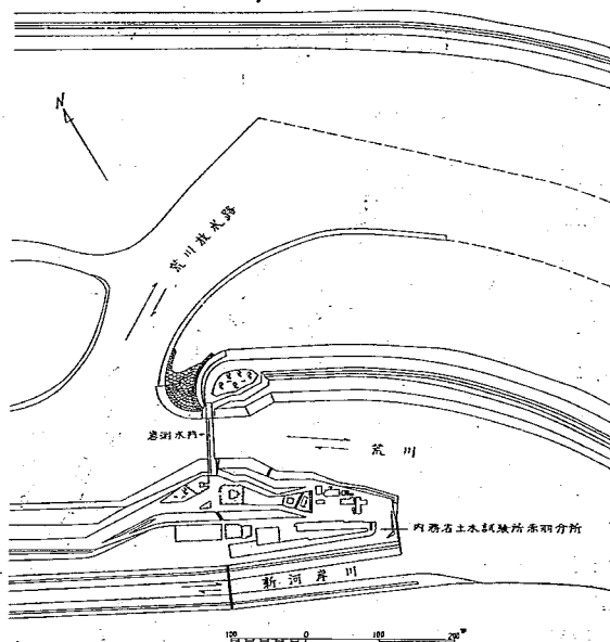
圖一 岩淵水門附近平面圖
