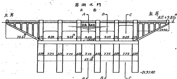
圖-3 岩淵水門正面及側面圖
