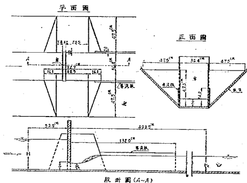
圖—64 岩淵水門 2 徑間模型
