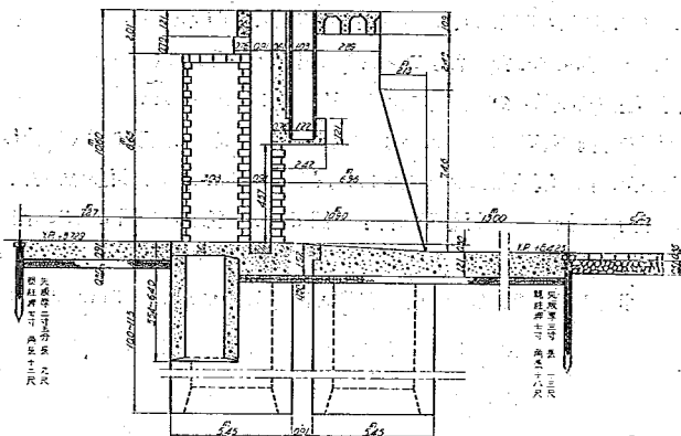
圖 一 27 翼 壁
