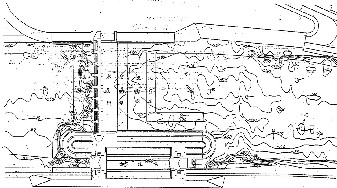
關宿水門及閘門上下流深淺圖
