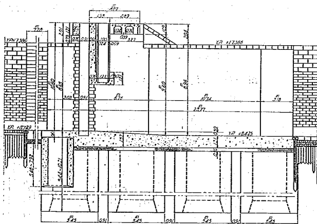
圖 一 27 翼 壁
