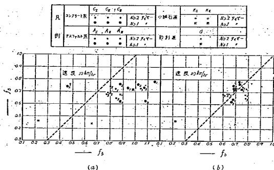
圖-53 撒水路面の f_b \sim f_s 係數關係
