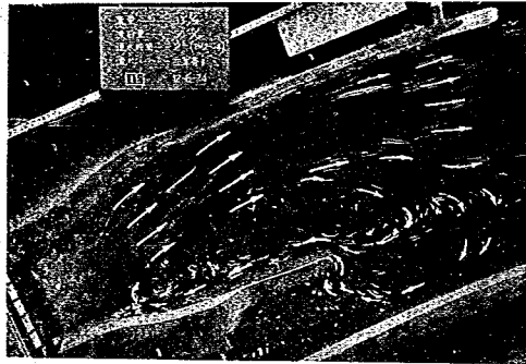
圖—95 流れが右岸寄りに集中する場合の流向
