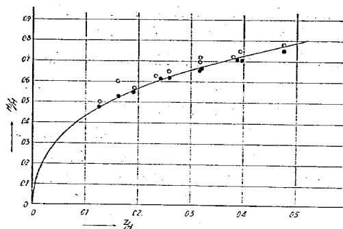
図-66 岩淵水門1 徑間模型に於ける射流及び潜流の限界曲線 (導流板なし)
