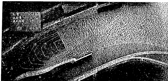
圖—98 導流堤を 50 m 延長せる場合の沈掘状態，流出状態 圖—59 (b)
