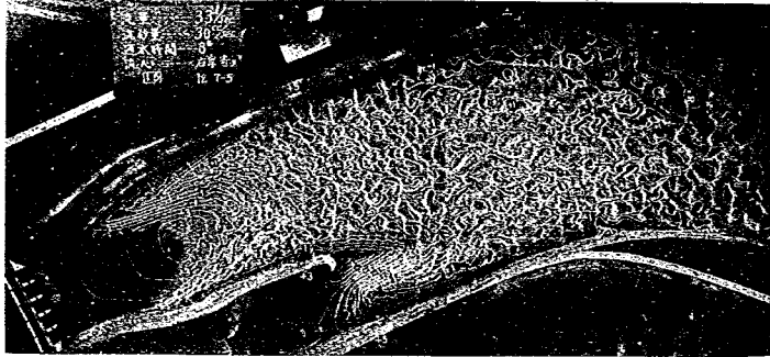
圖—121 流砂量 30 cc/sec に於る洗掘状態 (8 時間後) 流出状態 圖—59 (a)
