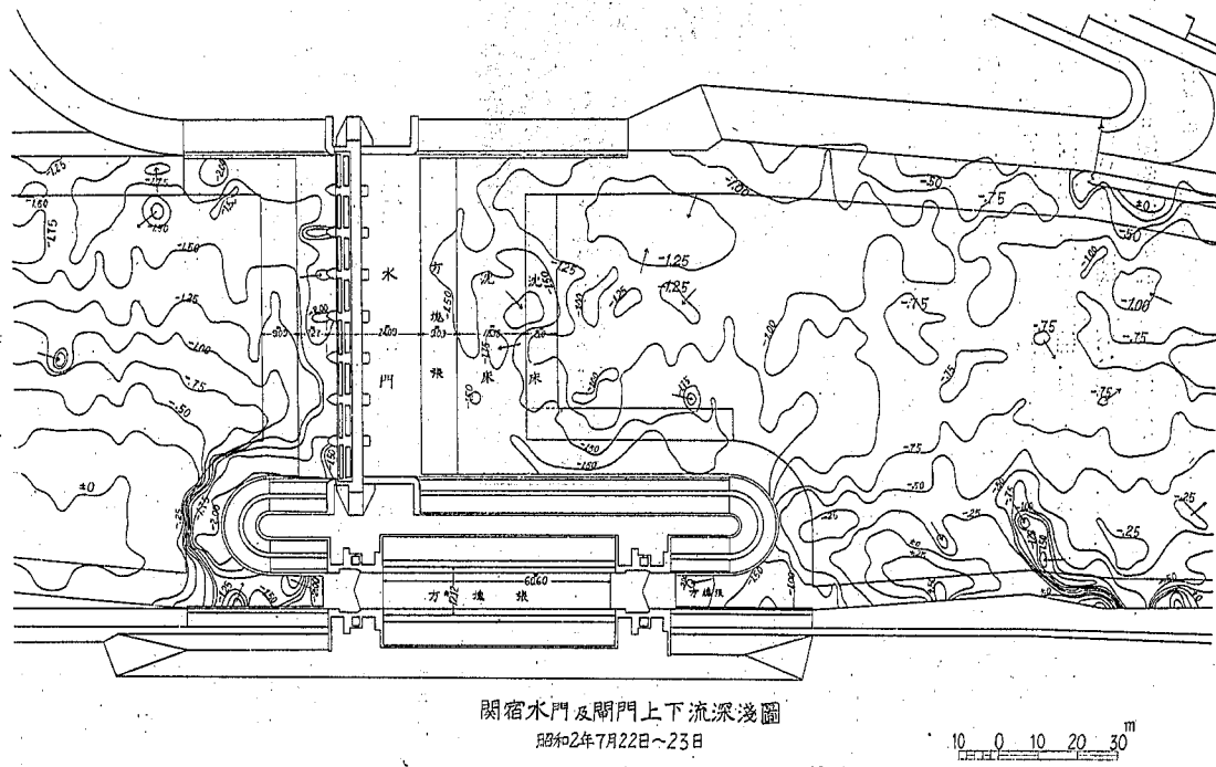
圖 一 29 昭和2年7月に於る關宿水門上下流洗掘堆積狀態
