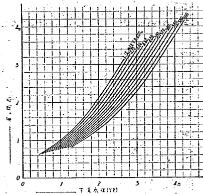
圖—69 射流を生ぜしめざる扉の開高
