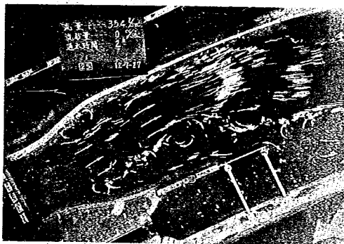
圖一103 導流堤 25 m 短縮, 導流杭 50 m 設置の場合に於ける洗掘状態, 流出状態 圖一59 (b)
