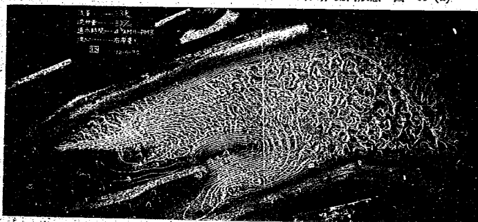
圖—122 流砂量 30 cc/sec に於る洗掘状態 (4 時間後), 流出状態 圖—59 (a)
