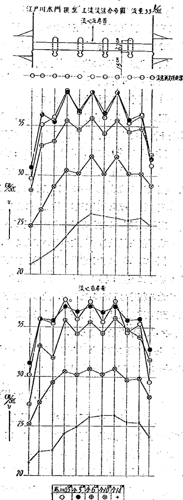
圖—129 水門上流流速分布
