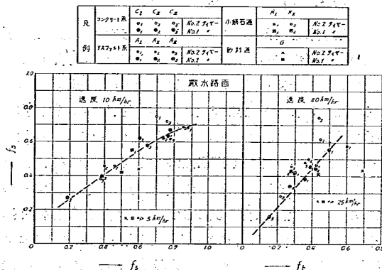
圖-53 撒水路面の f_b \sim f_s 係數關係
