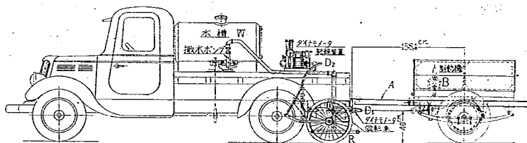
(a) 縦滑り試験の場合 路面抵抗測定車
