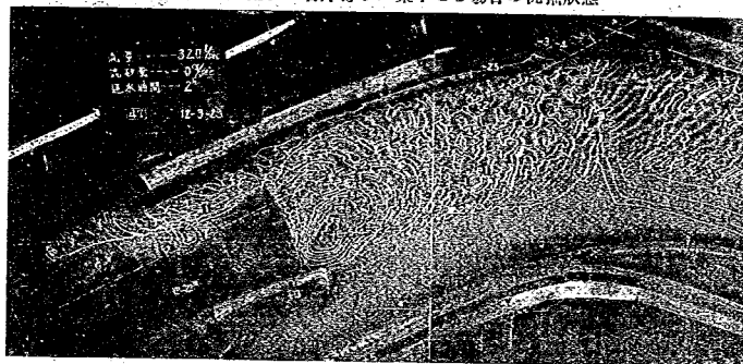
圖—86 流れが左岸寄りに集中せる場合の洗掘状態
