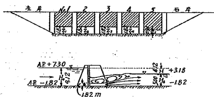
圖 — 7 開高及最高水位
