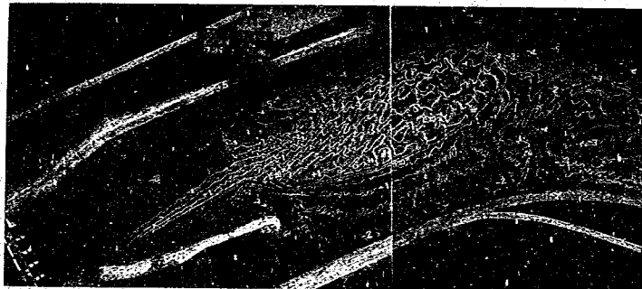
圖—115 流砂量 29.6 cc/sec に於る洗掘状態, 流出状態 圖—59 (a)
