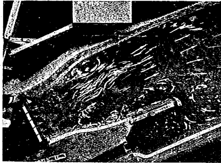
圖—100 導流堤を 25 m 短縮堤上を越流せしめざる場合の流向、流出状態 圖—59 (b)
