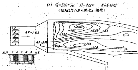
圖—43 岩淵水門模型實驗に於る下流洗掘狀態
