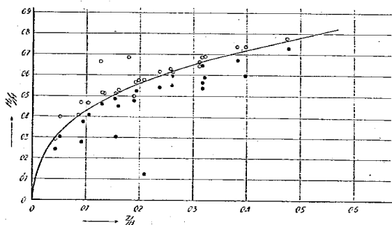
図-66 岩淵水門1 徑間模型に於ける射流及び潜流の限界曲線 (導流板なし)
