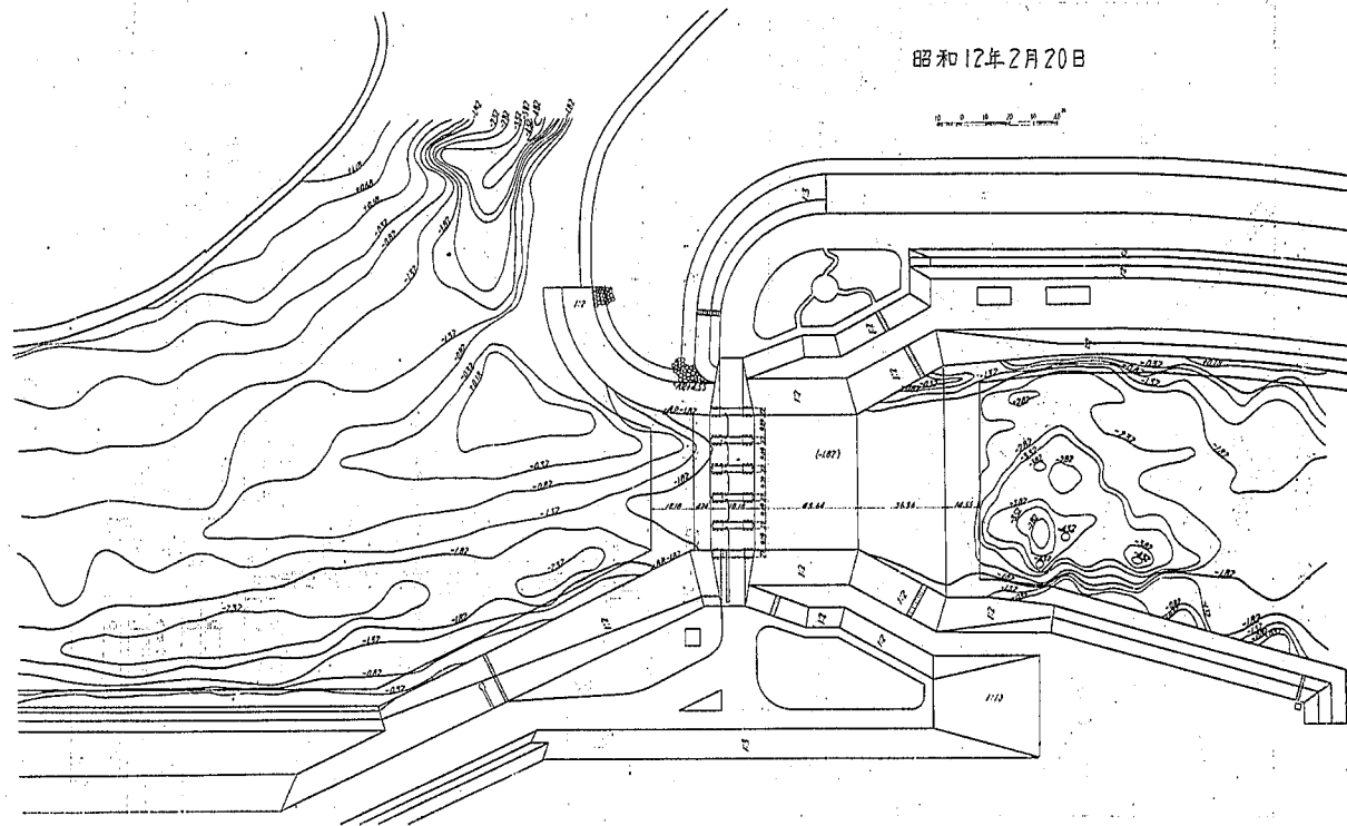
圖-20 岩淵水門上下流河底現狀
