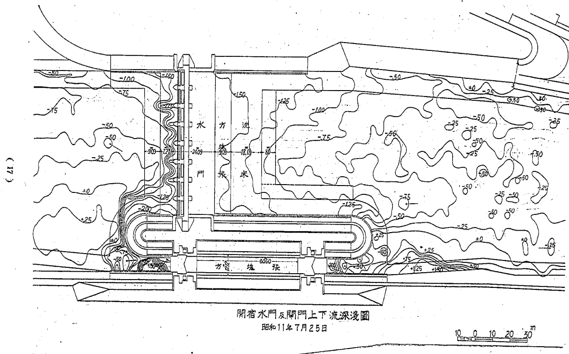
圖 — 30 昭和 11 年 7 月に於ける關宿水門上下流洗掘堆積狀態
