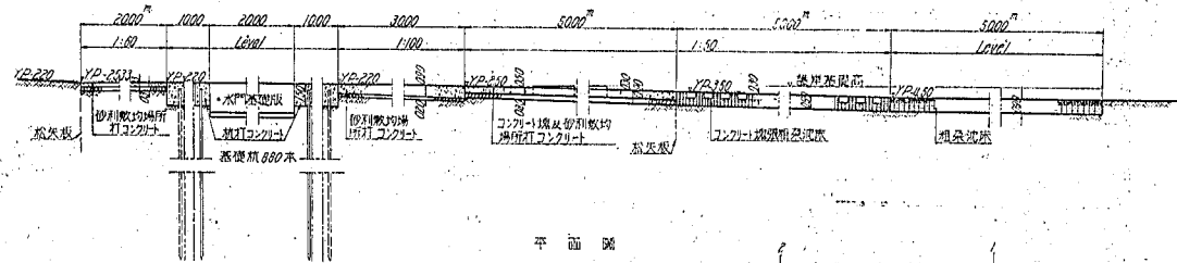
圖一 36 江戸川水門床固及沈床
