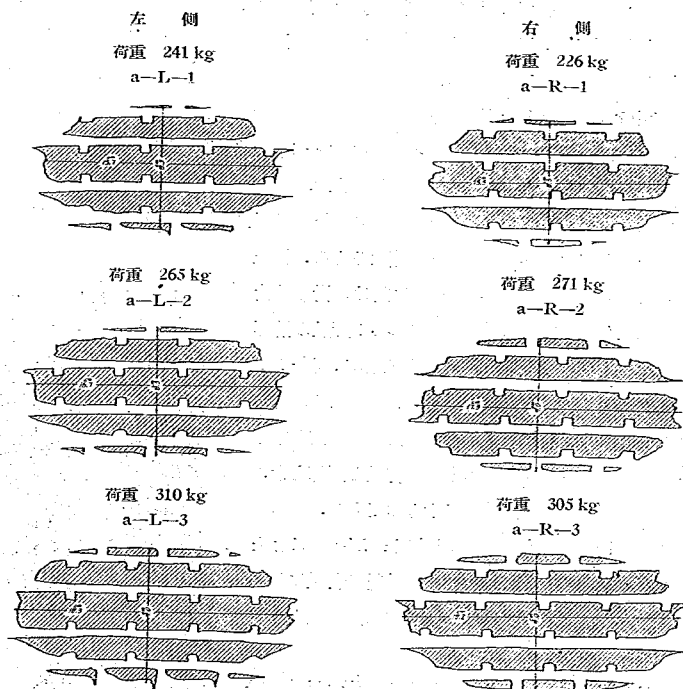
圖-6 (a) タイヤー No. 2 接觸図形 空氣壓力 29 lbs/□"
