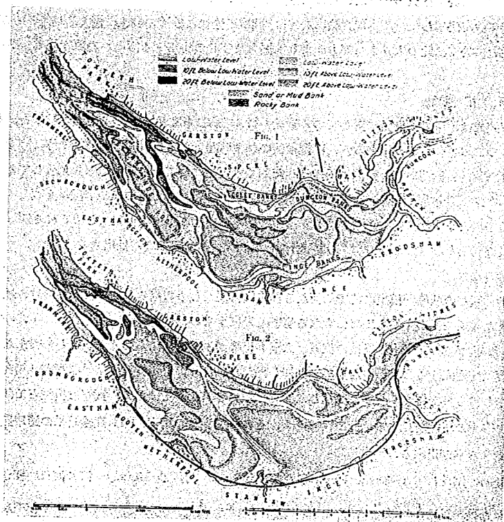
圖—42 Mersey 河口河底 (上) と模型に於ける河底 (下)
