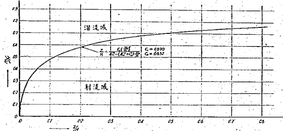
圖-62 江戸川水門模型に於る射流及び潜流の限界曲線
