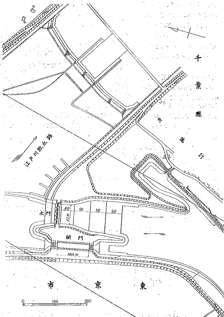
圖一 33 江戸川水門及開門附近平面圖（兩鐵線内の部分を模倣に取入れた）
