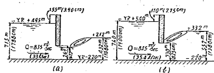
圖—59 江戸川水門上下流水位及び扉の開高 ( )内は模型に於ける量を示す
