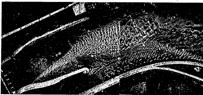
圖—115 流砂量 29.6 cc/sec に於る洗掘状態, 流出状態 圖—59 (a)
