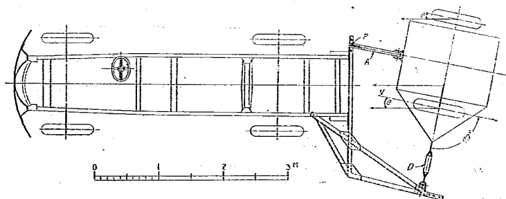
(c) 横滑り試験の場合 (平面圖)
