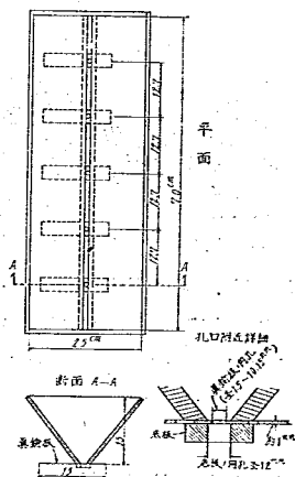
圖-47 給砂装置
