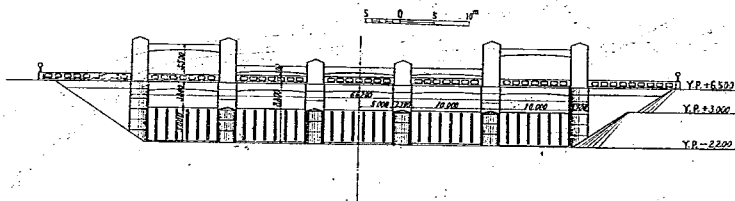
圖—34 江戸川水門正面圖 正面圖
