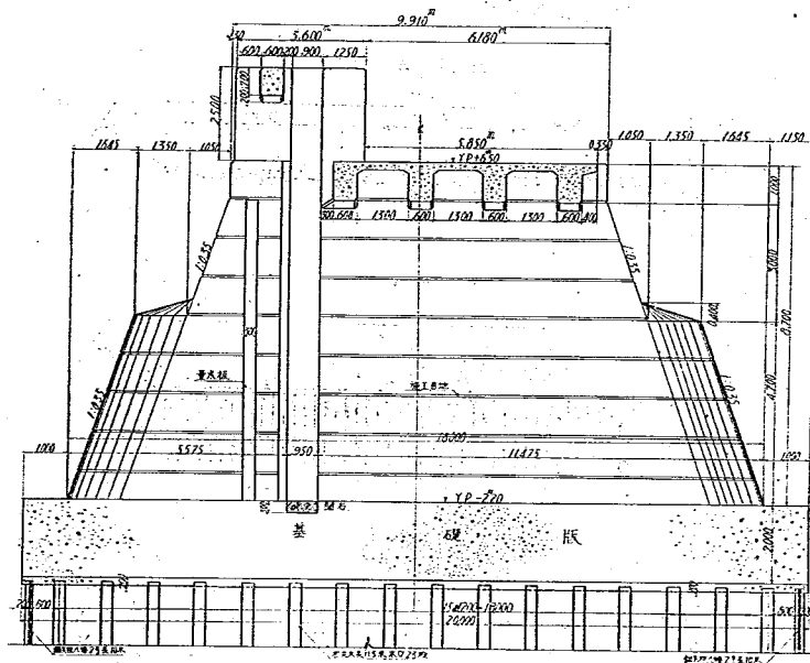
図-38 堰 柱 側 面 圖
