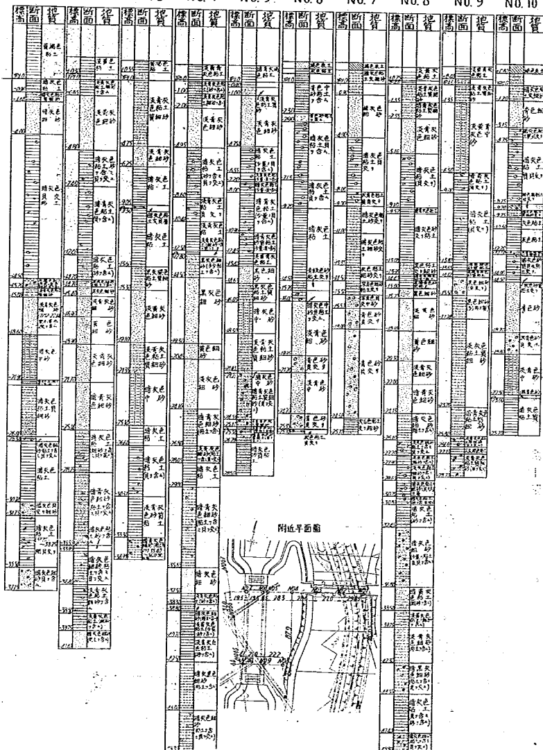
圖一 35 江戸川水門及開門地質圖
