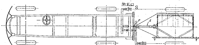
(b) 同上平面圖
