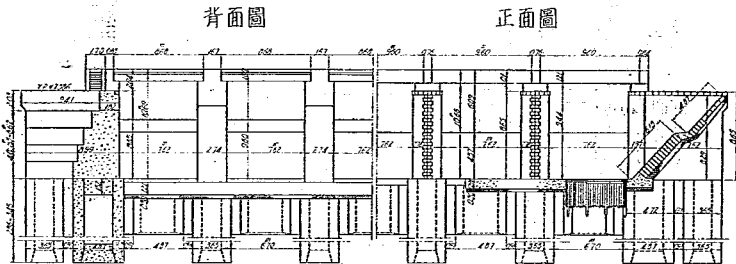
圖-25 關宿水門正面圖及背面圖
