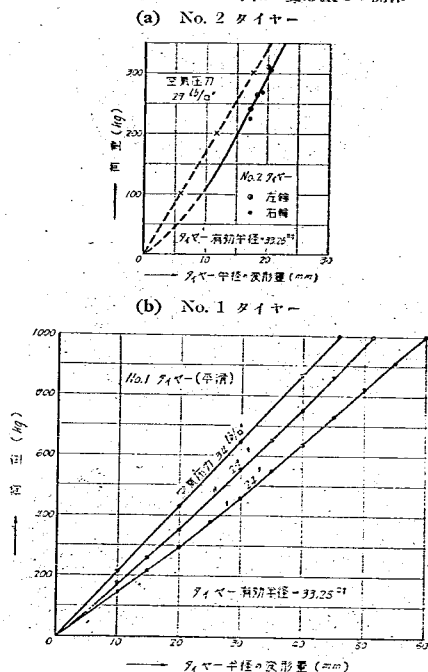
圖-8 荷重とタイヤ半径の變形量との関係
