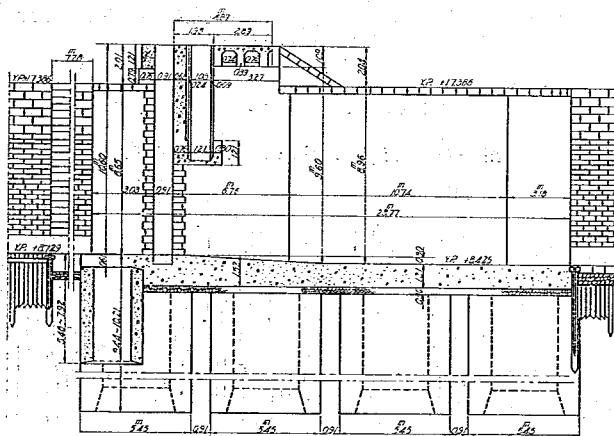
圖-27 翼 壁
