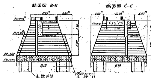
圖-5 岩淵水門堰柱
