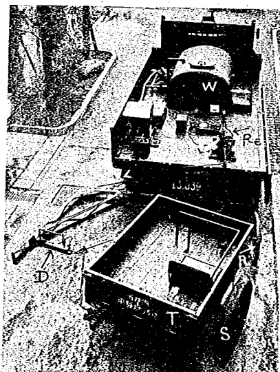
寫眞-1 (b) 横滑り試験に於ける試験装置の裝備
