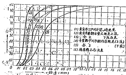
圖—41 江戸川砂及實驗用小名濱砂篩分曲線
