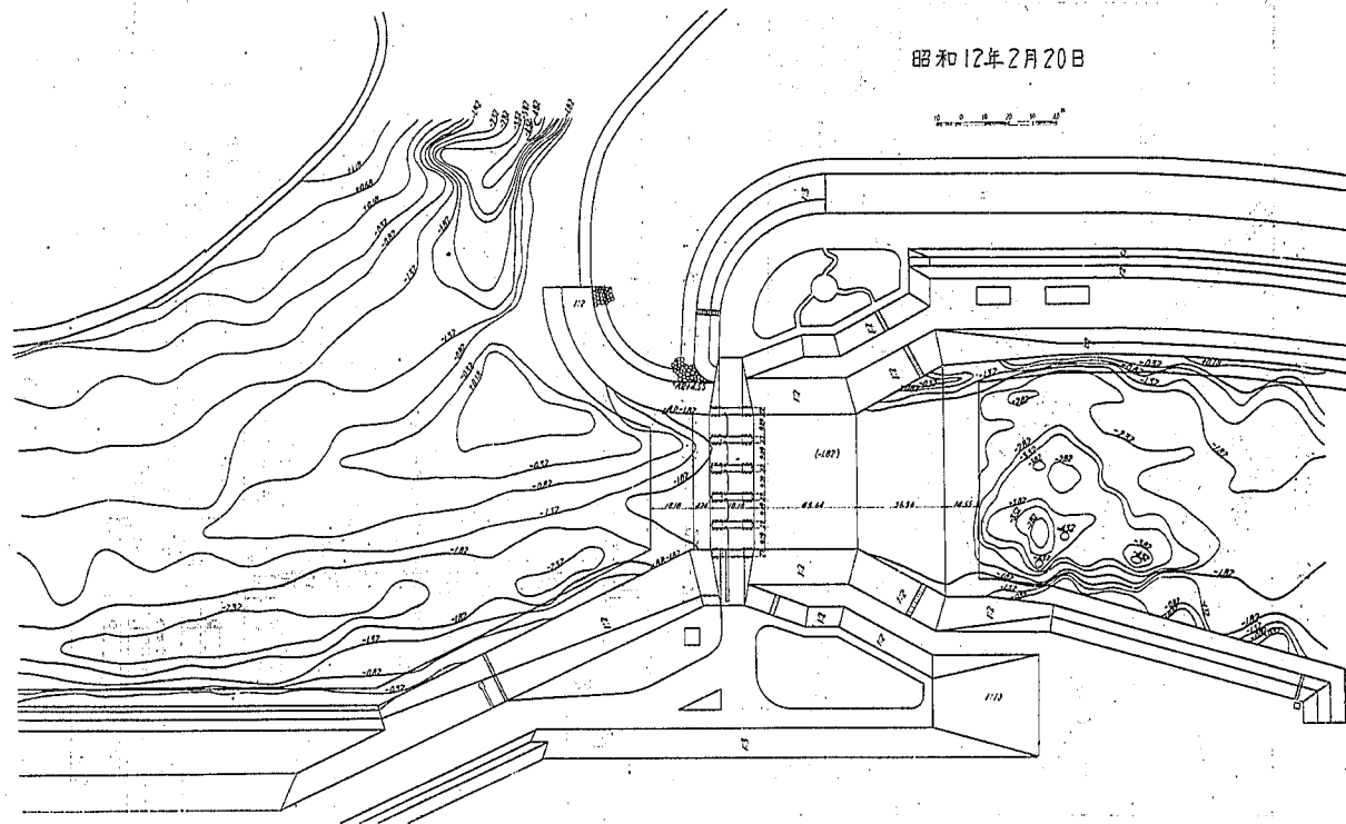
圖一20 岩淵水門上下流河底現狀
