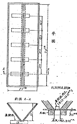
圖-47 給砂裝置
