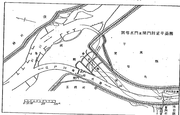
圖—22 關宿水門及開門附近平面圖
