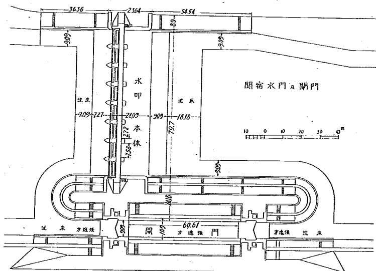
圖—23 關宿水門及開門平面圖
