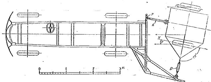
(c) 横滑り試験の場合 (平面圖)
