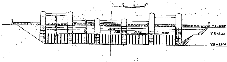
圖—34 江戸川水門正面圖 正面圖
