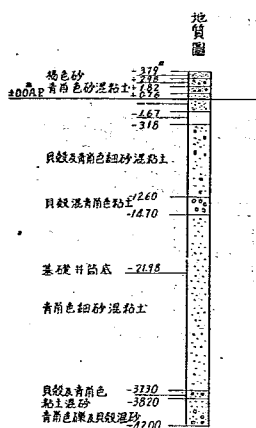
圖-4 岩淵水門地質圖
