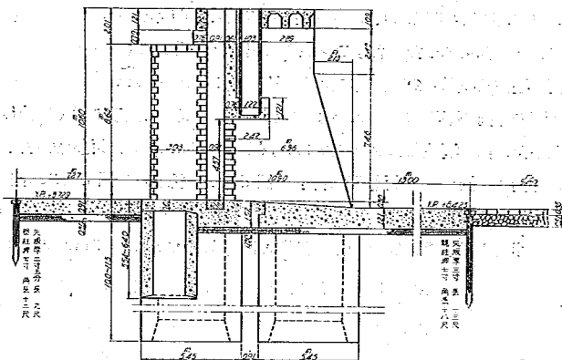
圖-27 翼 壁
