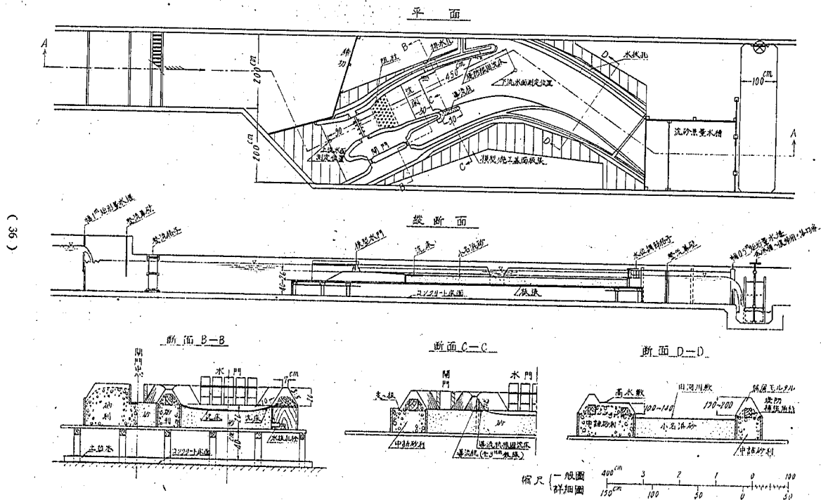
圖一 44 模 型 平 面、縱 斷 面 及 び 横 斷 面 圖
