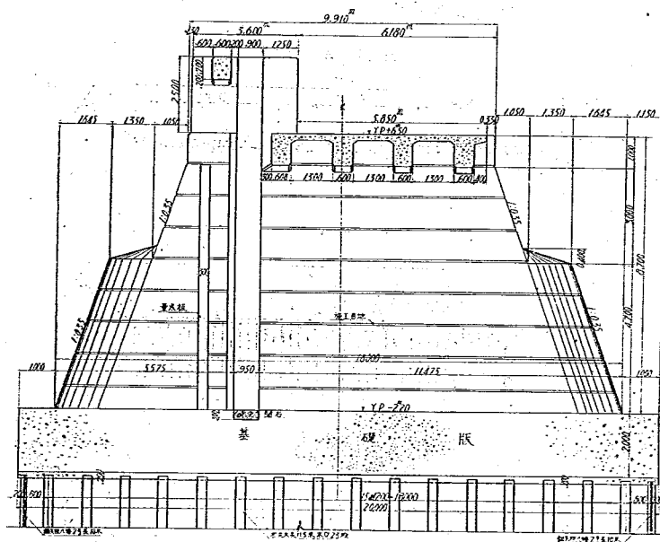
圖一 38 堰 柱 側面圖
