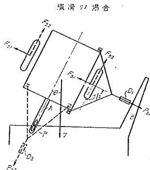
圖一5 摩擦抵抗算定用圖
