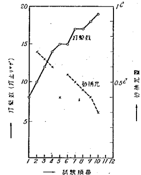
圖-7 試験順序と打止り迄の打撃回数
